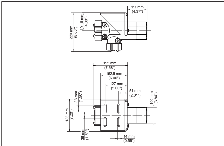
Fig. 25: POINTRAC 31 zonder detectorbuis, 46 mm (1,8 in) - met meegeleverde montagetoebehoren
