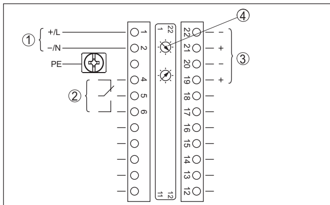
Fig. 12: Elektronica- en aansluitruimte (Ex-d) bij instrumenten met intrinsiekveilige stroomuitgang
