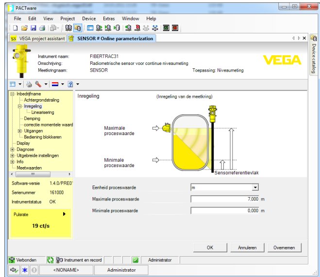
Fig. 23: Voorbeeld van een DTM-aanzicht
