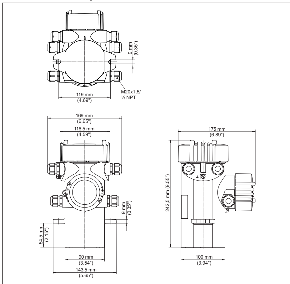
Fig. 30: Aluminium behuizing resp. rvs-behuizing (fijnnetwerk)
