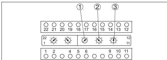
Fig. 15: Adreskeuzeschakelaar
