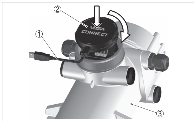
Fig. 18: Aansluiting van de PC via interface-adapter direct op de sensor
