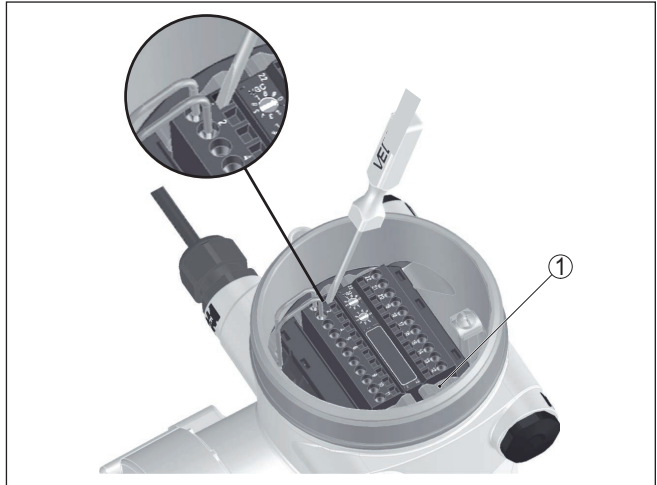
Fig. 10: Aansluitstappen 4 en 5
