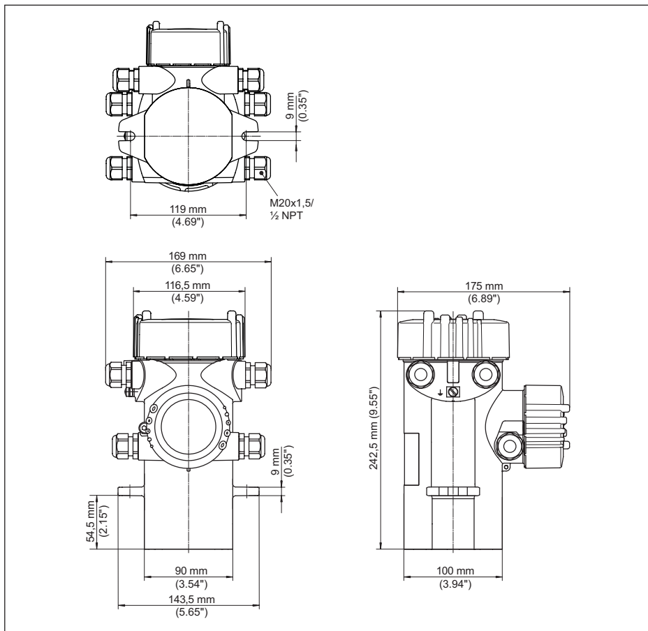
Fig. 25: Aluminium behuizing resp. rvs-behuizing (fijnnetwerk)
