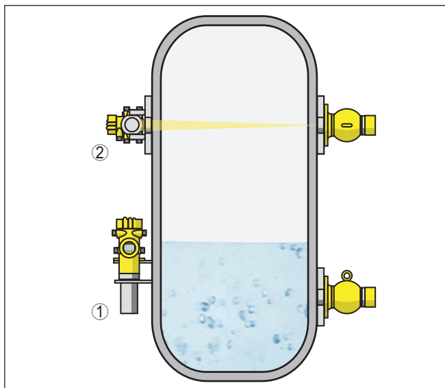
Fig. 4: Montagepositie - niveaudetectie - uitvoering met detectorbuis
