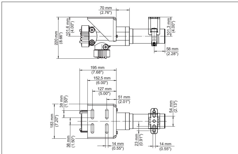
Fig. 27: POINTRAC 31 met detectorbuis, 152 mm of 304 mm (6 in/12 in) - met meegeleverde montage toebehoren
