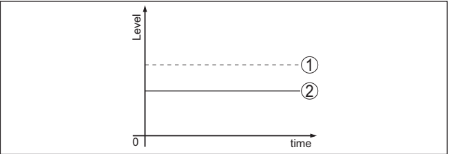
Abb. 25: Die gestrichelte Linie 1 zeigt den tatsächlichen Füllstand, die durchgezogene Linie 2 zeigt den vom Sensor angezeigten Füllstand
