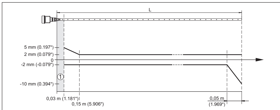
Abb. 27: Messabweichung VEGAFLEX 81 in Koaxialausführung in Medium Wasser
