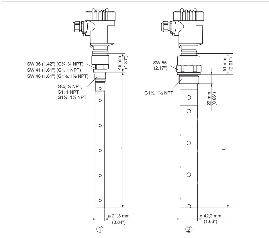
Abb. 36: VEGAFLEX 81, Gewindeausführung
