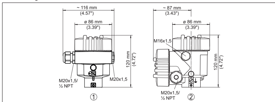
Abb. 32: Gehäuseausführungen in Schutzart IP66/IP68 (0,2 bar), (mit eingebautem Anzeige- und Bedienmodul vergrößert sich die Gehäusehöhe um 9 mm/0.35 in)
