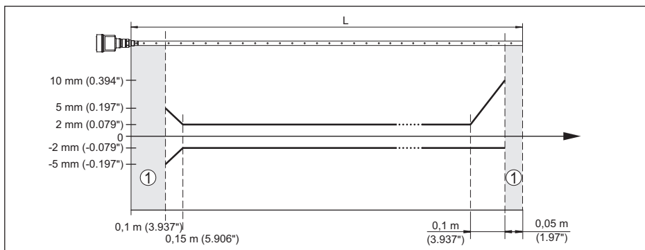
Abb. 28: Messabweichung VEGAFLEX 81 in Koaxialausführung in Medium Öl
