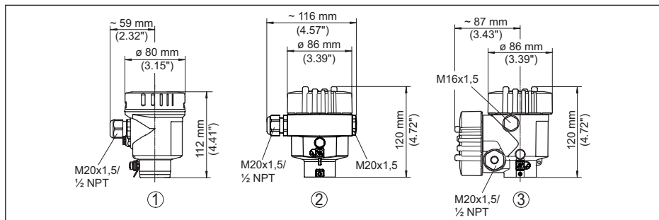
Abb. 41: Gehäuseausführungen in Schutzart IP66/IP68 (0,2 bar), (mit eingebautem Anzeige- und Bedienmodul vergrößert sich die Gehäusehöhe um 18 mm/0.71 in)
