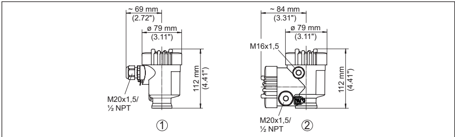
Abb. 38: Gehäuseausführungen in Schutzart IP66/IP67 (mit eingebautem Anzeige- und Bedienmodul vergrößert sich die Gehäusehöhe um 9 mm/0.35 in)
