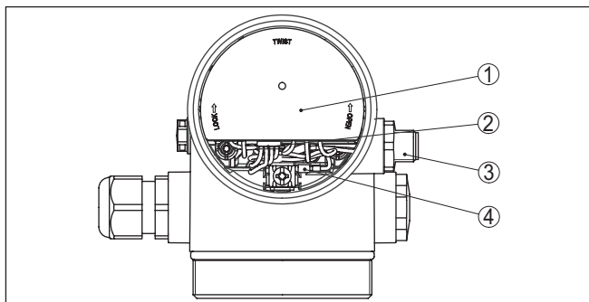
Abb. 15: Sicht auf den Elektronikraum mit VEGADIS-Adapter zum Anschluss der externen Anzeige- und Bedieneinheit
