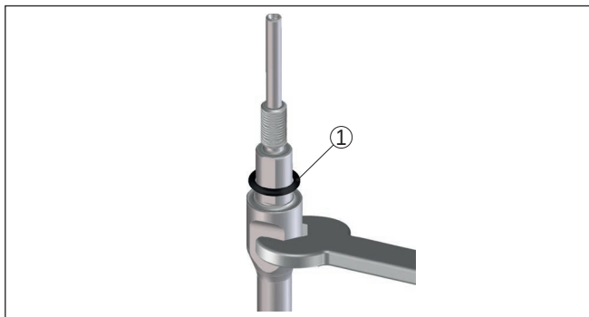
Abb. 31: Messstab wechseln
