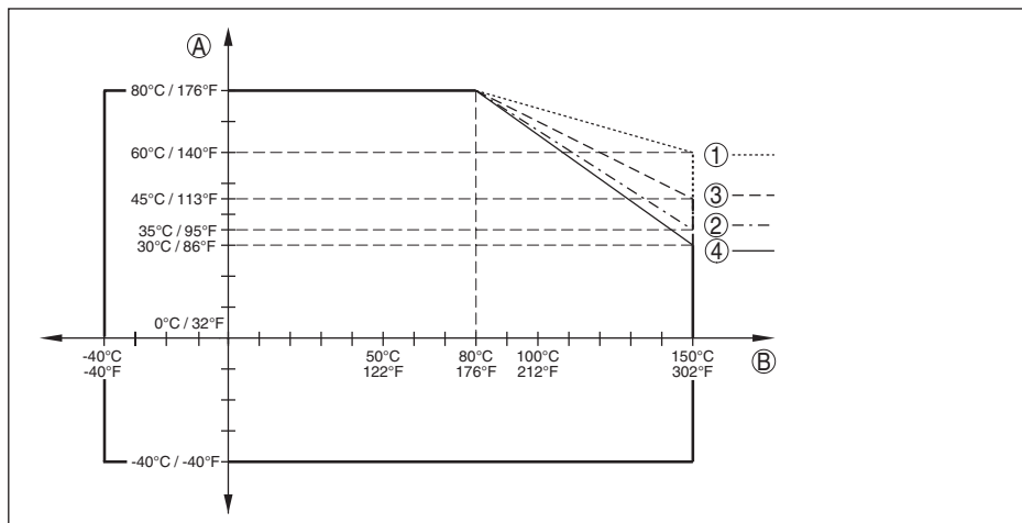
Abb. 37: Umgebungstemperatur - Prozesstemperatur, Standardausführung
