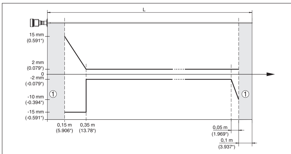
Abb. 36: Messabweichung VEGAFLEX 83 in Stabausführung in Medium Öl
