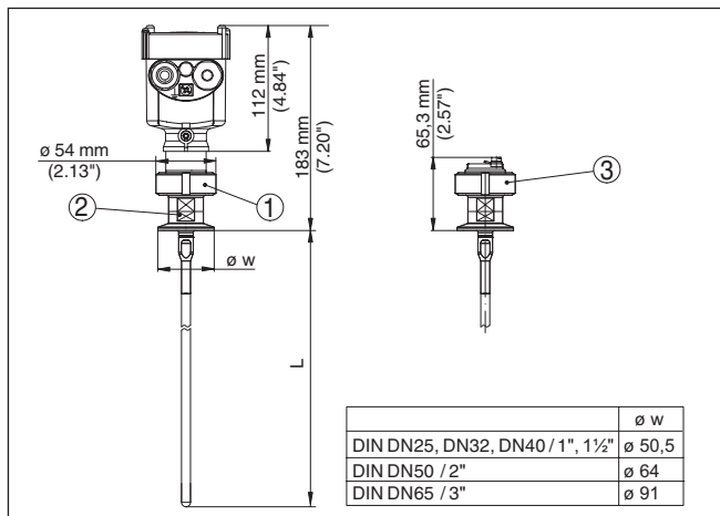
Abb. 8: Autoklavierbare Ausführung
