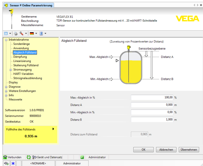
Abb. 28: Beispiel einer DTM-Ansicht
