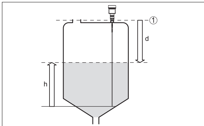
Abb. 1: Füllstandmessung
