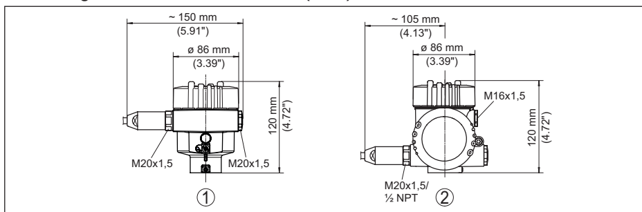
Abb. 40: Gehäuseausführungen in Schutzart IP66/IP68 (1 bar), (mit eingebautem Anzeige- und Bedienmodul vergrößert sich die Gehäusehöhe um 18 mm/0.71 in)
