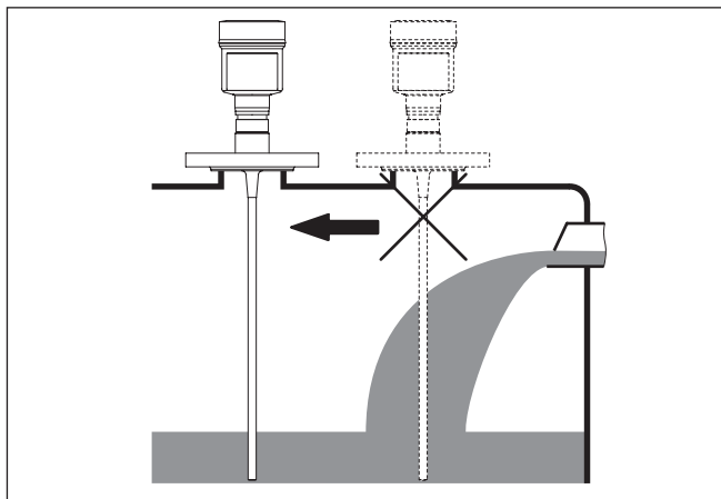
Abb. 7: Montage des Sensors bei einströmendem Medium
