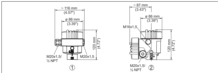
Abb. 39: Gehäuseausführungen in Schutzart IP66/IP68 (0,2 bar), (mit eingebautem Anzeige- und Bedienmodul vergrößert sich die Gehäusehöhe um 18 mm/0.71 in)
