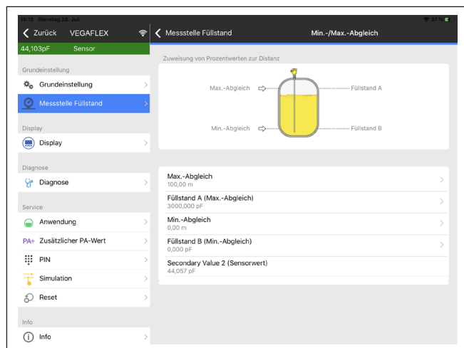
Abb. 25: Beispiel einer App-Ansicht - Inbetriebnahme Sensorabgleich
