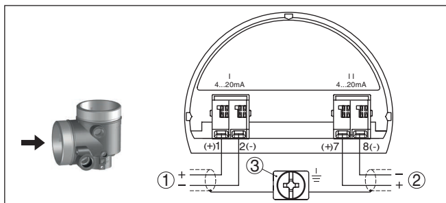
Abb. 18: Anschlussraum Zweikammergehäuse, Zusatzelektronik - Zusätzlicher Stromausgang
