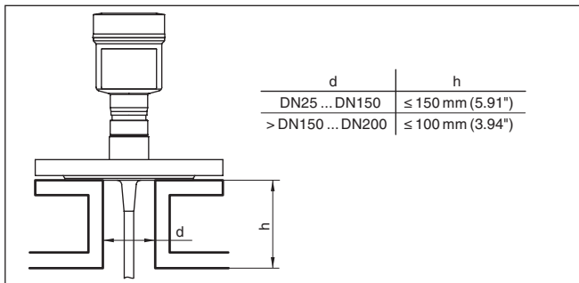
Abb. 5: Montagestutzen
