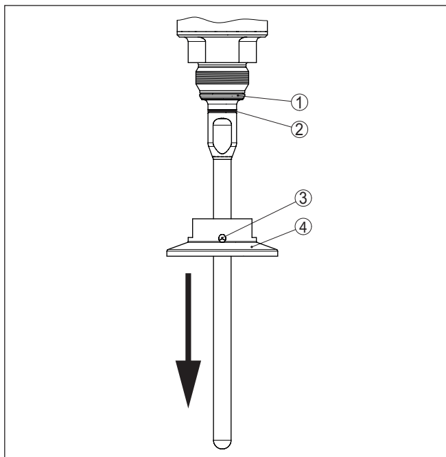
Abb. 33: Dichtung - Prozessanschluss
