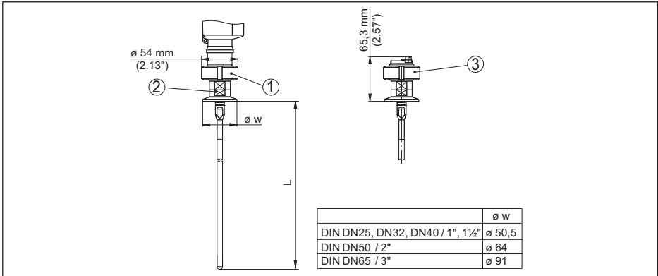
Abb. 44: VEGAFLEX 83, Stabausführung ø 8 mm (0.315 in), poliert - Autoklavierbare Ausführung
