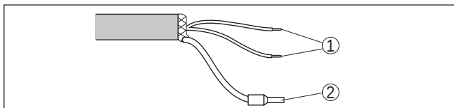
Abb. 17: Aderbelegung fest angeschlossenes Anschlusskabel
