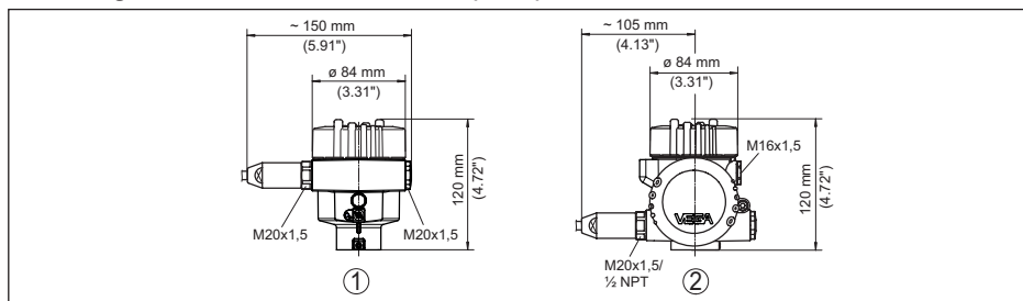
Abb. 42: Gehäuseausführungen in Schutzart IP66/IP68 (1 bar), (mit eingebautem Anzeige- und Bedienmodul vergrößert sich die Gehäusehöhe um 18 mm/0.71 in)
