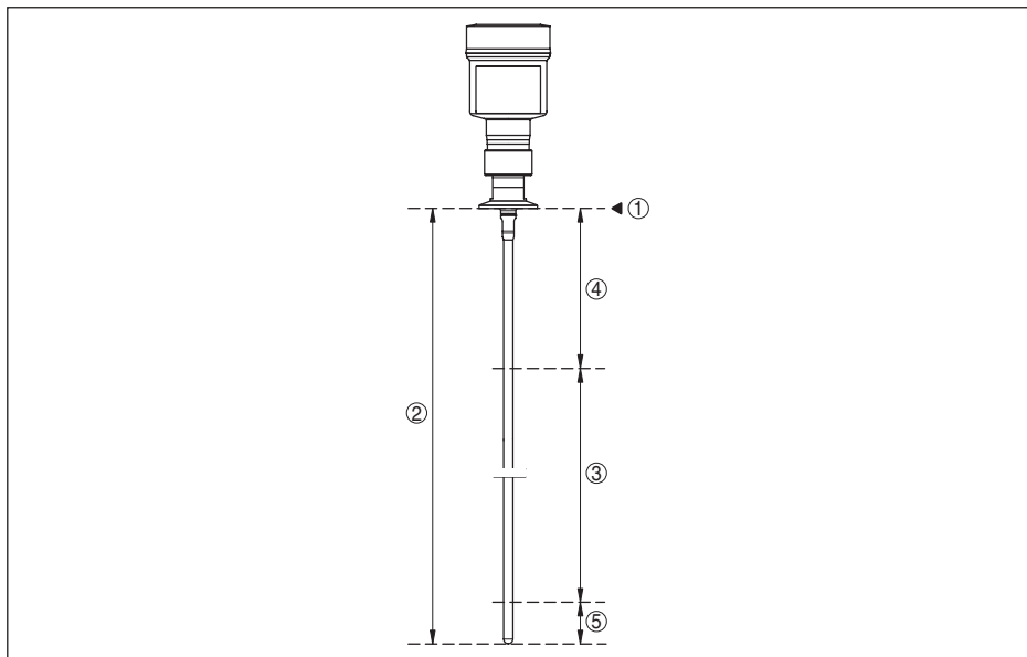
Abb. 34: Messbereiche - VEGAFLEX 83
