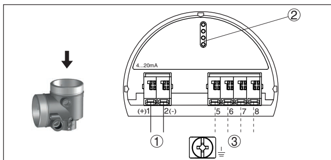
Abb. 13: Elektronikraum - Zweikammergehäuse
