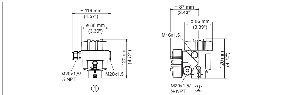
Abb. 38: Gehäuseausführungen in Schutzart IP66/IP68 (0,2 bar), (mit eingebautem Anzeige- und Bedienmodul vergrößert sich die Gehäusehöhe um 18 mm/0.71 in)
