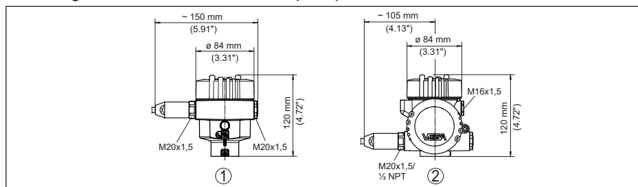
Abb. 41: Gehäuseausführungen in Schutzart IP66/IP68 (1 bar), (mit eingebautem Anzeige- und Bedienmodul vergrößert sich die Gehäusehöhe um 18 mm/0.71 in)
