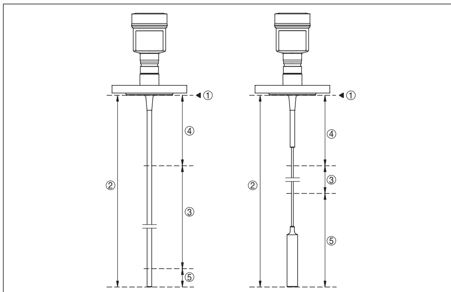
Abb. 31: Messbereiche - VEGAFLEX 83
