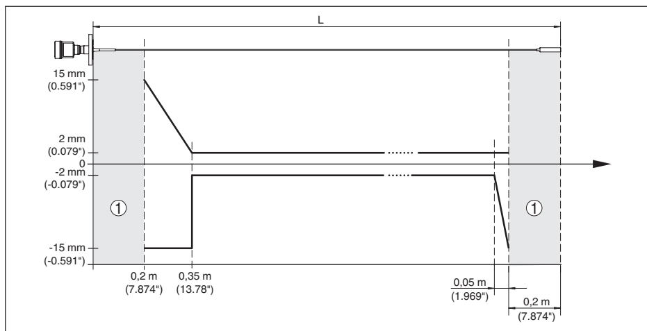
Abb. 35: Messabweichung VEGAFLEX 83 in Seilausführung (beschichtet) in Medium Öl
