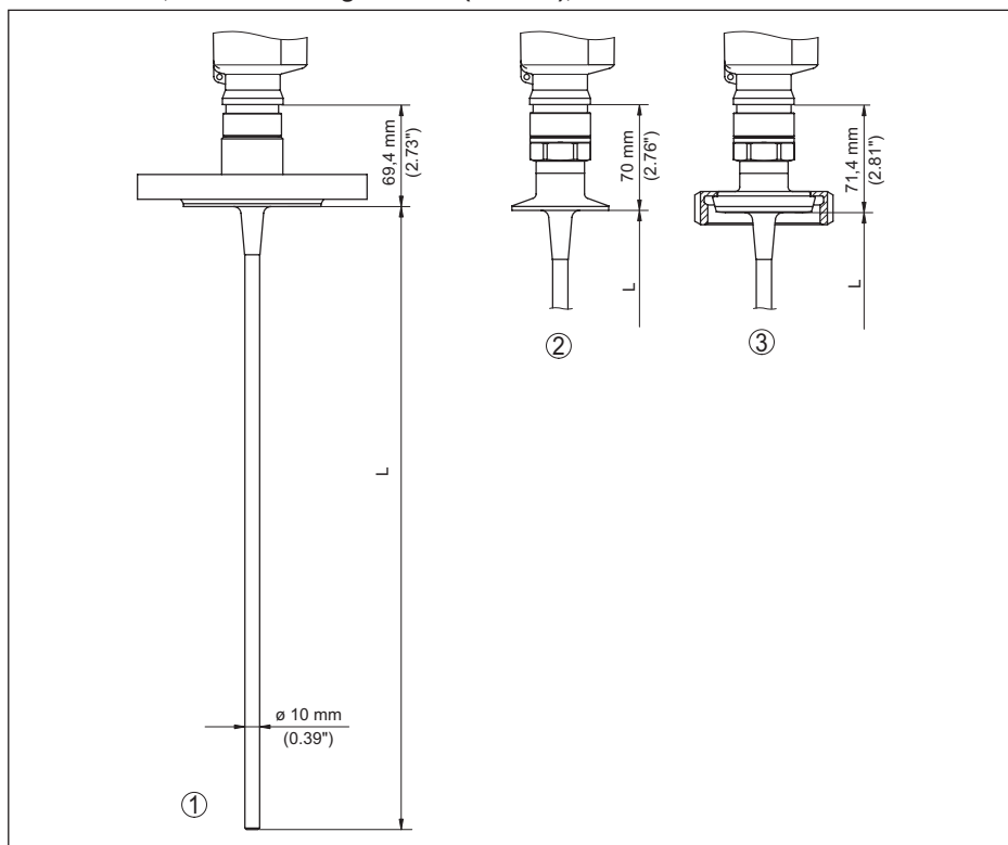
Abb. 43: VEGAFLEX 83, Stabausführung
