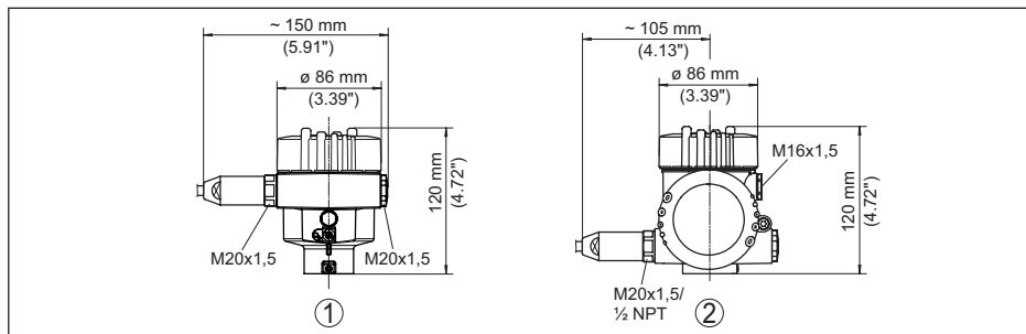
Abb. 39: Gehäuseausführungen in Schutzart IP66/IP68 (1 bar), (mit eingebautem Anzeige- und Bedienmodul vergrößert sich die Gehäusehöhe um 18 mm/0.71 in)
