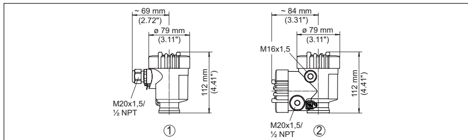
Abb. 37: Gehäuseausführungen in Schutzart IP66/IP67 (mit eingebautem Anzeige- und Bedienmodul vergrößert sich die Gehäusehöhe um 9 mm/0.35 in)
