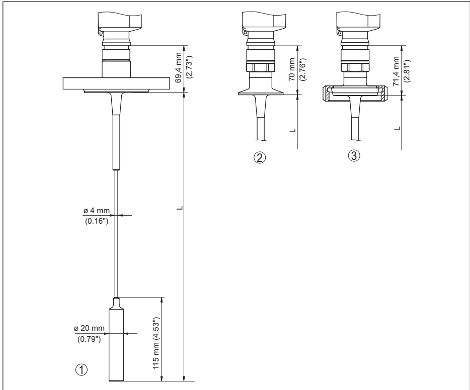
Abb. 42: VEGAFLEX 83, Seilausführung mit Straffgewicht
