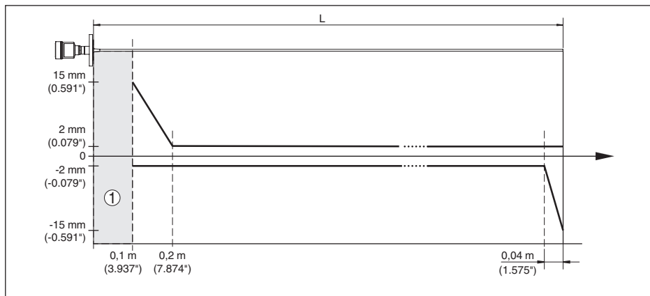
Abb. 32: Messabweichung VEGAFLEX 83 in Stabausführung (beschichtet) in Medium Wasser
