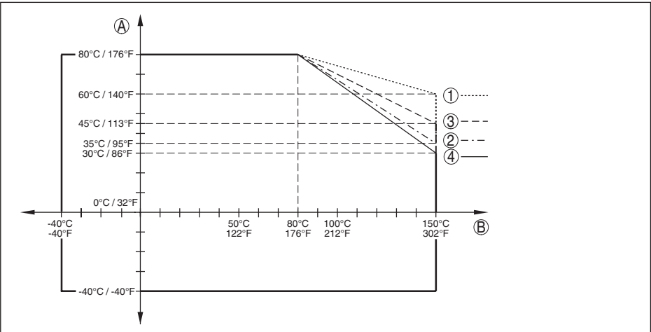
Abb. 36: Umgebungstemperatur - Prozesstemperatur, Standardausführung
