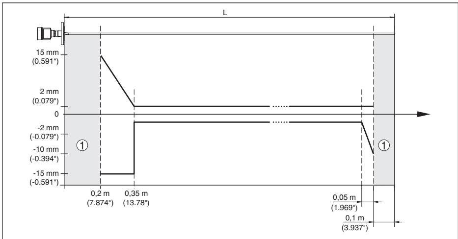
Abb. 31: Messabweichung VEGAFLEX 83 in Stabausführung (beschichtet) in Medium Öl
