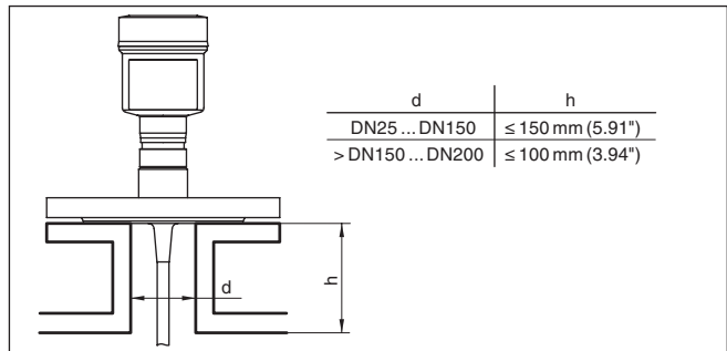
Abb. 6: Montagestutzen
