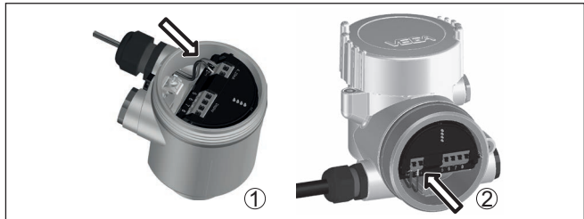
Abb. 10: Anschlusschritte 5 und 6
