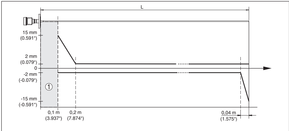
Abb. 30: Messabweichung VEGAFLEX 83 in Stabausführung (beschichtet) in Medium Wasser
