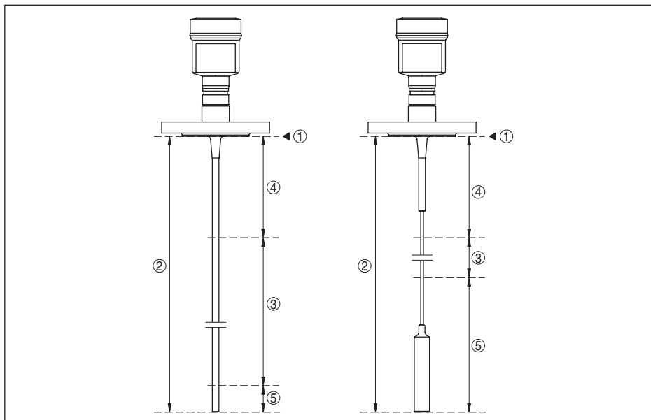
Abb. 29: Messbereiche - VEGAFLEX 83
