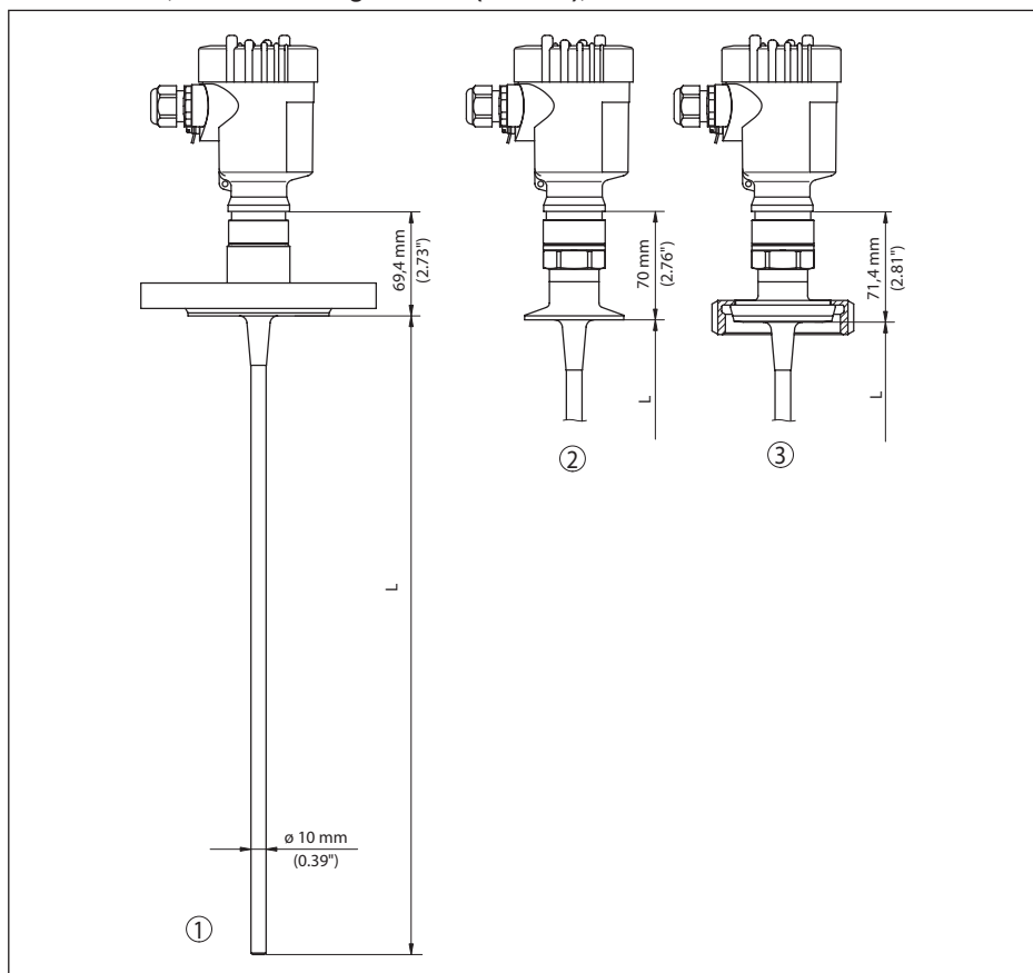
Abb. 41: VEGAFLEX 83, Stabausführung
