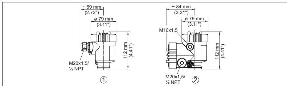
Fig. 41: Variantes de boîtier en protection IP66/IP67 (avec un module de réglage et d'affichage intégré, la hauteur du boîtier augmente de 9 mm/0.35 in)
