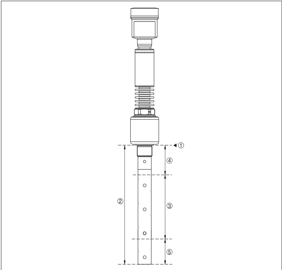
Fig. 28: Plages de mesure - VEGAFLEX 86
