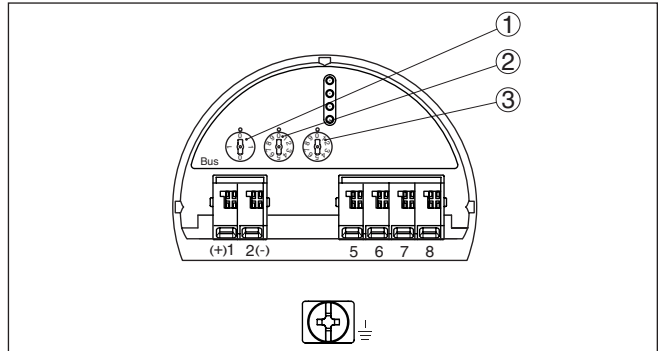
Fig. 15: Bouton de sélection d'adresse
