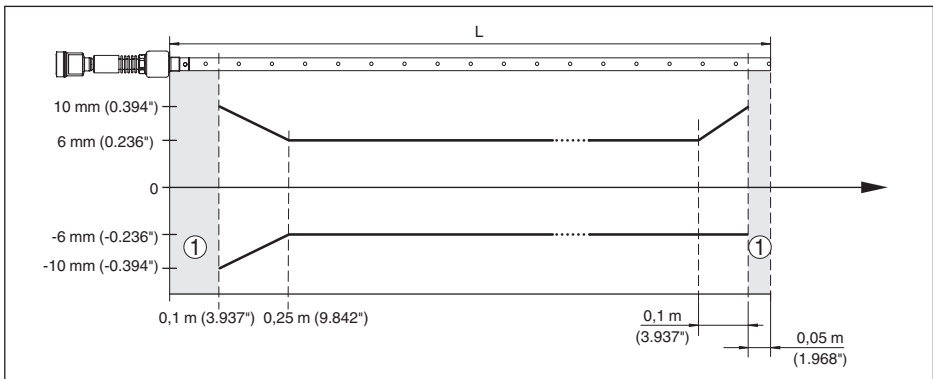
Fig. 32: Écart de mesure VEGAFLEX 86 en version coaxiale dans l'huile (longueur de mesure jusqu'à 6 m/19.69 ft)
