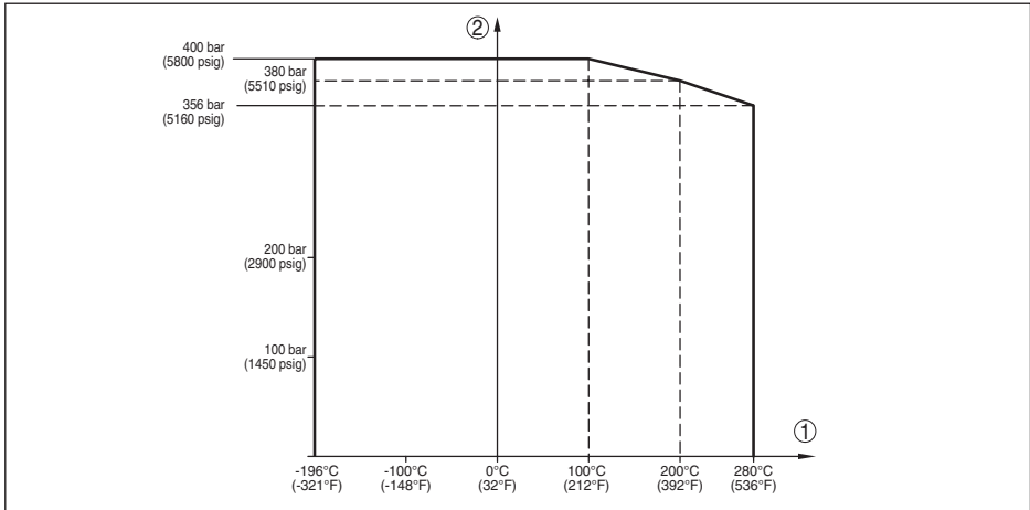
Fig. 36: Pression process - température du process (version -196 ... +280 °C/-321 ... +536 °F)
