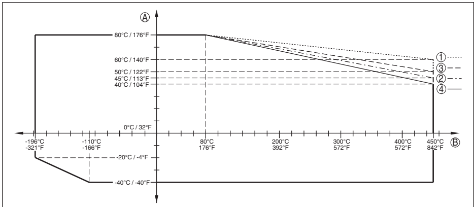
Fig. 35: Température ambiante - température process, version standard
