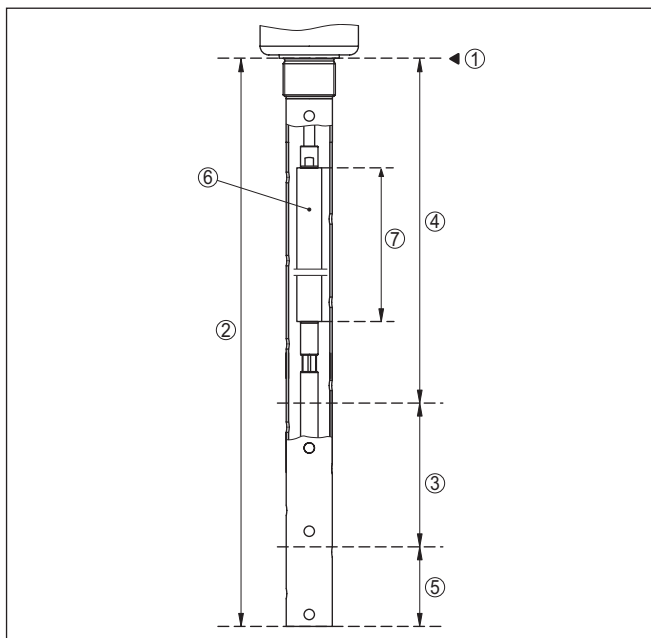
Fig. 33: Plages de mesure - VEGAFLEX 86 avec compensation de la vapeur
