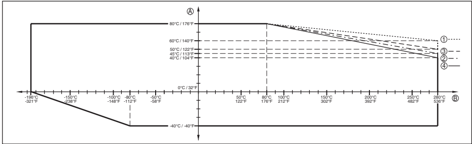
Fig. 34: Température ambiante - température process, version standard
