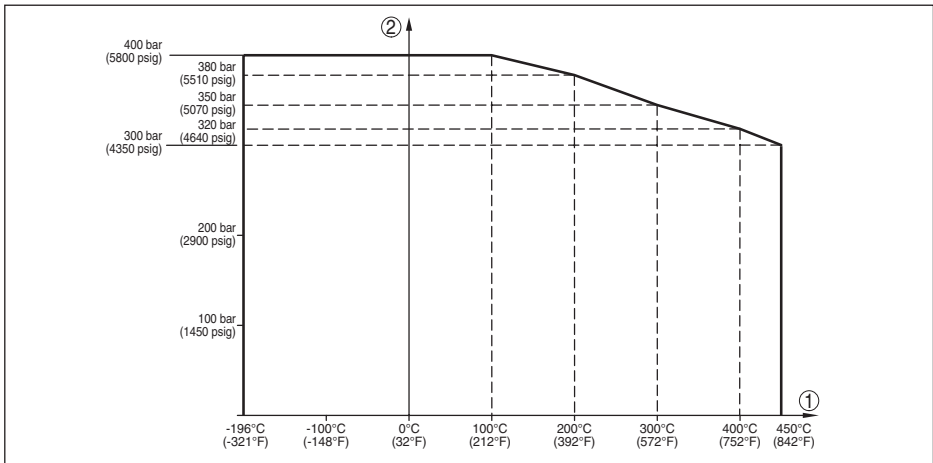
Fig. 37: Pression process - température du process (version -196 ... +450 °C/-321 ... +842 °F)
