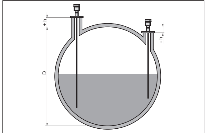
Fig. 20: Hauteur de la cuve et valeur de correction du manchon
