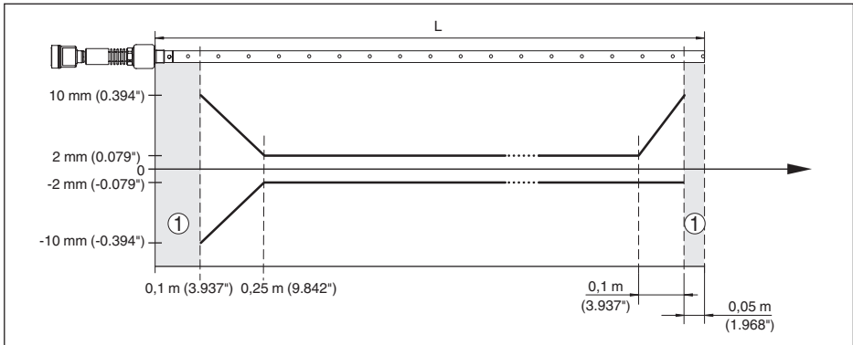
Fig. 31: Écart de mesure VEGAFLEX 86 en version coaxiale dans l'huile (longueur de mesure jusqu'à 1,5 m/4.92 ft)
