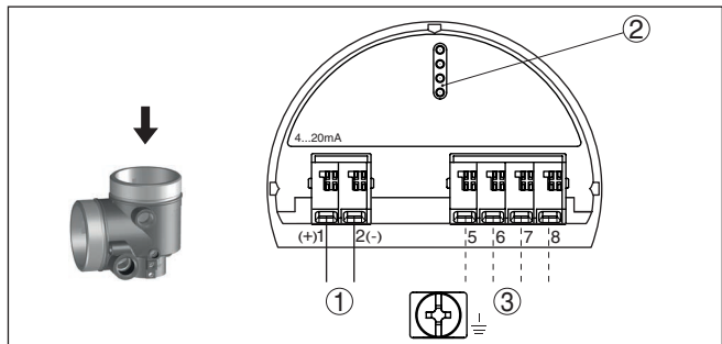
Fig. 12: Compartiment électronique - boîtier à deux chambres
