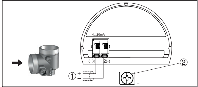
Fig. 13: Compartiment de raccordement - Boîtier à deux chambres Ex d ia
