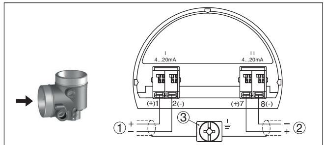
Fig. 17: Compartiment de raccordement boîtier à deux chambres, électronique supplémentaire - sortie courant supplémentaire
