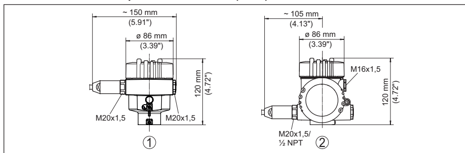
Fig. 42: Variantes de boîtier en protection IP66/IP68 (1 bar), (avec un module de réglage et d'affichage intégré, la hauteur du boîtier augmente de 18 mm/0.71 in)
