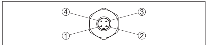
Fig. 15: Vue sur le connecteur M12 x 1
