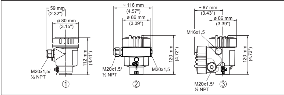
Fig. 43: Variantes de boîtier en protection IP66/IP68 (0,2 bar), (avec un module de réglage et d'affichage intégré, la hauteur du boîtier augmente de 18 mm/0.71 in)
