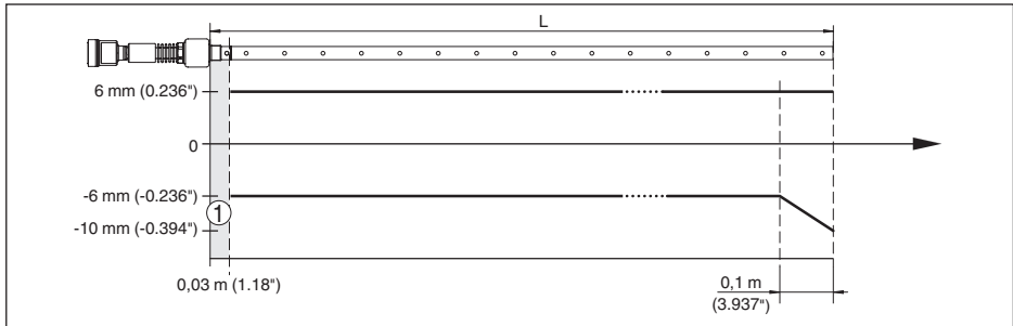
Fig. 32: Écart de mesure VEGAFLEX 86 en version coaxiale dans l'eau (longueur de mesure jusqu'à 6 m/19.69 ft)
