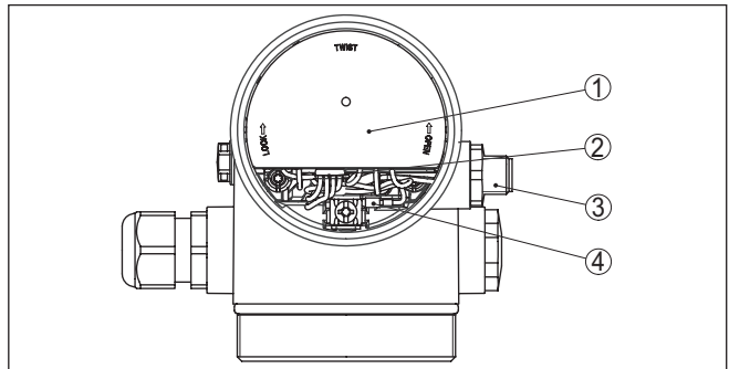
Fig. 14: Vue sur le compartiment de l'électronique avec l'adaptateur VEGADIS pour le raccordement de l'unité de réglage et d'affichage
