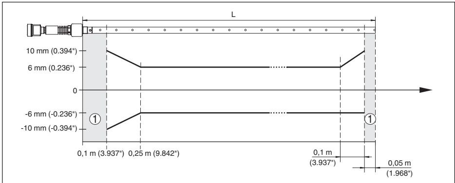
Fig. 34: Écart de mesure VEGAFLEX 86 en version coaxiale dans l'huile (longueur de mesure jusqu'à 6 m/19.69 ft)
