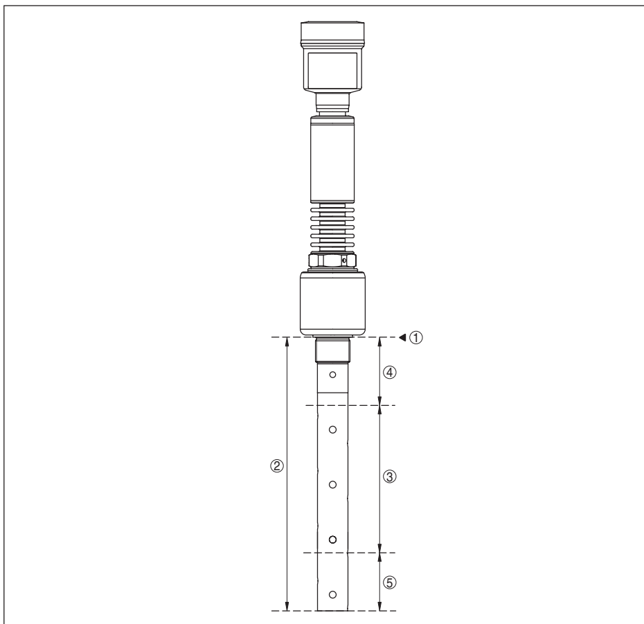
Fig. 30: Plages de mesure - VEGAFLEX 86
