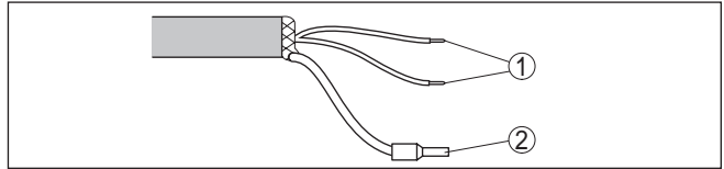
Fig. 16: Affectation des conducteurs du câble de raccordement raccordé de façon fixe
