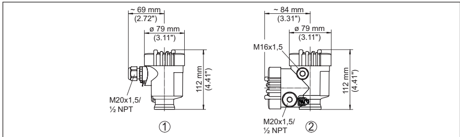
Fig. 40: Variantes de boîtier en protection IP66/IP67 (avec un module de réglage et d'affichage intégré, la hauteur du boîtier augmente de 9 mm/0.35 in)
