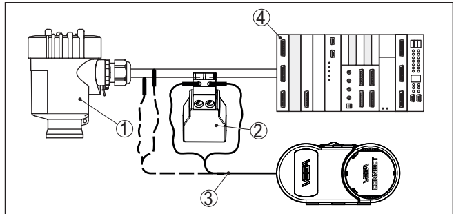
Fig. 26: Raccordement du PC à la ligne signal via HART
