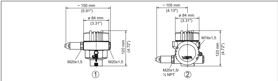
Fig. 44: Variantes de boîtier en protection IP66/IP68 (1 bar), (avec un module de réglage et d'affichage intégré, la hauteur du boîtier augmente de 18 mm/0.71 in)
