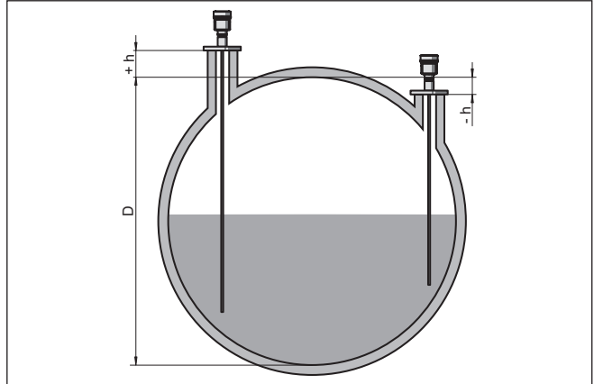
Fig. 22: Hauteur de la cuve et valeur de correction du manchon
