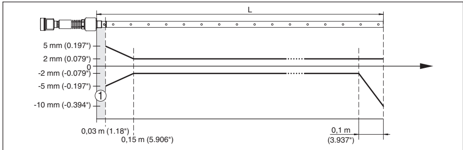
Fig. 31: Écart de mesure VEGAFLEX 86 en version coaxiale dans l'eau (longueur de mesure jusqu'à 1,5 m/4.92 ft)
