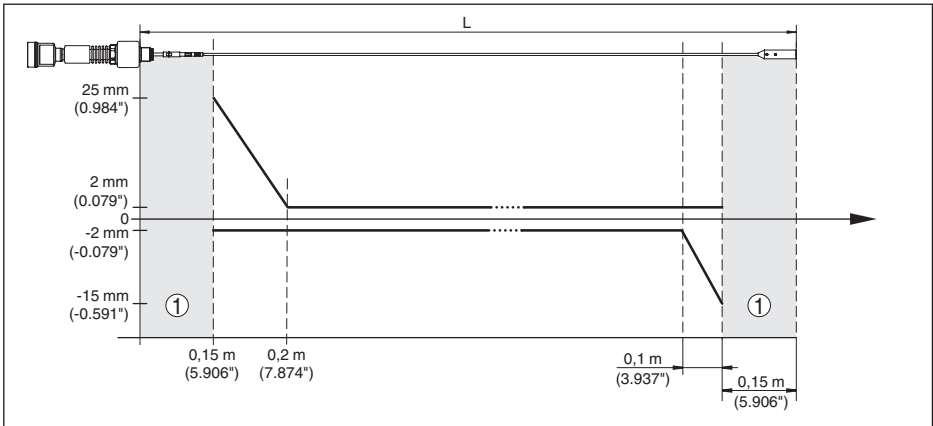
Fig. 38: Meetafwijking VEGAFLEX 86 in kabeluitvoering (4 mm/0.157 in), in medium olie
