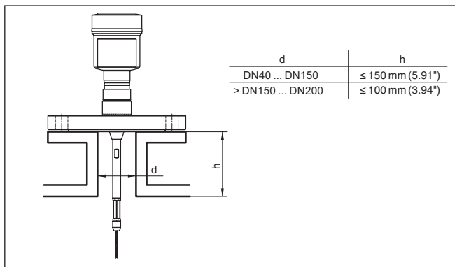
Fig. 6: Montagesok
