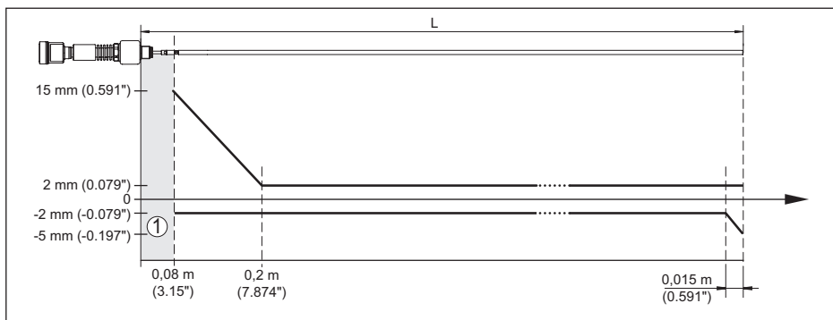
Fig. 34: Meetnauwkeurigheid VEGAFLEX 86 in staafuitvoering in medium water
