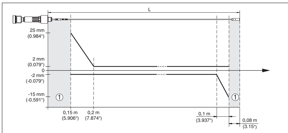
Fig. 37: Meetafwijking VEGAFLEX 86 in kabeluitvoering (2 mm/0.079 in), in medium olie
