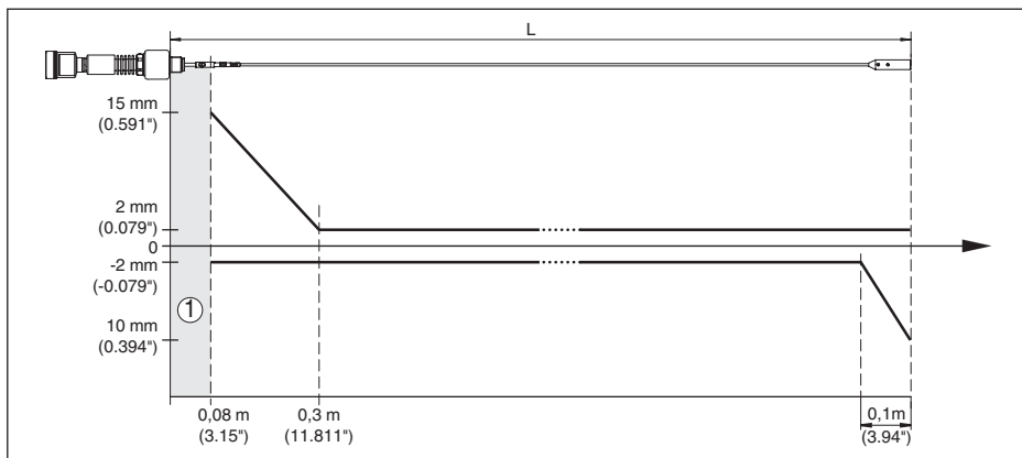
Fig. 36: Meetnauwkeurigheid VEGAFLEX 86 in kabeluitvoering in medium water
