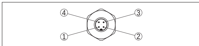
Fig. 19: Zicht op de M12 x 1-stekkerverbinding
