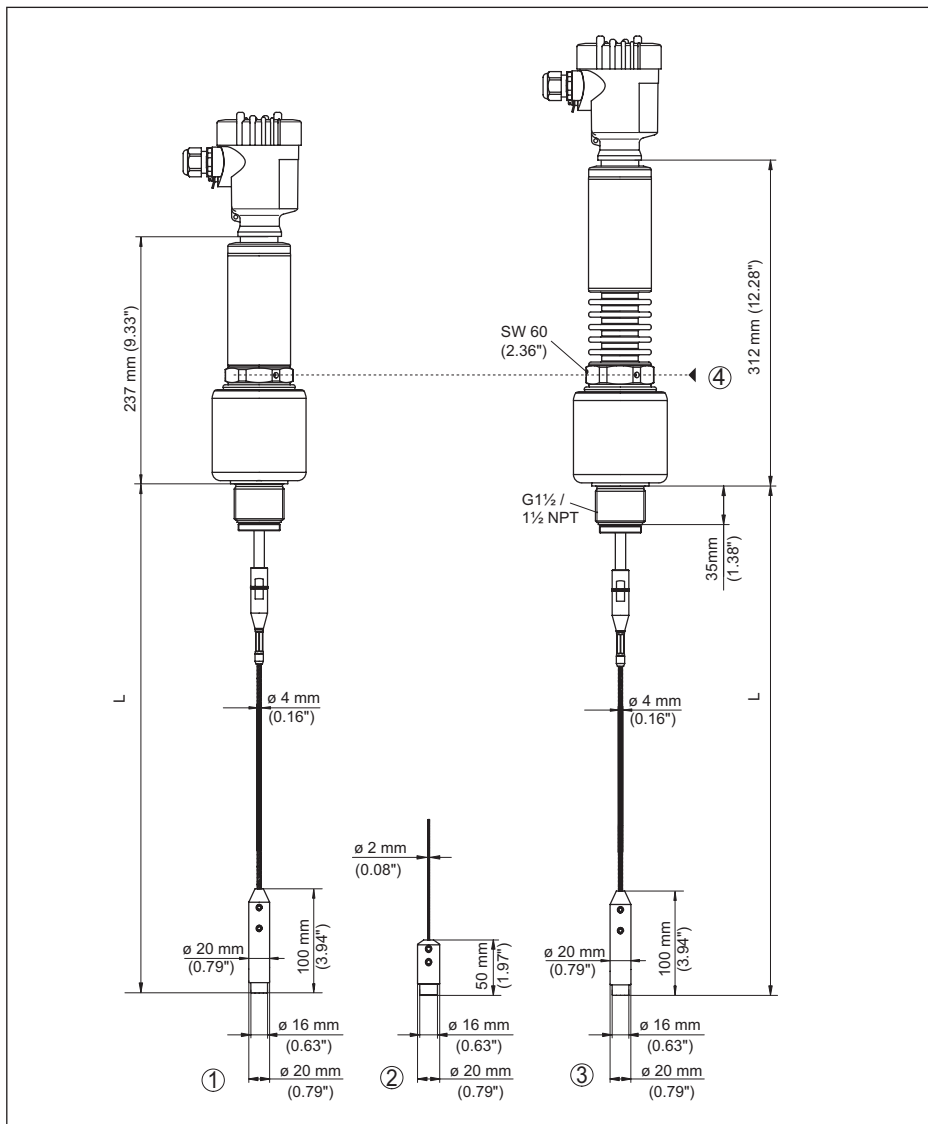
Fig. 51: VEGAFLEX 86, schroefdraaduitvoering met spangewicht (alle spangewichten met schroefdraad M8 voor oogbout)
