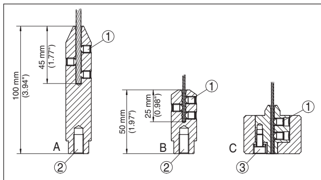
Fig. 32: Kabelmeetsonde inkorten
