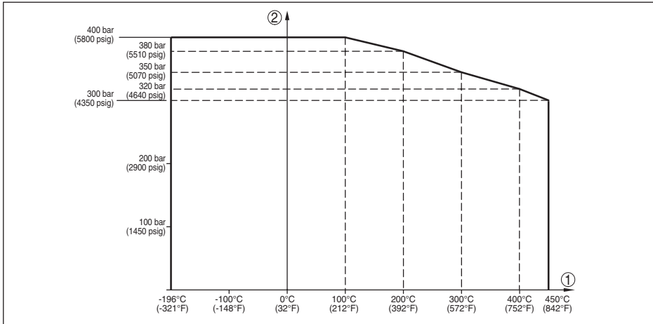
Fig. 42: Procesdruk - procestemperatuur (uitvoering -196 ... +450 °C/-321 ... +842 °F)
