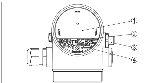
Fig. 18: Een blik op de elektronicaruimte met VEGADIS-adapter voor aansluiting van de externe display- en bedieningseenheid
