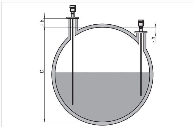
Fig. 25: Tankhoogte en sokcorrectiewaarde
