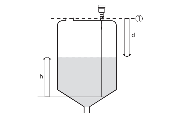
Fig. 2: Niveaumeting
