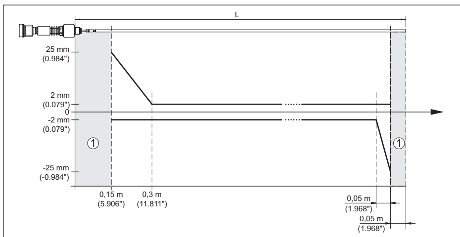
Fig. 35: Meetnauwkeurigheid VEGAFLEX 86 in staafuitvoering in medium olie
