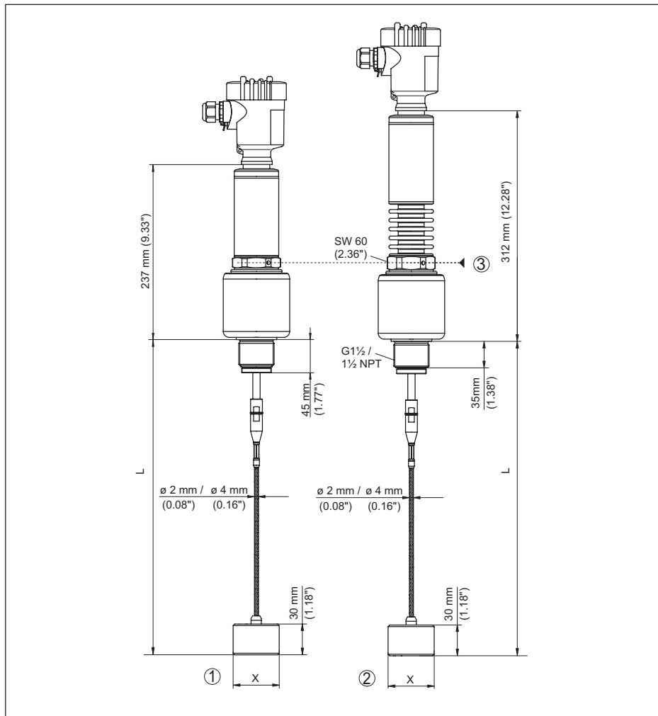
Fig. 52: VEGAFLEX 86, schroefdraaduitvoering met centreergewicht
