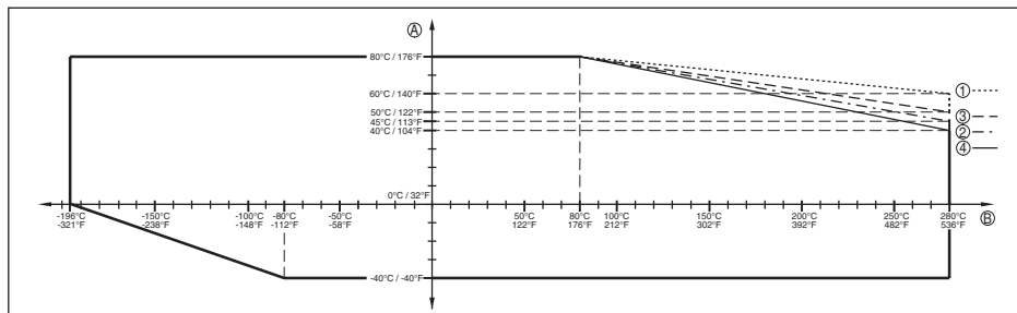
Fig. 39: Omgevingstemperatuur - procestemperatuur standaarduitvoering
