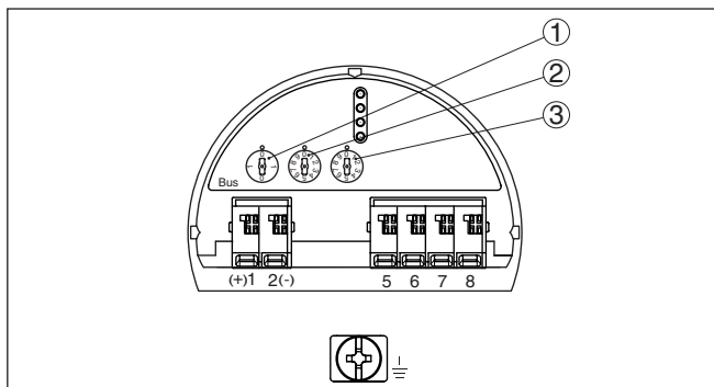
Fig. 21: Adreskeuzeschakelaar
