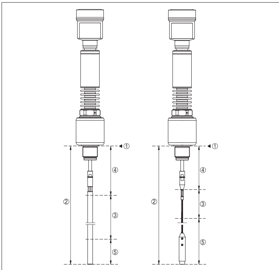
Fig. 33: Meetbereiken - VEGAFLEX 86
