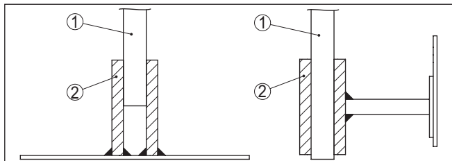
Abb. 12: Messsonde fixieren
