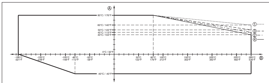
Abb. 41: Umgebungstemperatur - Prozesstemperatur, Standardausführung
