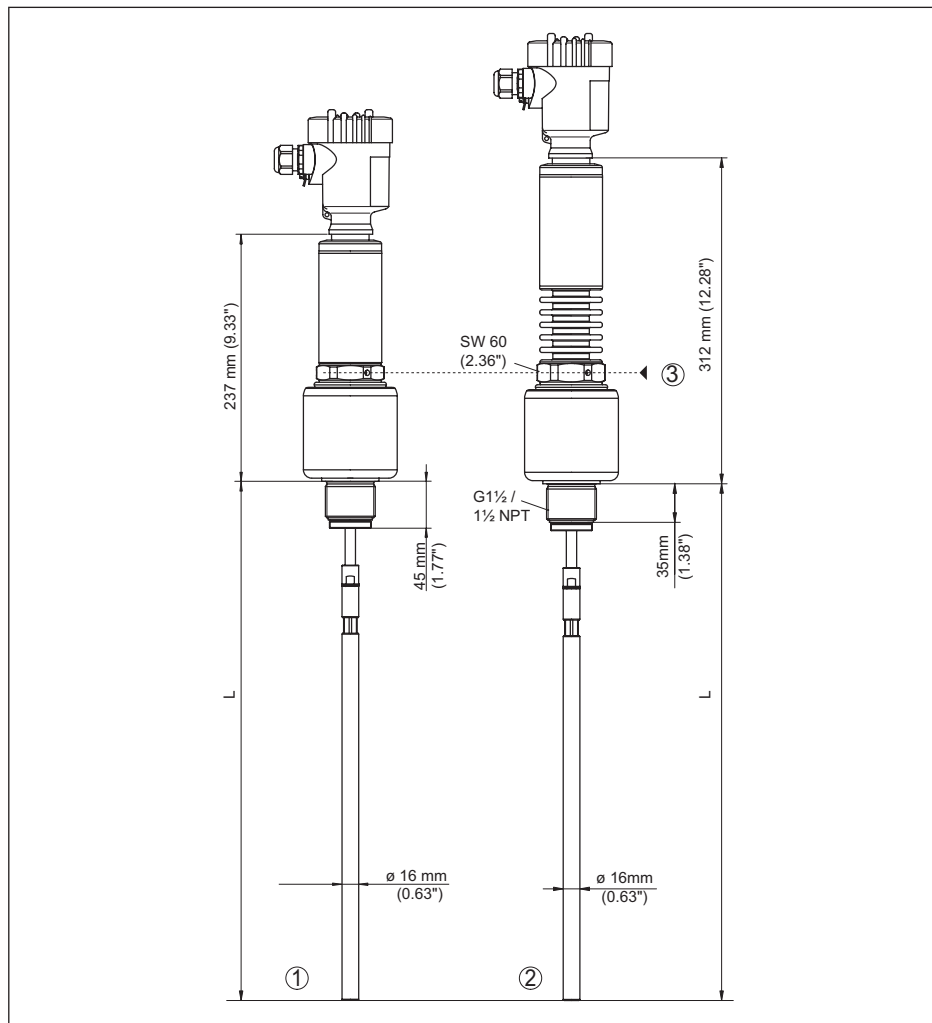
Abb. 52: VEGAFLEX 86, Gewindeausführung
