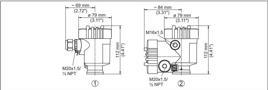
Abb. 45: Gehäuseausführungen in Schutzart IP66/IP67 (mit eingebautem Anzeige- und Bedienmodul vergrößert sich die Gehäusehöhe um 9 mm/0.35 in)
