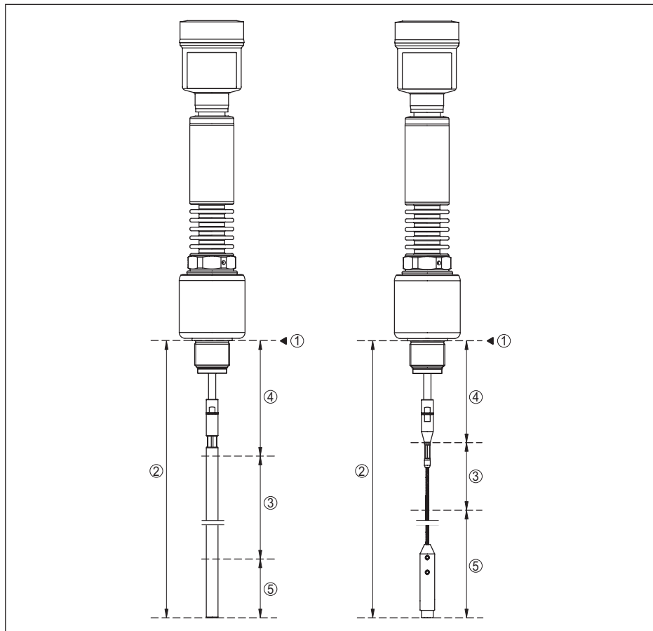
Abb. 35: Messbereiche - VEGAFLEX 86
