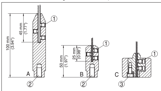
Abb. 34: Seilmesssonde kürzen
