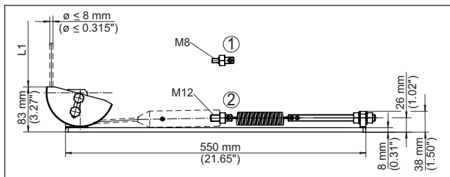
Abb. 13: Abspannvorrichtung für Seilausführungen
