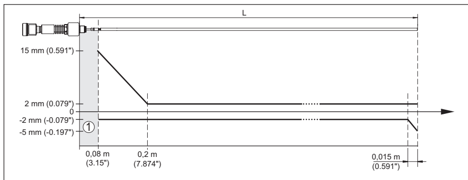
Abb. 36: Messabweichung VEGAFLEX 86 in Stabausführung in Medium Wasser
