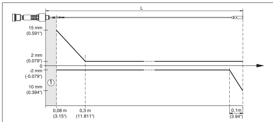
Abb. 38: Messabweichung VEGAFLEX 86 in Seilausführung in Medium Wasser
