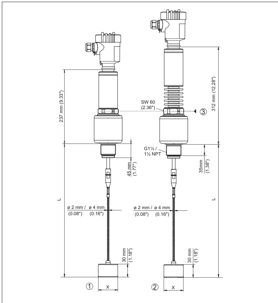
Abb. 51: VEGAFLEX 86, Gewindeausführung mit Zentriergewicht
