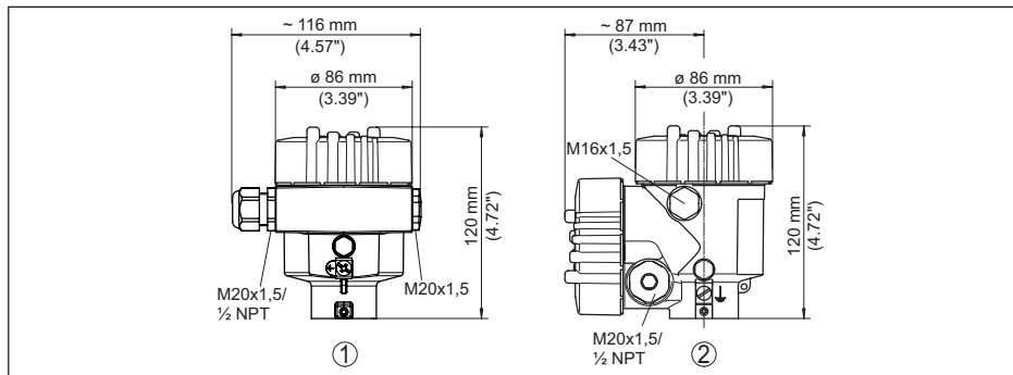
Abb. 46: Gehäuseausführungen in Schutzart IP66/IP68 (0,2 bar), (mit eingebautem Anzeige- und Bedienmodul vergrößert sich die Gehäusehöhe um 9 mm/0.35 in)
