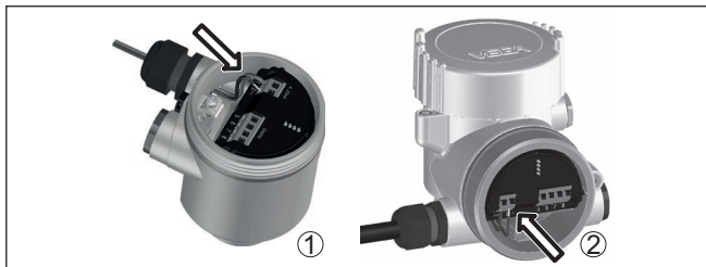
Abb. 14: Anschlusssschritte 5 und 6
