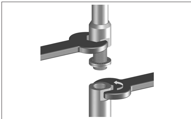
Abb. 33: Messseil bzw. Messstab wechseln
