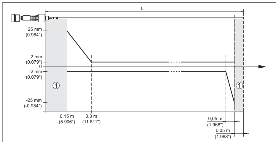
Abb. 37: Messabweichung VEGAFLEX 86 in Stabausführung in Medium Öl
