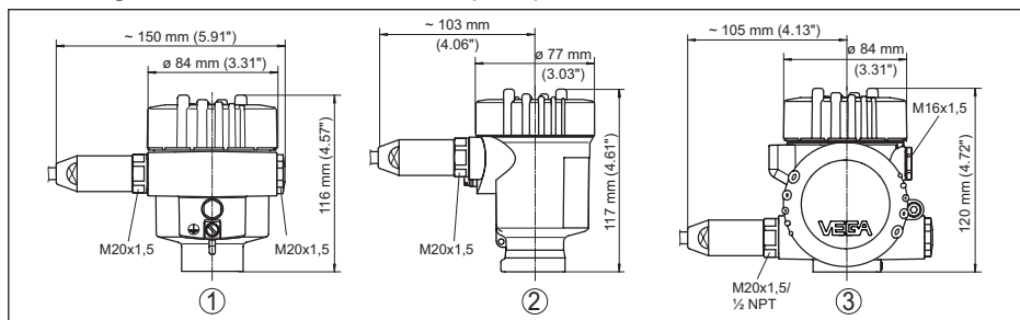
Abb. 49: Gehäuseausführungen in Schutzart IP66/IP68 (1 bar), (mit eingebautem Anzeige- und Bedienmodul vergrößert sich die Gehäusehöhe um 9 mm/0.35 in)
