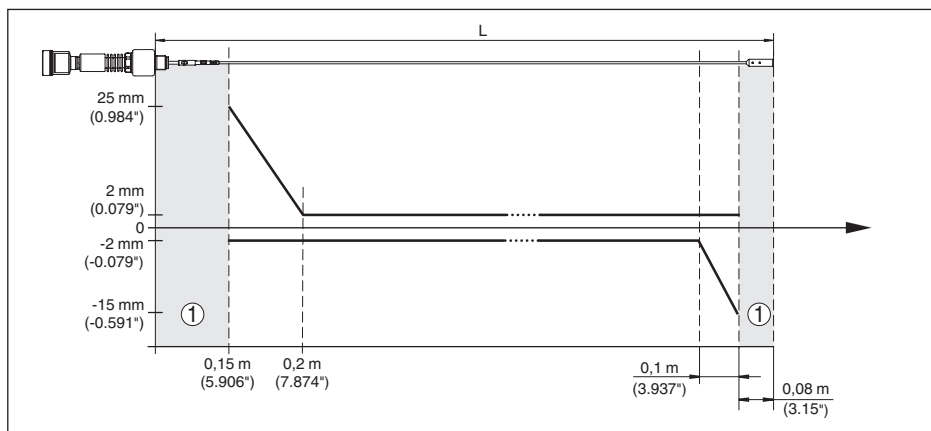
Abb. 39: Messabweichung VEGAFLEX 86 in Seilausführung (2 mm/0.079 in), in Medium Öl
