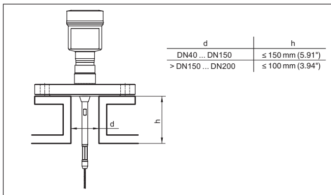
Abb. 6: Montagesutzen
