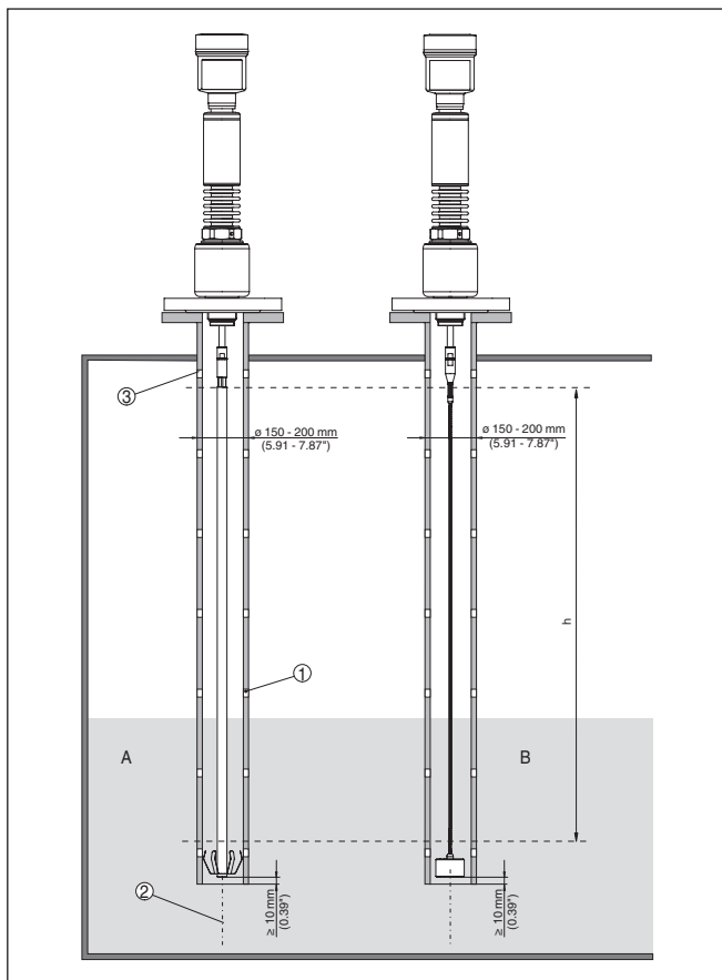
Abb. 10: Montage in einem Standrohr
