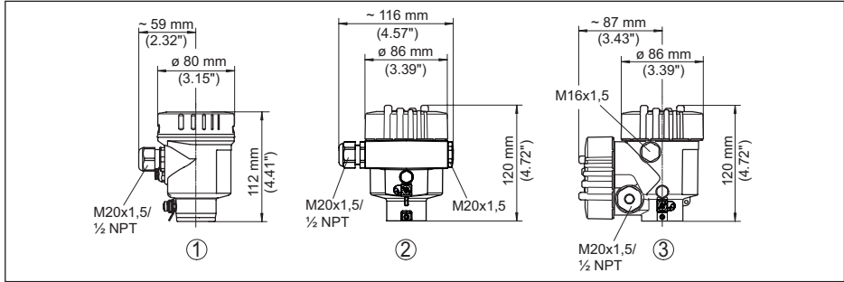
Fig. 50: Variantes de boîtier en protection IP66/IP68 (0,2 bar), (avec un module de réglage et d'affichage intégré, la hauteur du boîtier augmente de 18 mm/0.71 in)
