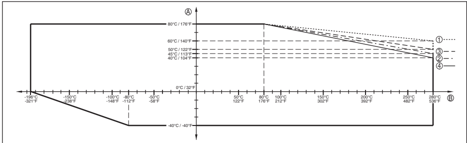
Fig. 43: Température ambiante - température process, version standard
