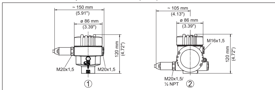
Fig. 49: Variantes de boîtier en protection IP66/IP68 (1 bar), (avec un module de réglage et d'affichage intégré, la hauteur du boîtier augmente de 18 mm/0.71 in)
