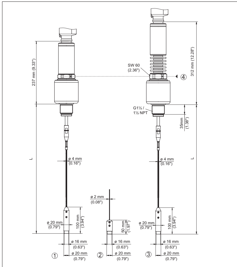
Fig. 52: VEGAFLEX 86, version filetée avec poids tenseur (tous les poids tenseurs avec filetage M8 pour anneau de levage)
