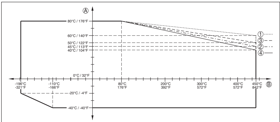
Fig. 44: Température ambiante - température process, version standard
