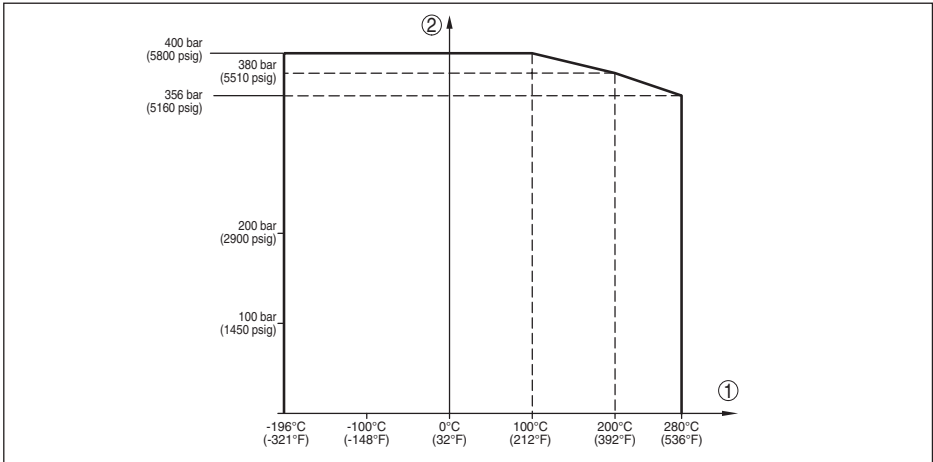
Fig. 45: Pression process - température du process (version -196 ... +280 °C/-321 ... +536 °F)
