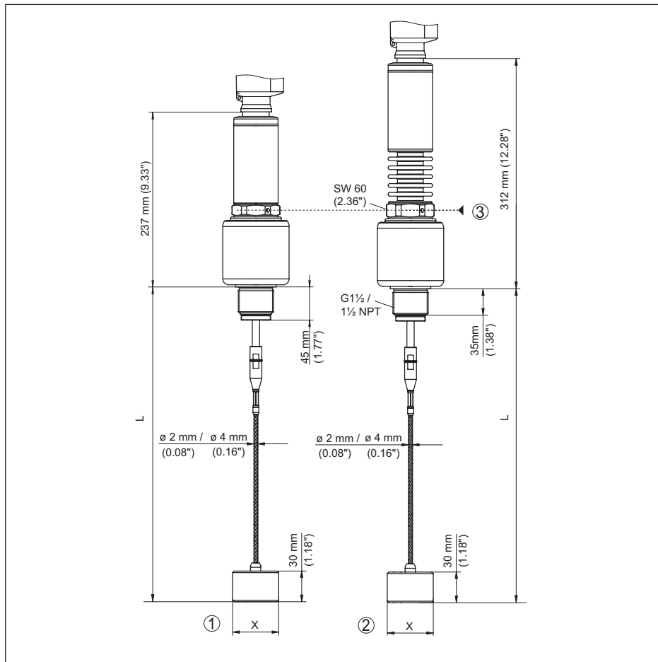
Fig. 53: VEGAFLEX 86, version filetée avec poids de centrage
