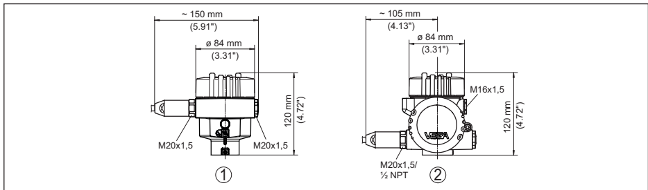
Fig. 51: Variantes de boîtier en protection IP66/IP68 (1 bar), (avec un module de réglage et d'affichage intégré, la hauteur du boîtier augmente de 18 mm/0.71 in)
