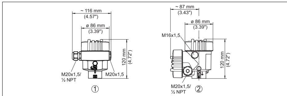
Fig. 48: Variantes de boîtier en protection IP66/IP68 (0,2 bar), (avec un module de réglage et d'affichage intégré, la hauteur du boîtier augmente de 18 mm/0.71 in)
