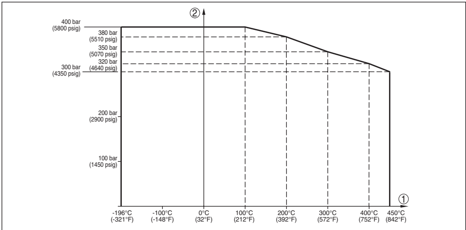
Fig. 46: Pression process - température du process (version -196 ... +450 °C/-321 ... +842 °F)
