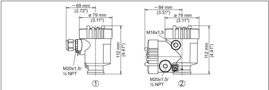
Fig. 45: Huisuitvoeringen in beschermingsklasse IP66/IP67 (met ingebouwde aanwijs- en bedieningsmodule wordt het huis 9 mm hoger)
