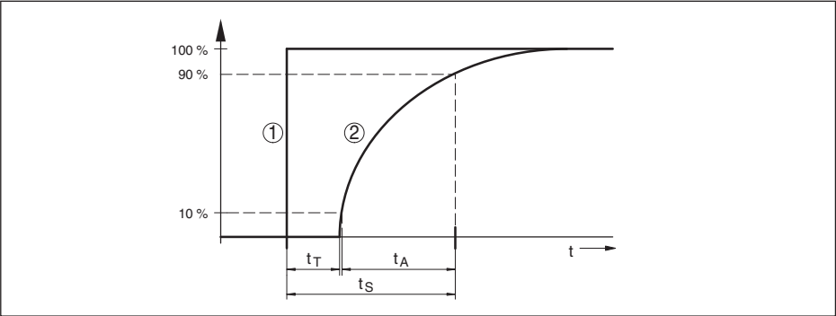
Fig. 37: Spronggewijze verandering van de proceseenheid. t_T : dode band; t_A : toenametijd; t_S : sprongantwoordtijd
