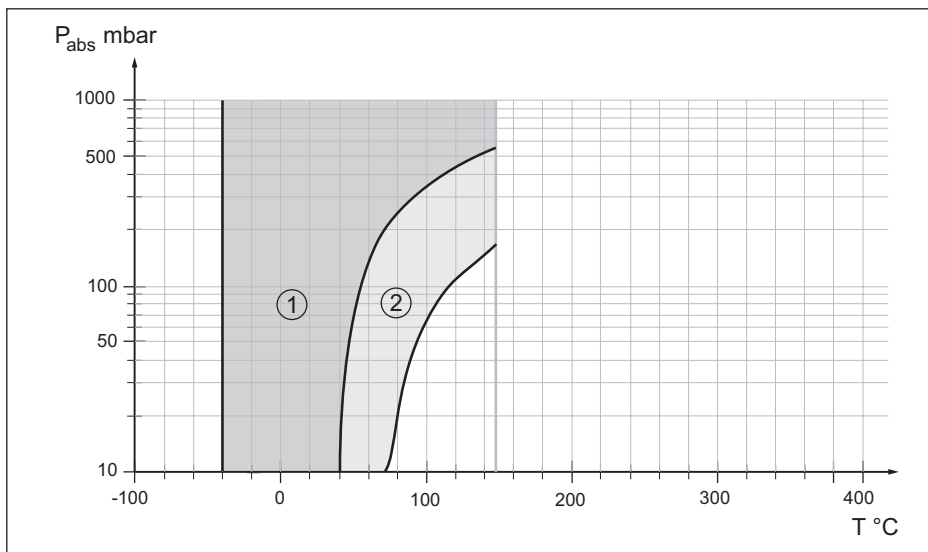
Fig. 42: Toepassingsgebied voor halocarbonolie KN 21
