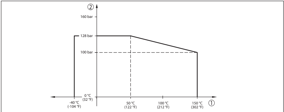
Fig. 38: Temperatuur derating VEGABAR 81, procesaansluitingen Alloy 400 (2.4360)
