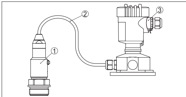
Fig. 24: VEGABAR 81 in IP68-uitvoering 25 bar met axiale kabeluitgang, externe behuizing
