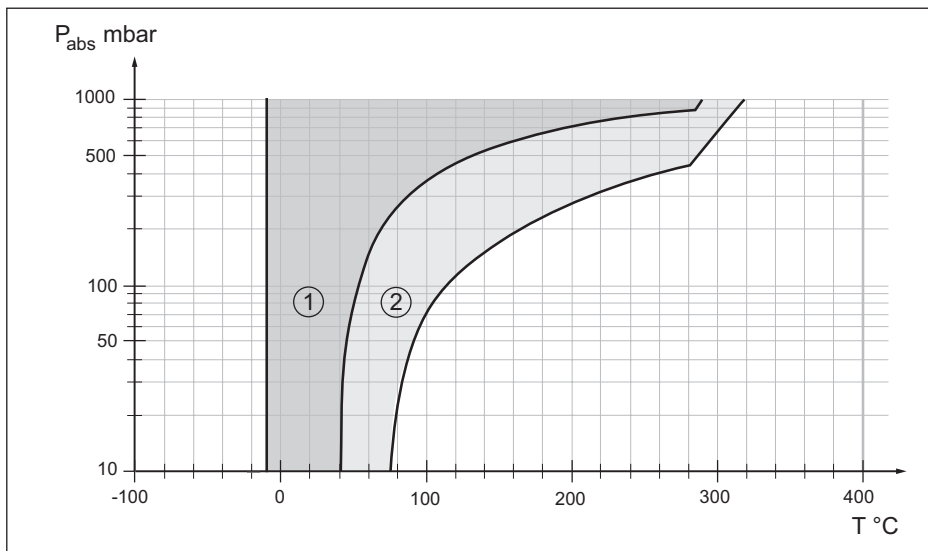
Fig. 41: Toepassingsgebied voor hogetemperatuurolie VE 32, KN 32
