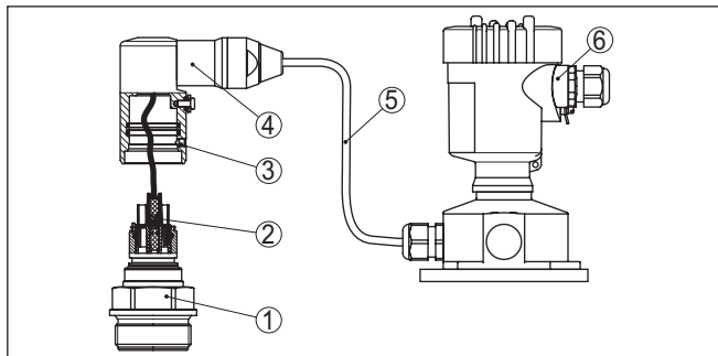
Fig. 36: VEGABAR 81 in IP 68-uitvoering 25 bar en kabeluitgang aan de zijkant, externe behuizing
