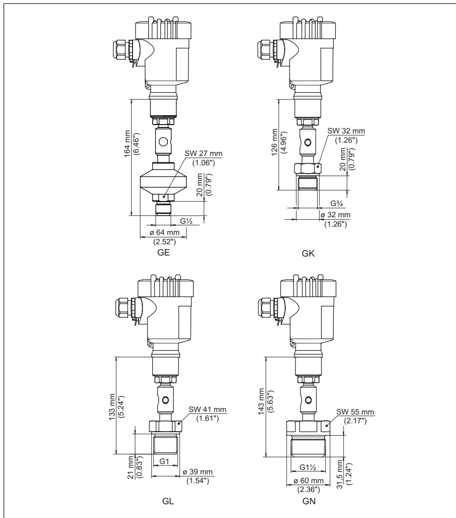
Fig. 52: VEGABAR 81, schroefdraadaansluiting
