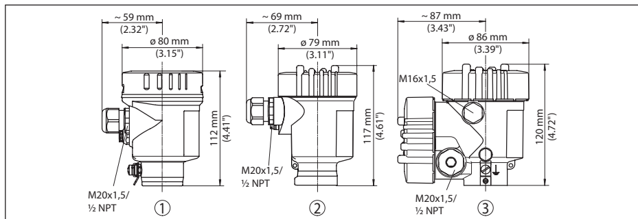
Fig. 48: Huisuitvoeringen in beschermingsklasse IP66/IP68, (0,2 bar), (met ingebouwde display- en bedieningsmodule wordt het huis 9 mm/0.35 in resp. 18 mm/0.71 in hoger)
