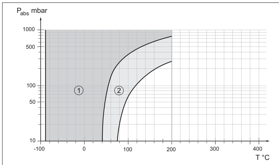
Fig. 40: Toepassingsgebied voor siliconen olie KN 17
