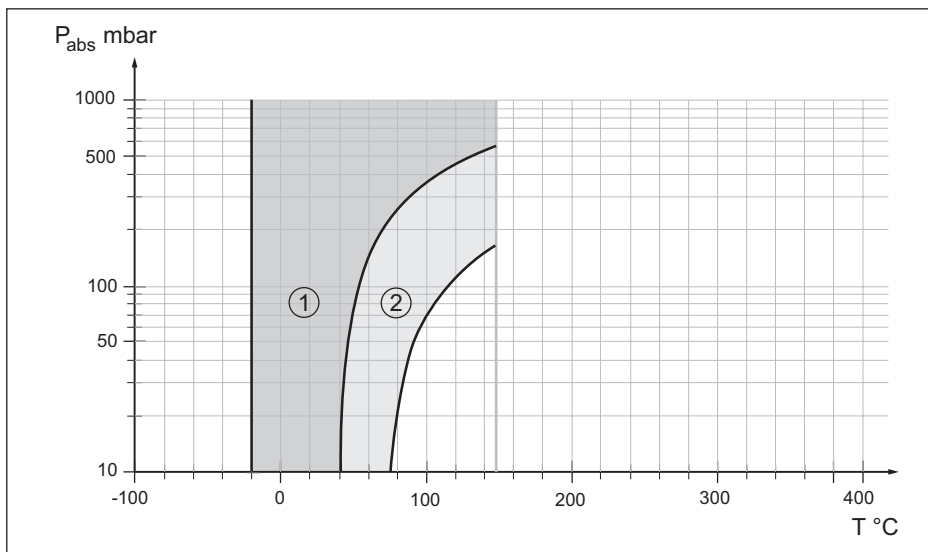
Fig. 44: Toepassingsgebied voor Neobee M-20 KN 59
