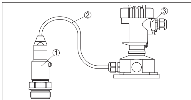
Abb. 20: VEGABAR 81 in IP68-Ausführung 25 bar mit axialem Kabelabgang, externes Gehäuse
