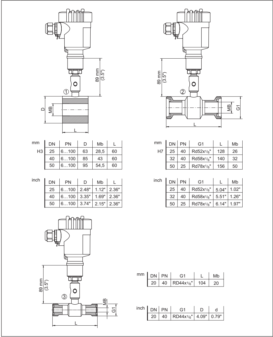
Abb. 42: VEGABAR 81, Rohrdruckmittler
