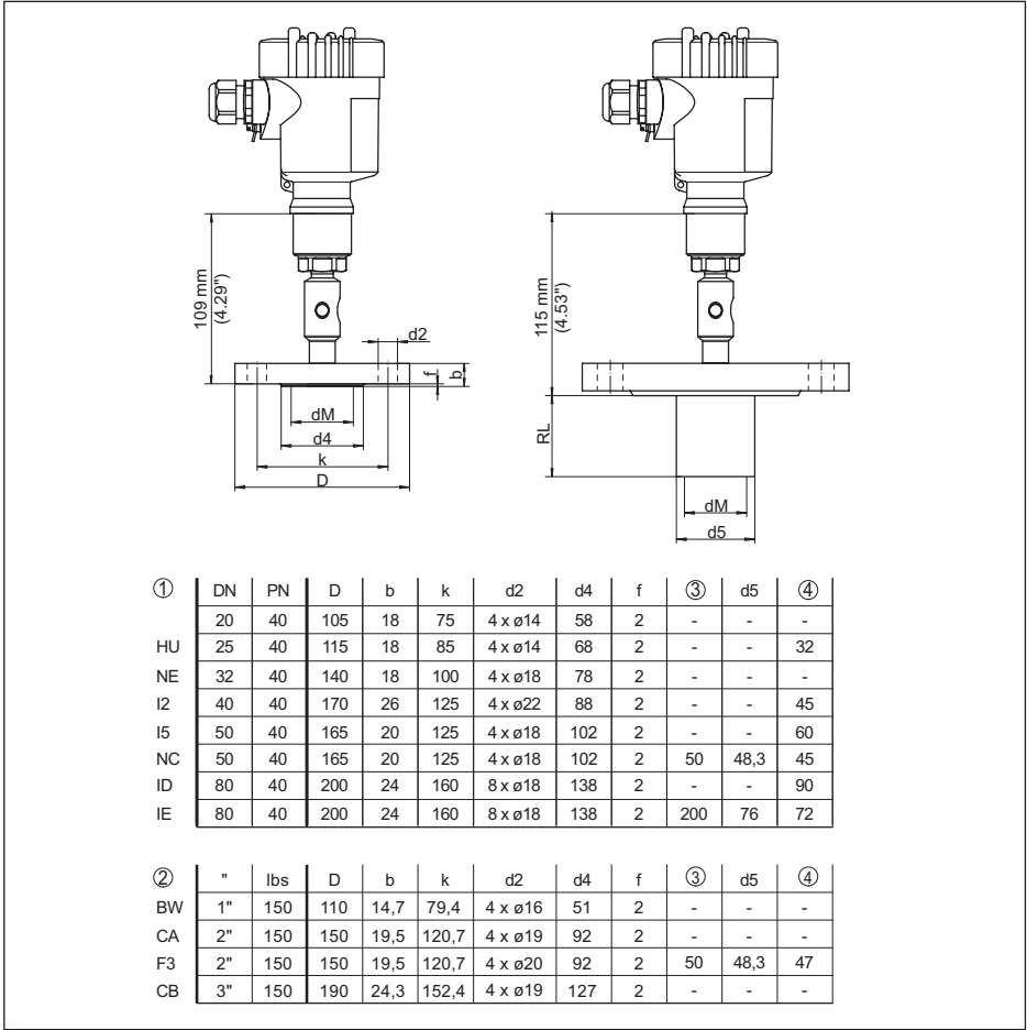
Abb. 43: VEGABAR 81, Flanschsanschluss, Maße in mm
