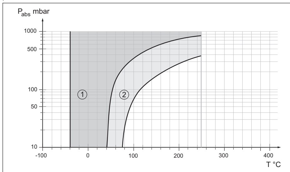
Figura 34: Campo d'impiego per olio siliconico VE 2.2, KN 2.2
