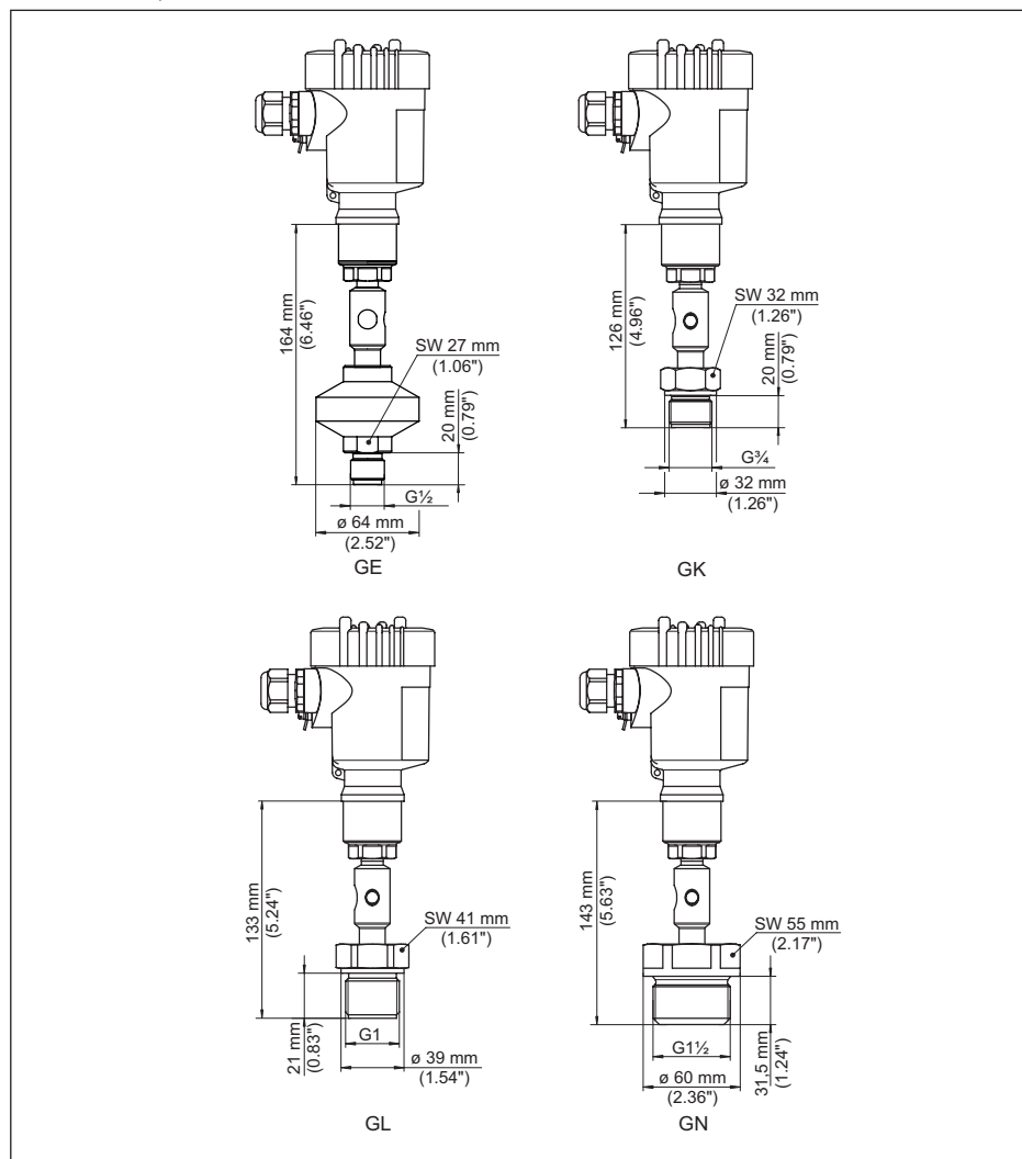
Figura 42: VEGABAR 81, attacco filettato
