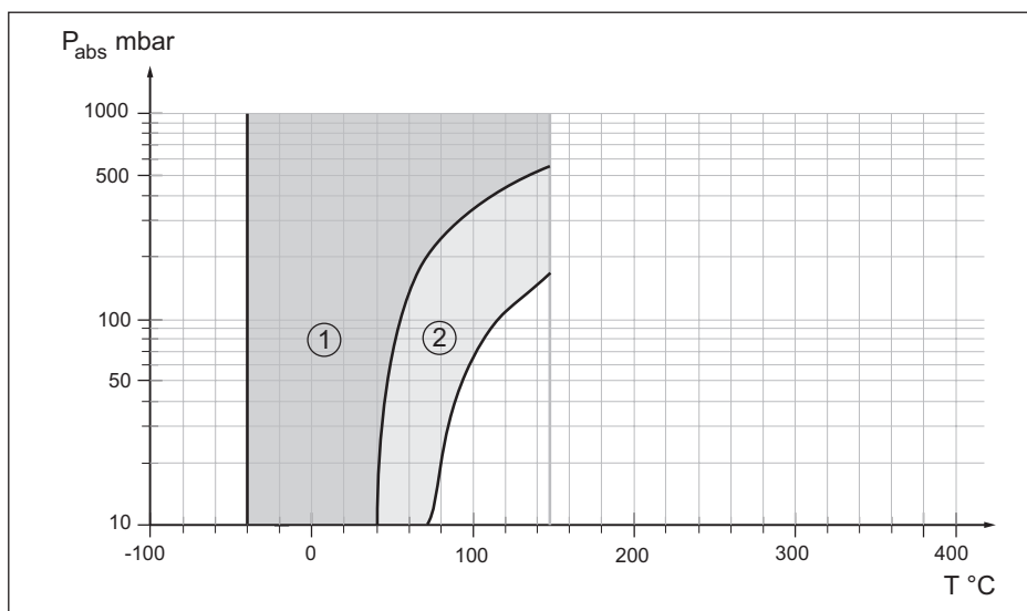
Figura 37: Campo d'impiego per olio Halocarbon KN 21
