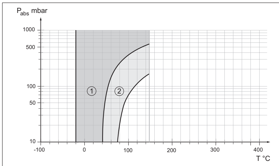
Figura 39: Campo d'impiego per Neobee M-20 KN 59
