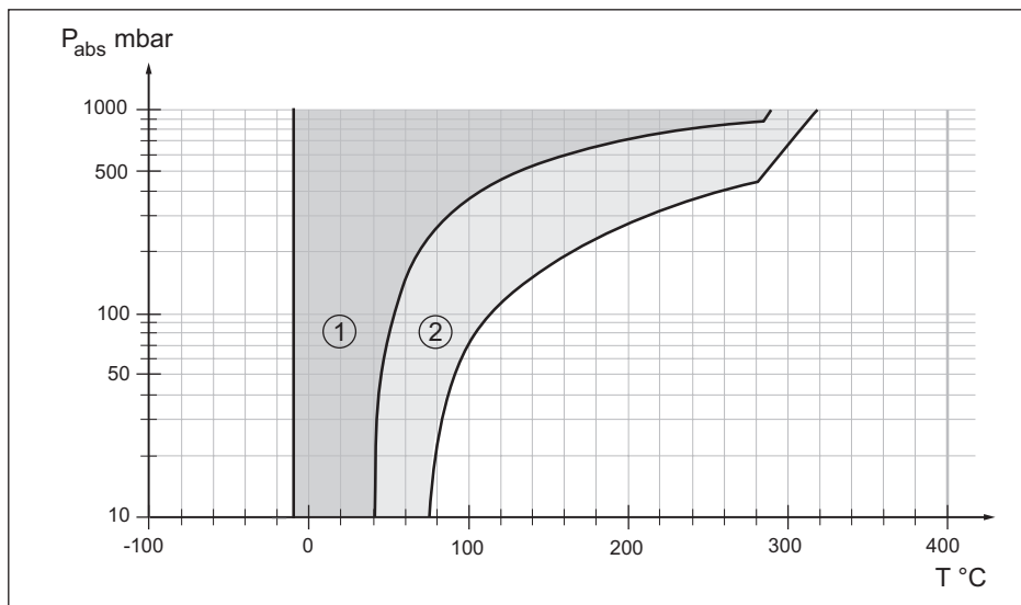
Figura 36: Campo d'impiego per olio per temperature elevate VE 32, KN 32
