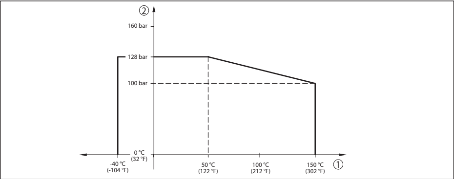
Figura 33: Derating termico VEGABAR 81, attacchi di processo lega 400 (2.4360)
