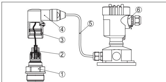
Figura 30: VEGABAR 81 in esecuzione IP68 25 bar e uscita del cavo laterale, custodia esterna
