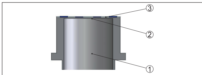
Figura 6: Struttura di un sistema di misura con elemento sensore DMS
