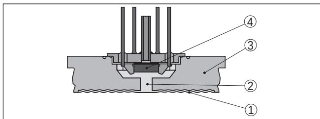
Figura 5: Struttura di un sistema di misura con cella di misura piezoresistiva
