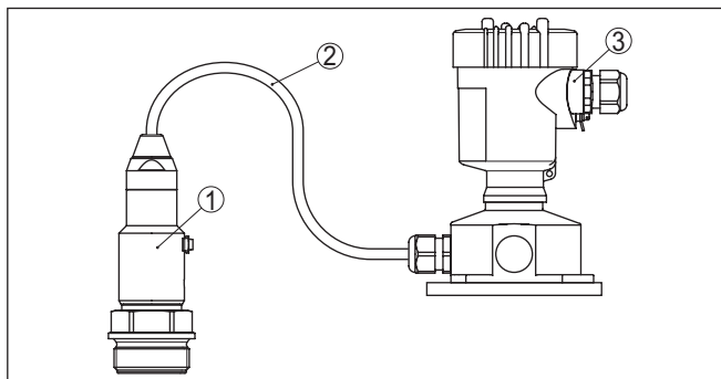
Figura 20: VEGABAR 81 in esecuzione IP68 25 bar con uscita del cavo assiale, custodia esterna
