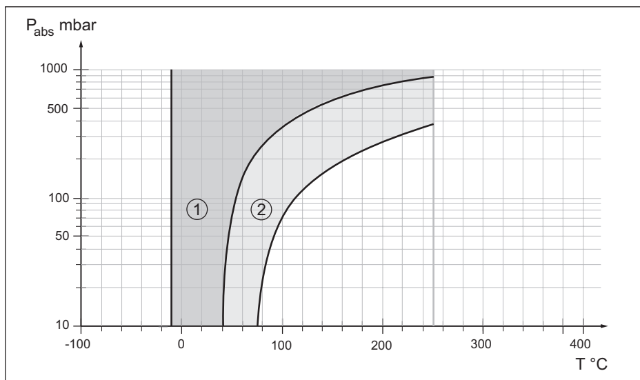
Figura 38: Campo d'impiego per olio bianco medicinale KN 92
