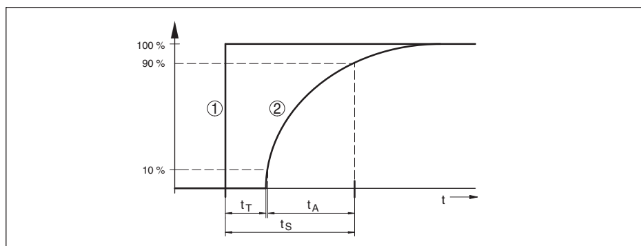
Figura 31: Brusca variazione della grandezza di processo. t_T : tempo morto; t_A : tempo di salita; t_S : tempo di risposta del salto
