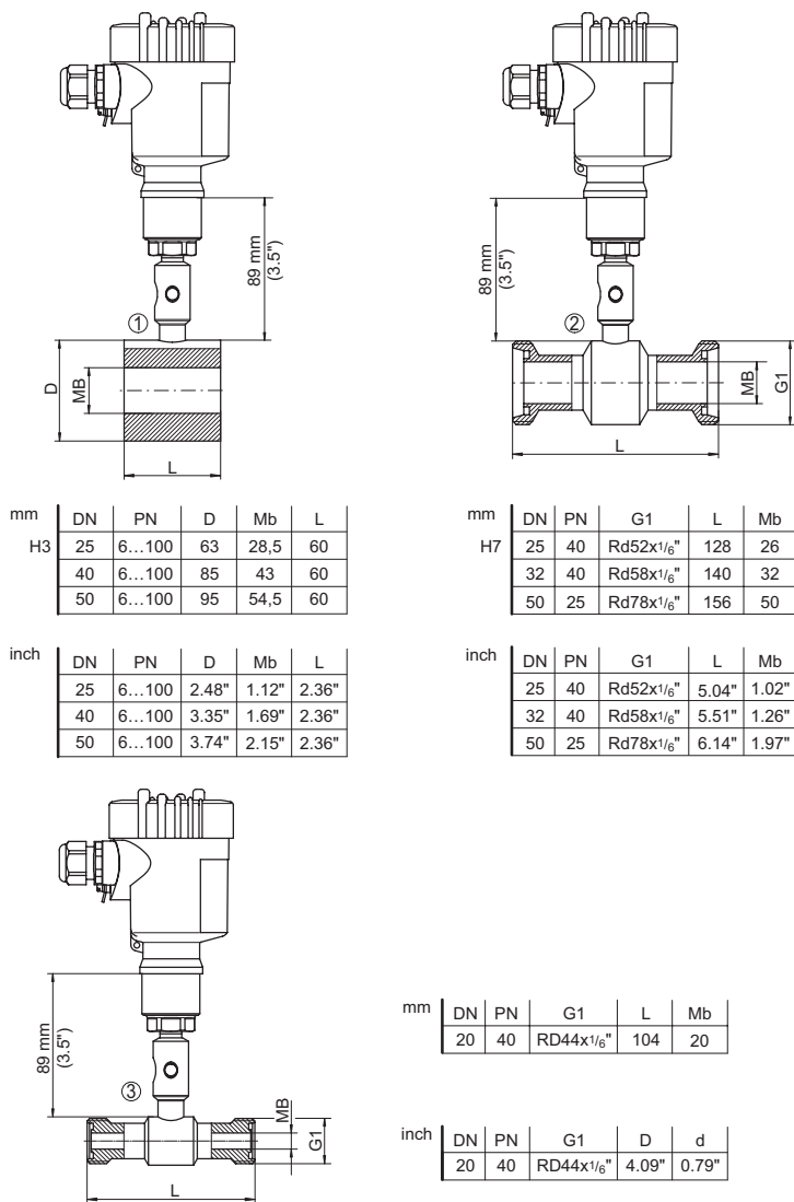
Figura 43: VEGABAR 81- Sistema di separazione su tubo
