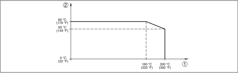
插图: 39: 温度的降低额度 VEGABAR 83 , 至 +200 °C (+392 °F) 的型式
