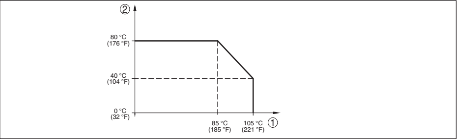
插图. 35: 温度的降低额度 VEGABAR 83 , 至 +105 °C (+221 °F) 的型式
