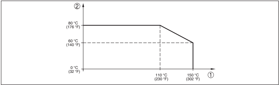
插图 37: 温度的降低额度 VEGABAR 83 , 至 +150 °C (+302 °F) 的型式
