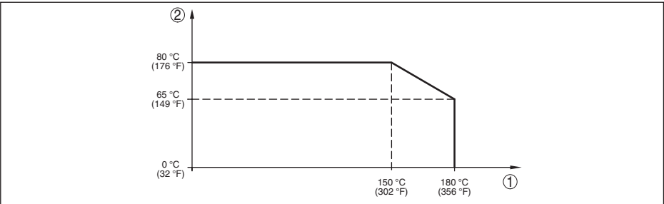
插图: 38: 温度的降低额度 VEGABAR 83 , 至 +180 °C (+356 °F) 的型式
