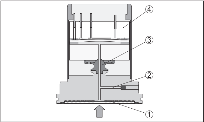
插图. 6: METEC®测量元件的结构
