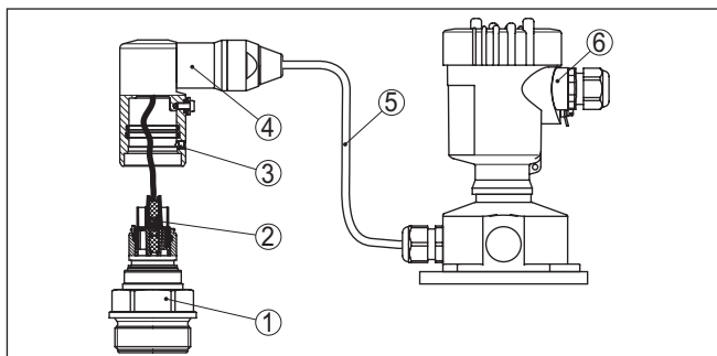
插图. 30: IP68 型 VEGABAR 83, 25 bar 及侧面电缆出口, 外部壳体
