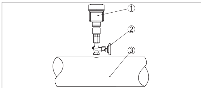
插图. 12: 测量气体的过程压力时在管道中对测量仪表的排布
