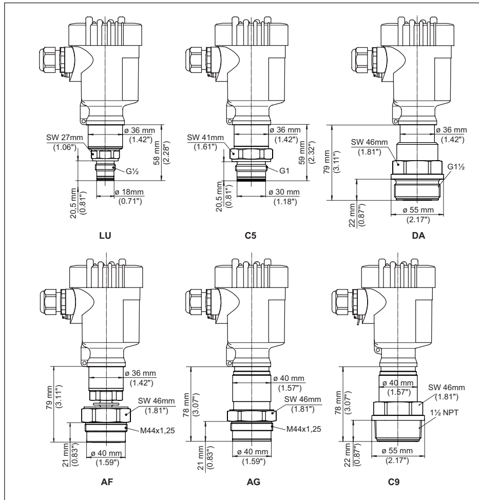
插图. 44: VEGABAR 83, 螺纹接头非正面齐平式
