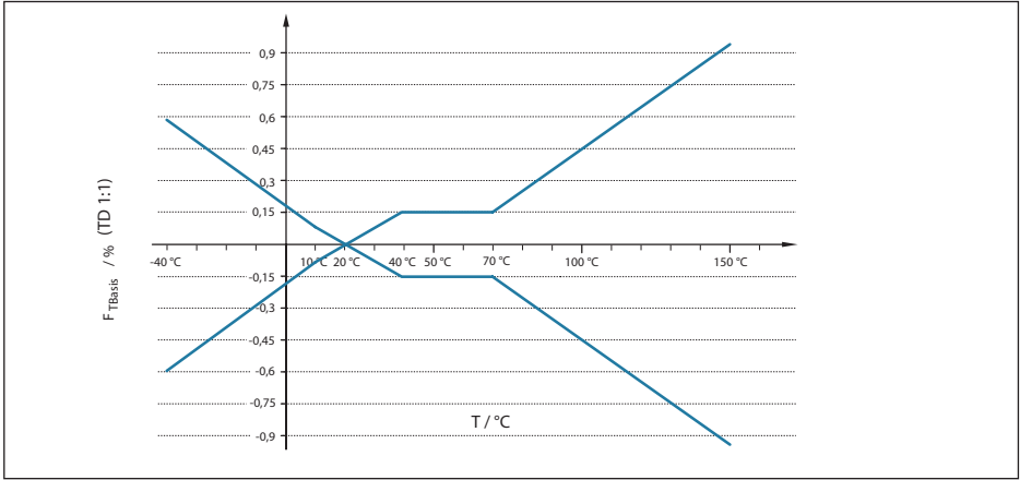
插图. 32: 基本温度错误 F_{TBasis} 当 TD 1 : 1 时
