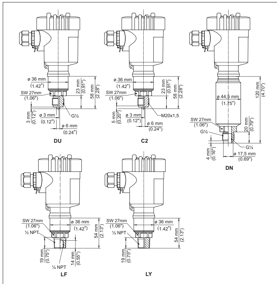
插图. 43: VEGABAR 83, 螺纹, 非正面齐平式
