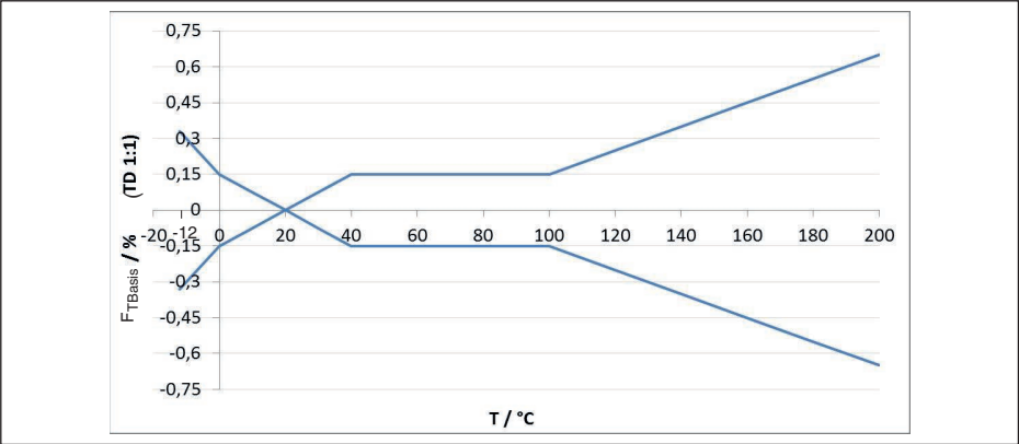
插图. 33: 基本温度错误 F T-Basis 当 TD 1 : 1 时
