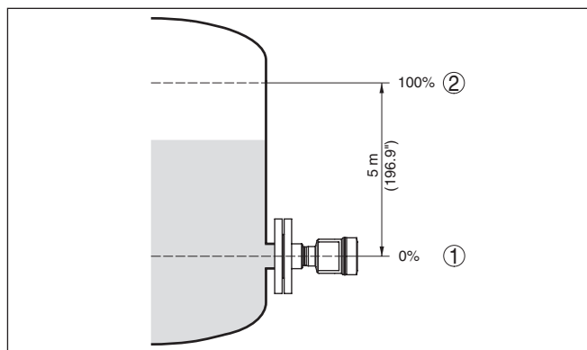
插图. 27: 物位测量时最小/最大调整的参数更改举例
