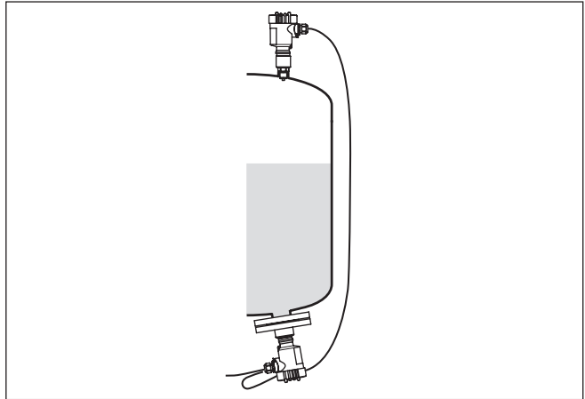
插图. 3: 通过主/从传感器组合来测量电子差压
