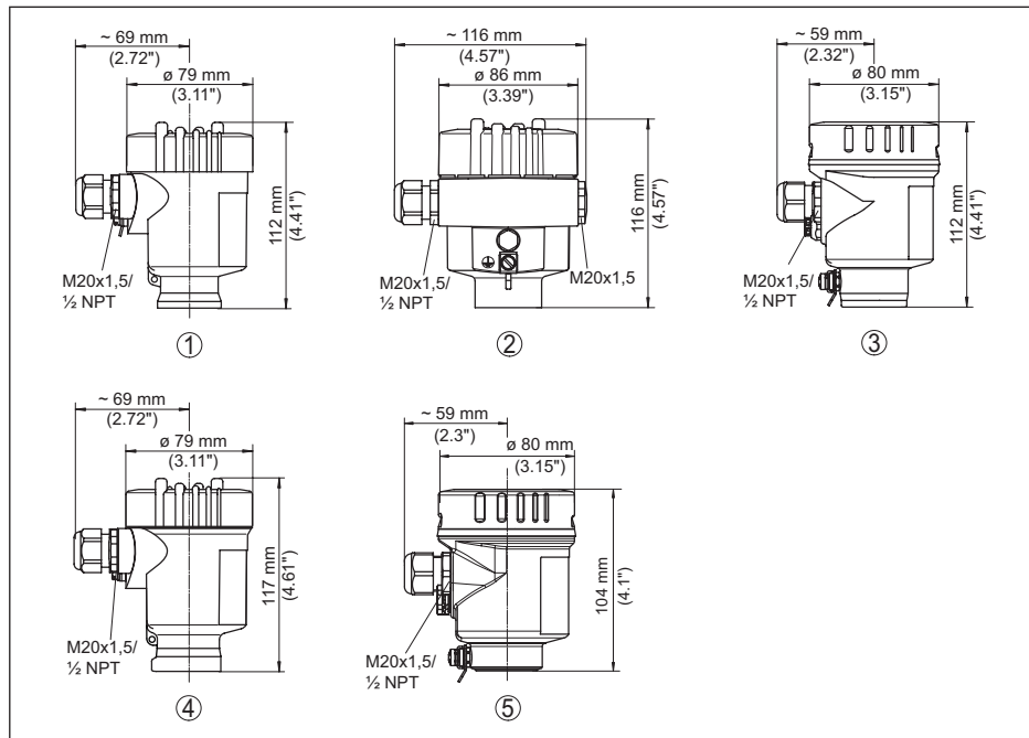
插图. 41: 采用保护等级达 IP66/IP67 和 IP66/IP68 (0.2 bar) 的壳体版本, (内装显示和调整模块后, 壳体高度增加了9 mm/0.35 in 或 18 mm/0.71 in)
