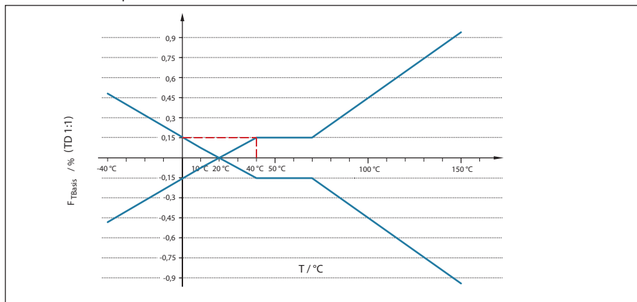
插图. 40: 为上例计算基本温度误差: F_{\text{TBasis}} = \mathbf{0.15 \%}
