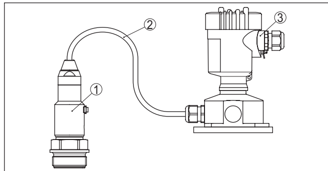
插图. 20: IP68 型 VEGABAR 83，25 bar，带轴向电缆出口，外部壳体
