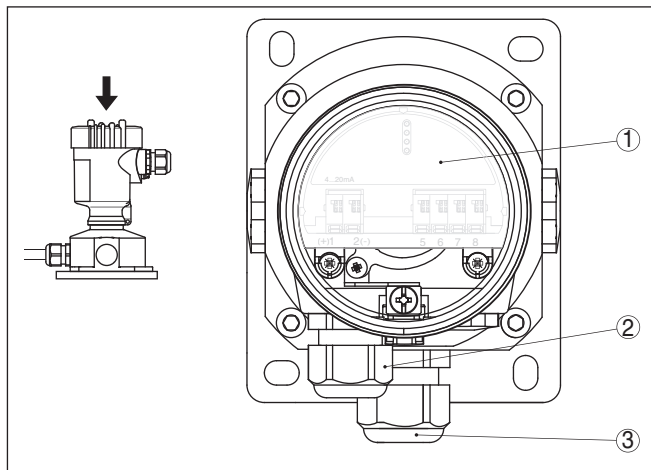
插图. 21: 电子部件腔和接线腔
