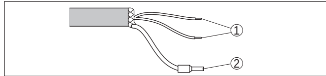
插图. 19: 固定连接电缆的芯线分布
