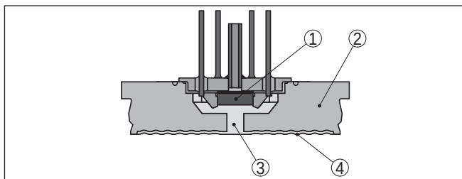
Figura 4: Struttura del sistema di misura con cella di misura piezoresistiva
