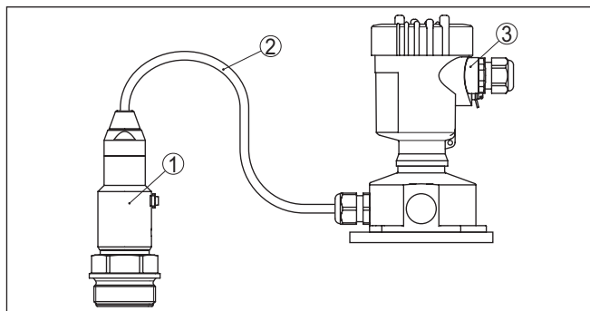
Figura 22: VEGABAR 83 in esecuzione IP68 25 bar con uscita del cavo assiale, custodia esterna
