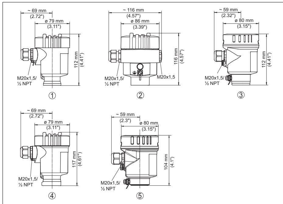
Figura 43: Differenti custodie con grado di protezione IP66/IP67 e IP66/IP68 (0,2 bar), (con tastierino di taratura con display incorporato l'altezza della custodia aumenta di 9 mm/0.35 in ovv. 18 mm/0.71 in)
