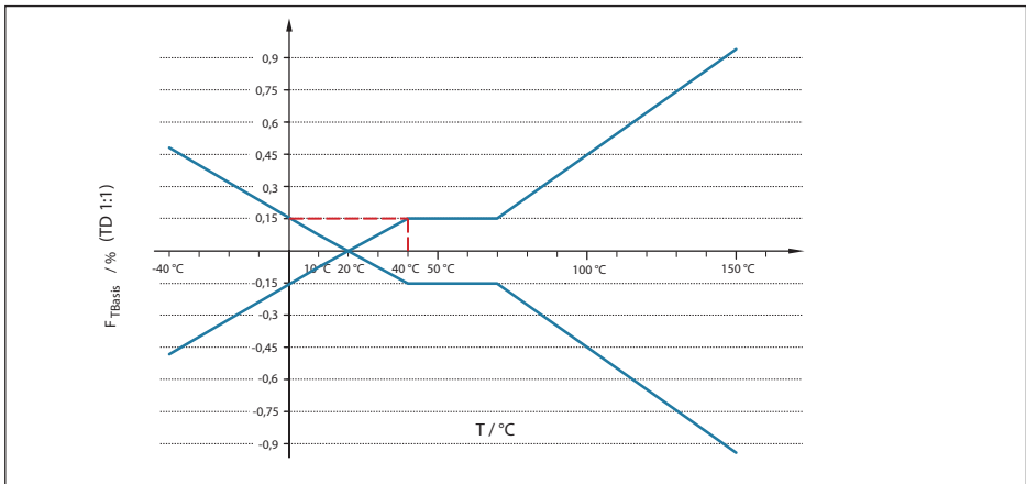
Figura 42: Calcolo dell'errore di temperatura base per il suddetto esempio: F_{TBasis} = 0,15\%
