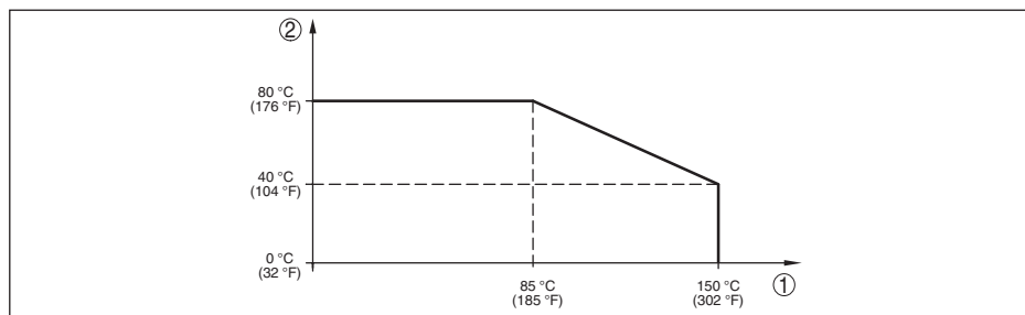
Figura 38: Derating di temperatura VEGABAR 83, esecuzione fino a +150 °C (+302 °F)
