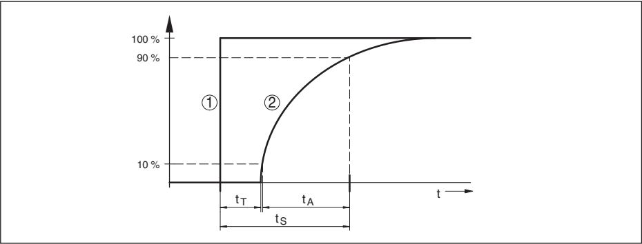
Figura 33: Comportamento in caso di brusca variazione della grandezza di processo. t_T : tempo morto; t_A : tempo di salita; t_S : tempo di risposta del salto
