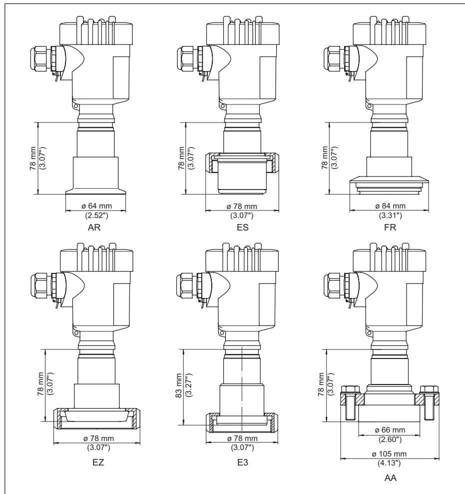
Figura 48: VEGABAR 83, attacco igienico 150 °C (cella di misura METEC®)
