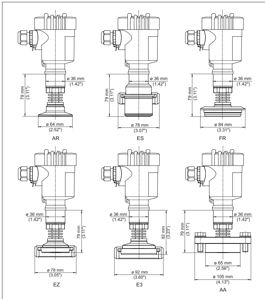
Figura 47: VEGABAR 83, attacco igienico 150 °C (cella di misura piezoresistiva/DMS)
