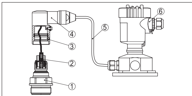
Figura 32: VEGABAR 83 in esecuzione IP68 25 bar e uscita del cavo laterale, custodia esterna
