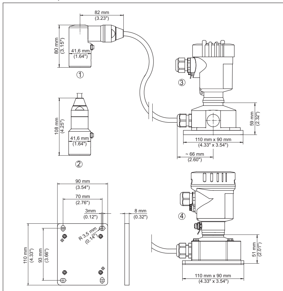
Figura 44: VEGABAR 83, esecuzione IP68 con custodia esterna
