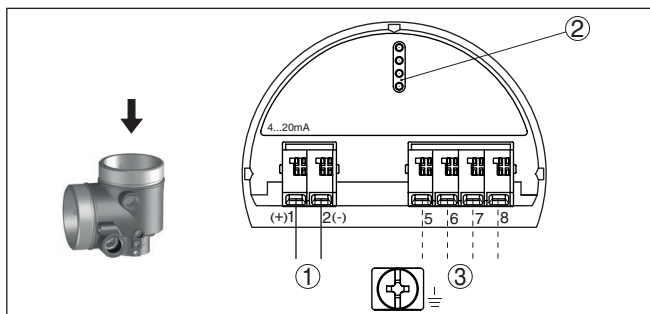
Figura 19: Vano dell'elettronica - custodia a due camere Ex-d-ia
