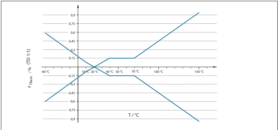
Figura 34: Errore di temperatura base F_{TBasis} con TD 1 : 1
