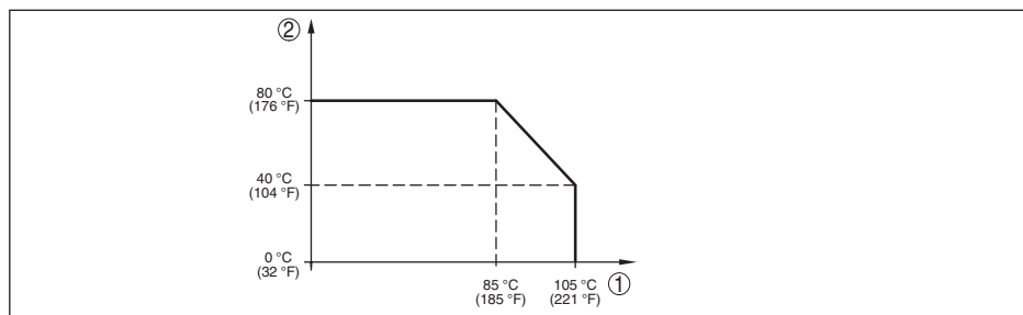
Figura 37: Derating di temperatura VEGABAR 83, esecuzione fino a +105 °C (+221 °F)
