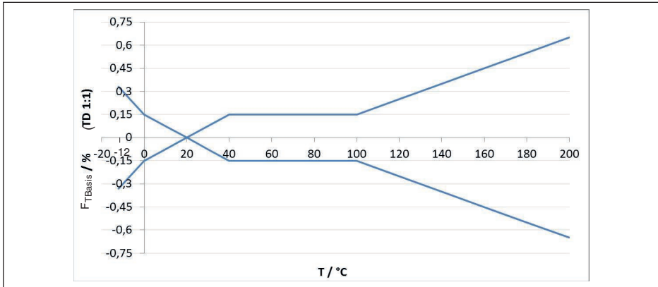
Figura 35: Errore di temperatura base F_{TBasis} con TD 1 : 1
