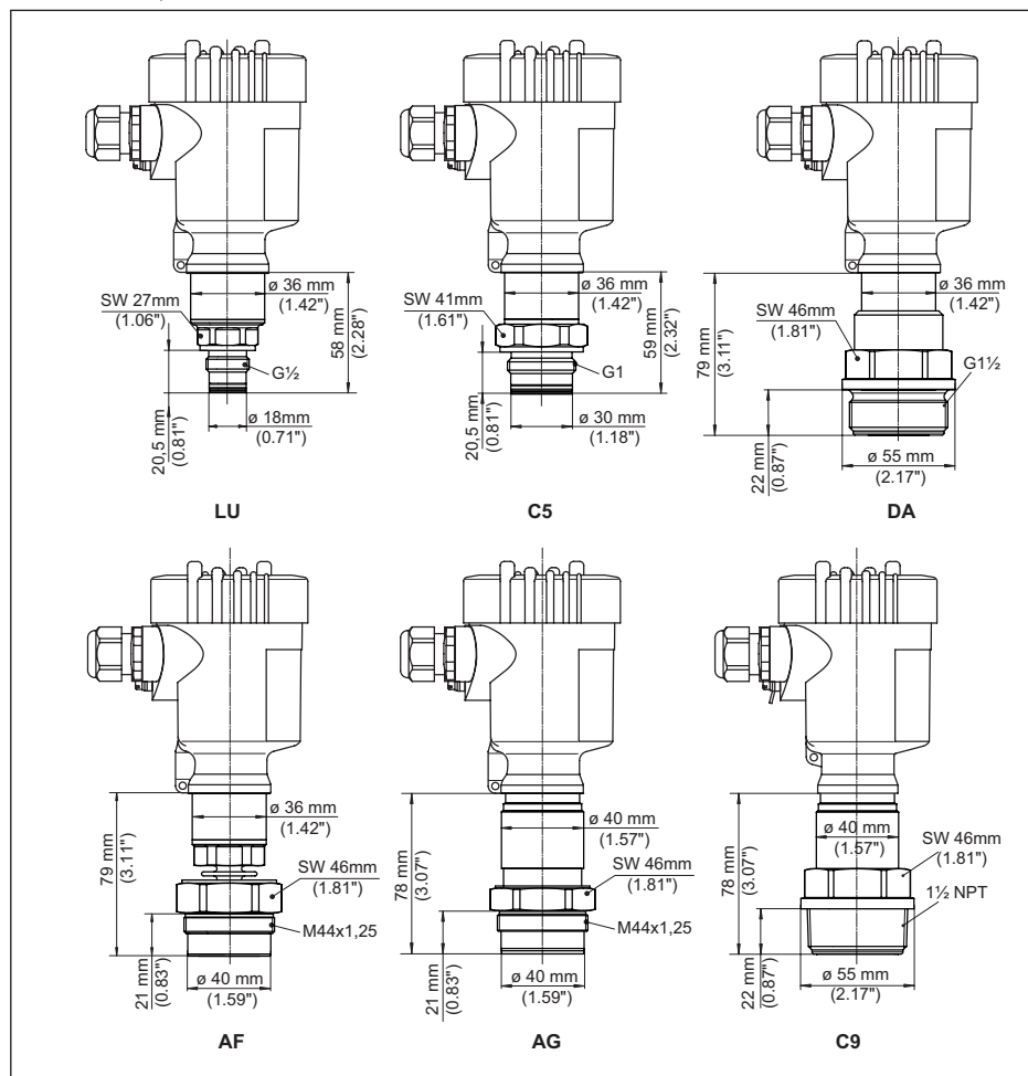
Figura 46: VEGABAR 83, attacco filettato affacciato
