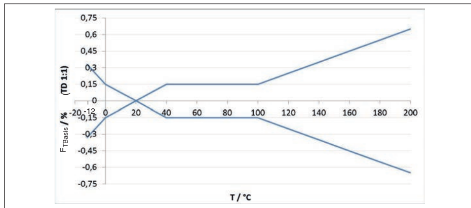
Fig. 35: Basistemperatuurfout F_{TBasis} bij TD 1 : 1
