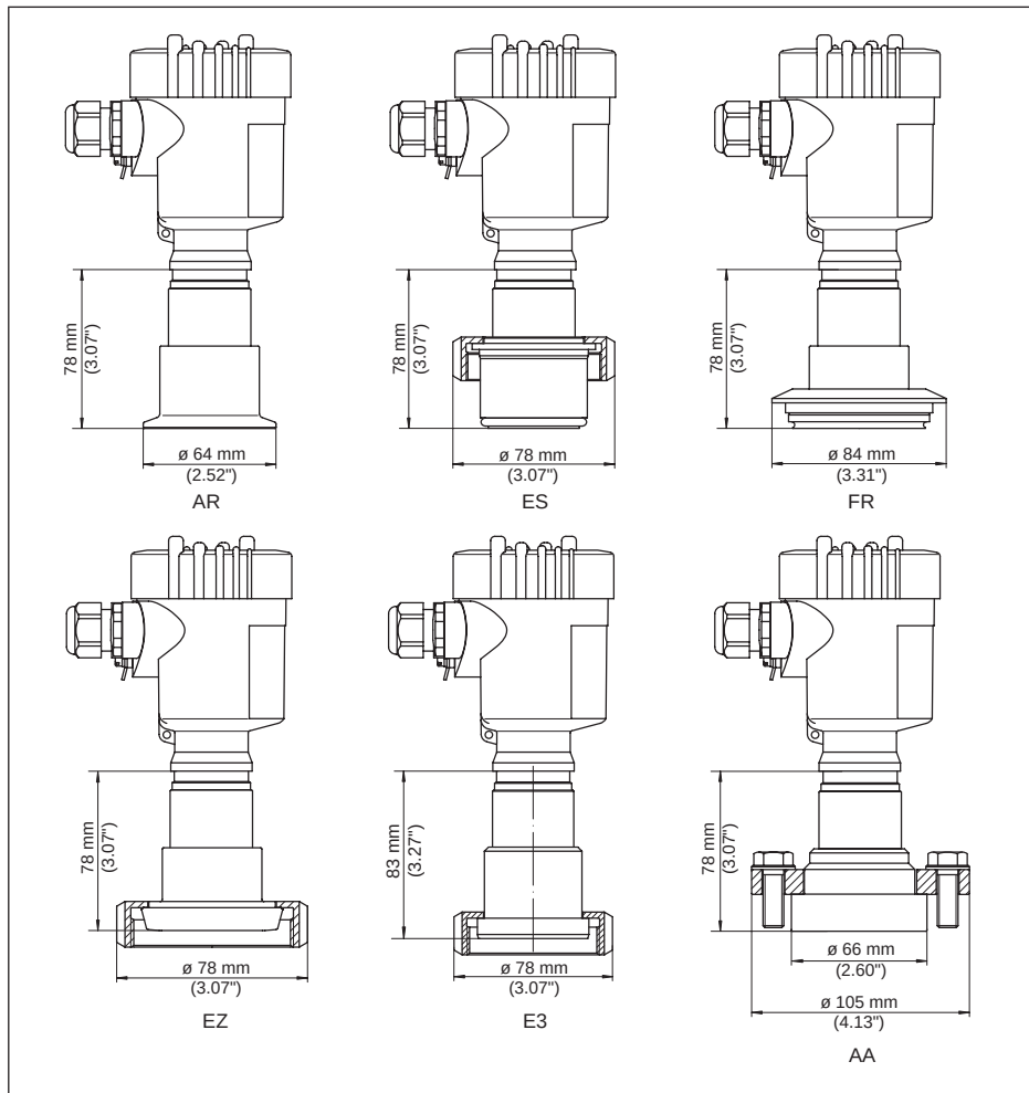
Fig. 48: VEGABAR 83, hygiënische aansluiting 150 °C (METEC®-meetcel)
