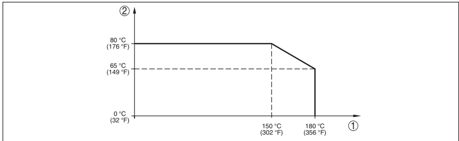
Fig. 37: Redução de temperatura VEGABAR 83, modelo até +180 °C (+356 °F)
