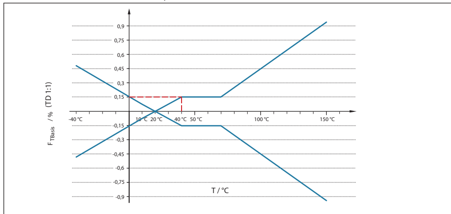
Fig. 39: Cálculo do erro de temperatura básico para o exemplo acima F_{TBasis} = 0,15\% :
