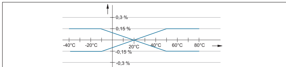
Fig. 33: Alteração térmica da saída de corrente
