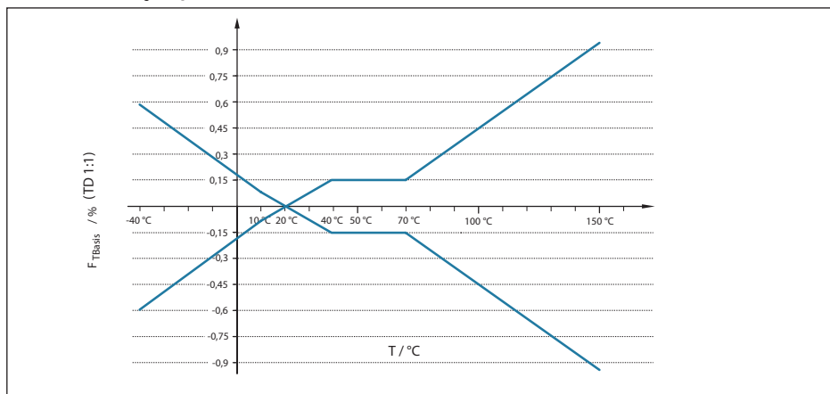
Fig. 31: Erro de temperatura básico F_{TBasic} com TD 1 : 1
