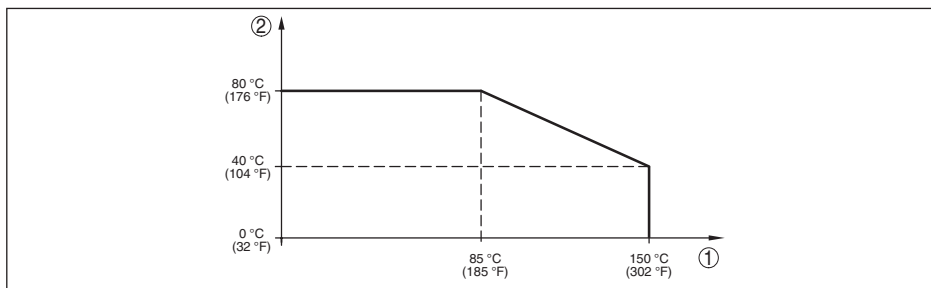
Fig. 35: Redução de temperatura VEGABAR 83, modelo até +150 °C (+302 °F)
