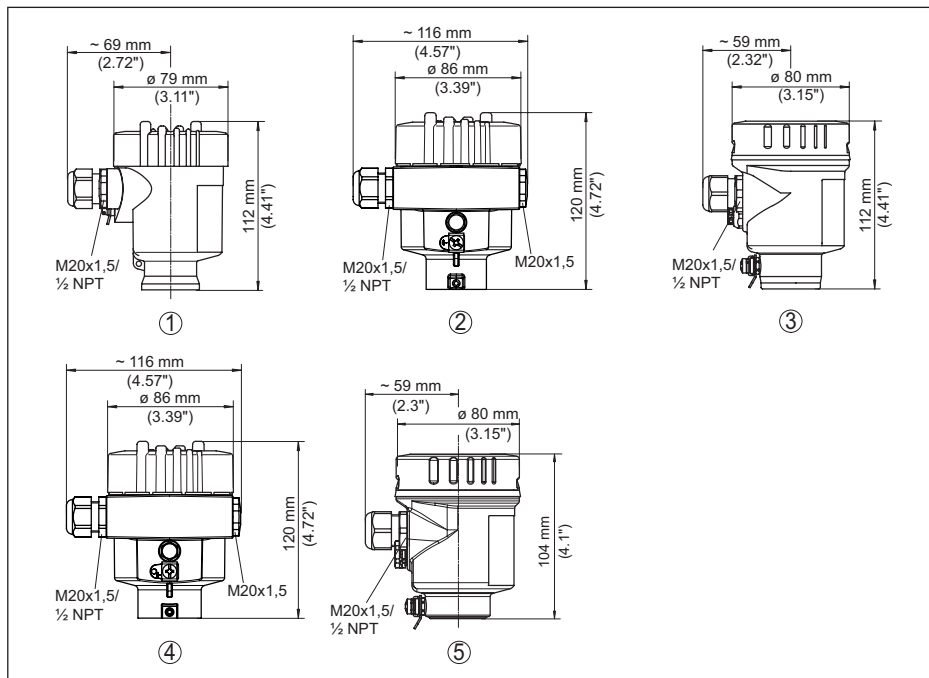
Fig. 40: Variantes da caixa com grau de proteção IP66/IP67 und IP66/IP68 (0,2 bar), (com o módulo de visualização e configuração montado, a altura da caixa é aumentada em 9 mm/0.35 in bzw. 18 mm/0.71 in)
