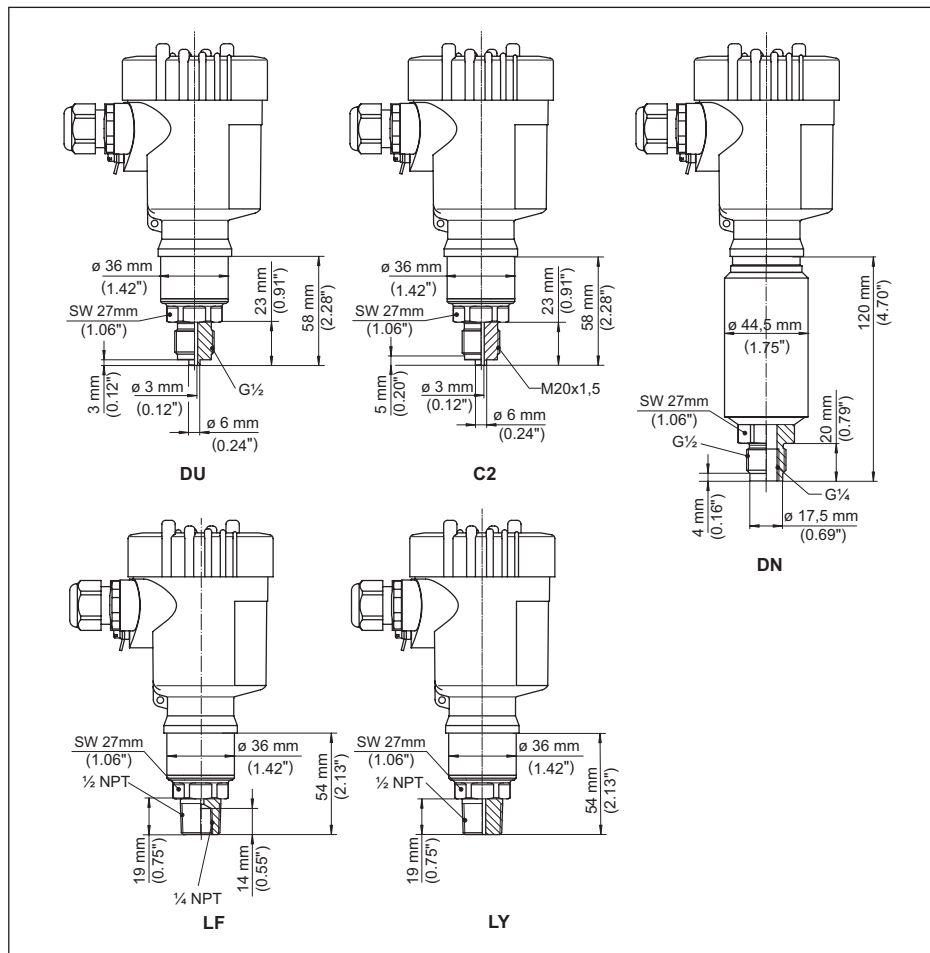
Fig. 42: VEGABAR 83, conexão rosca não embutida na frente
