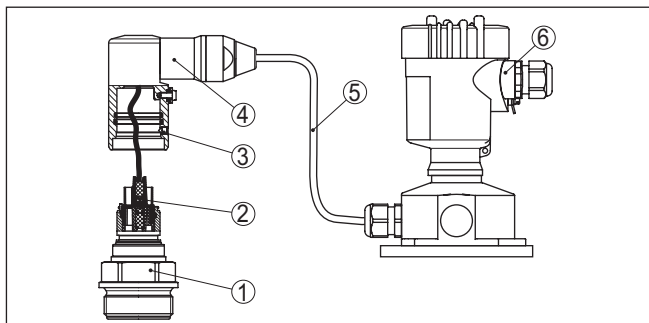
Fig. 36: VEGABAR 83 in IP 68-uitvoering 25 bar en kabeluitgang aan de zijkant, externe behuizing
