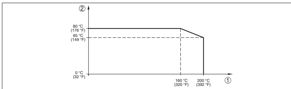
Fig. 44: Temperatuur-derating VEGABAR 83, uitvoering tot +200 °C (+392 °F)
