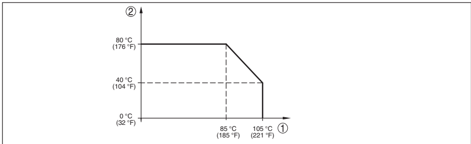
Fig. 40: Temperatuurderating VEGABAR 83, uitvoering tot +105 °C (+221 °F)
