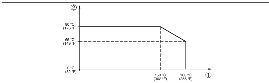
Fig. 43: Temperatuur-derating VEGABAR 83, uitvoering tot +180 °C (+356 °F)
