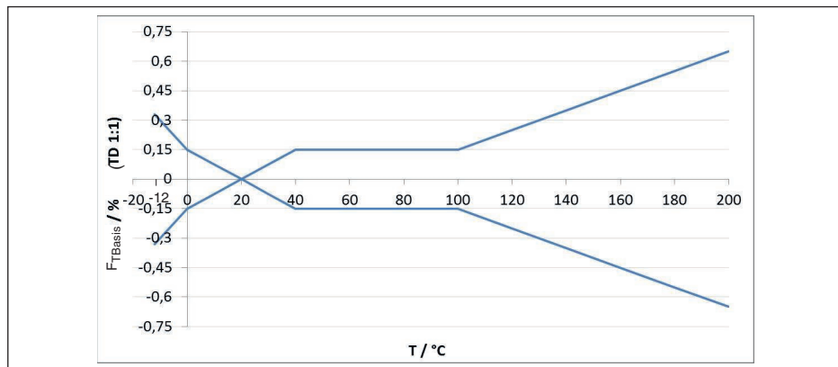
Fig. 39: Basistemperatuurfout F_{TBasis} bij TD 1 : 1
