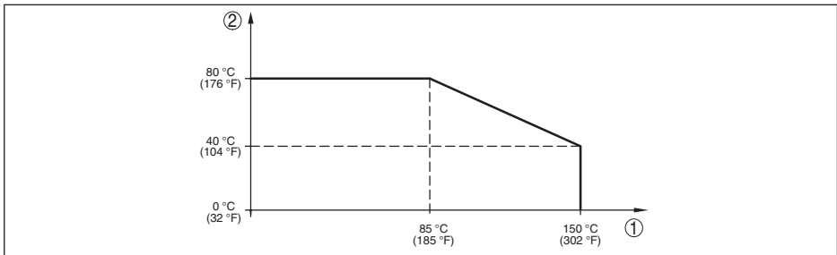
Fig. 41: Temperatuurderating VEGABAR 83, uitvoering tot +150 °C (+302 °F)
