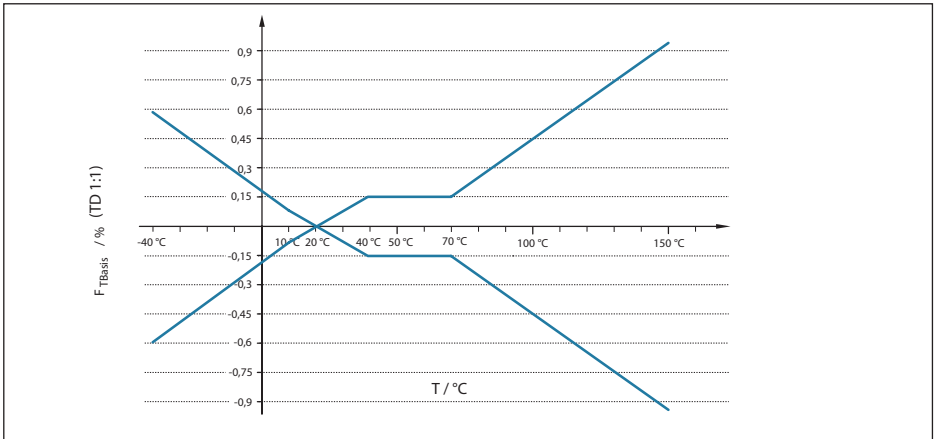
Fig. 38: Basistemperatuurfout F_{TBasis} bij TD 1 : 1
