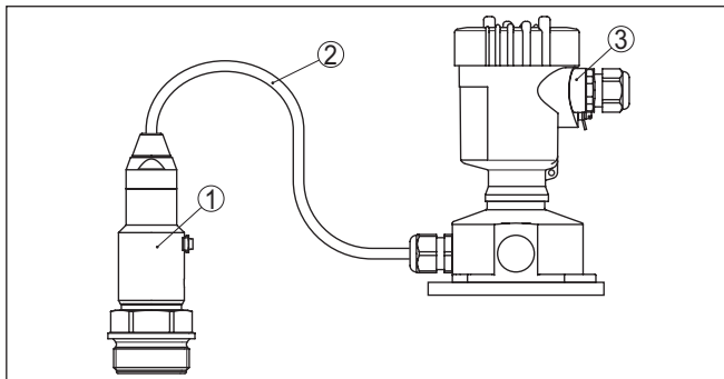
Fig. 24: VEGABAR 83 in IP68-uitvoering 25 bar met axiale kabeluitgang, externe behuizing
