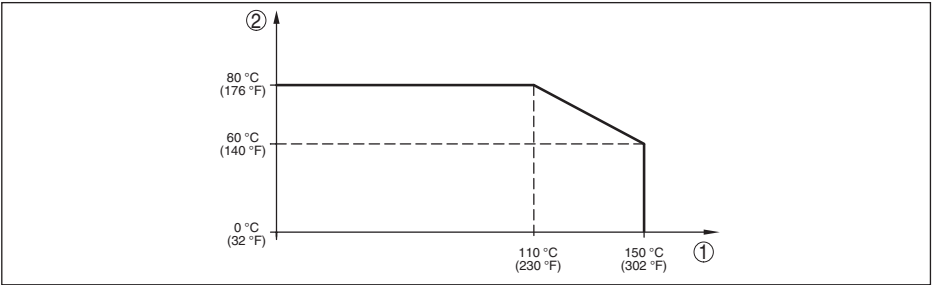
Fig. 42: Temperatuur-derating VEGABAR 83, uitvoering tot +150 °C (+302 °F)
