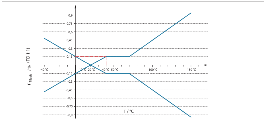
Fig. 45: Bepaling van de basistemperatuurfout voor het voorbeeld boven: F_{TBasis} = 0,15 \%
