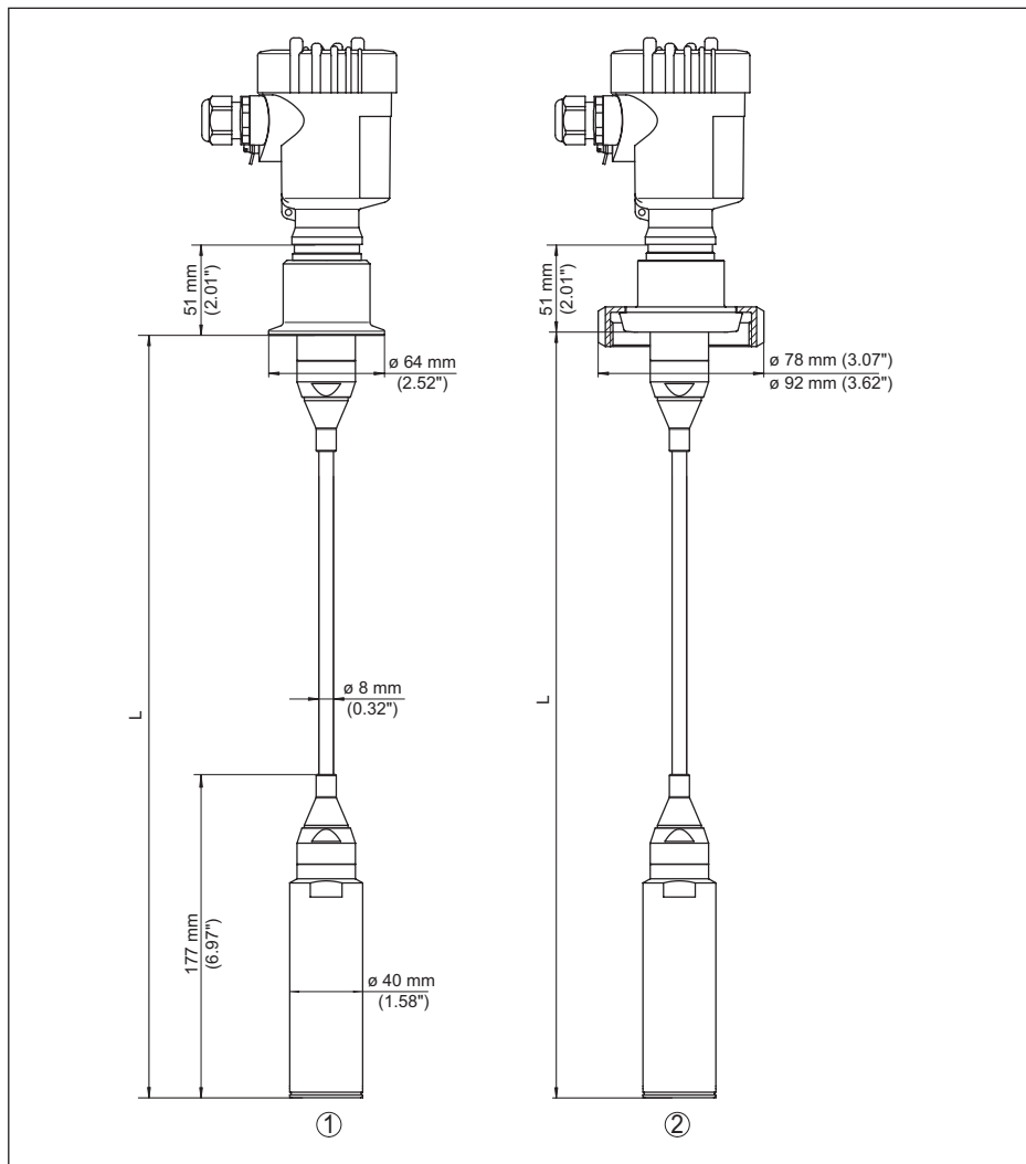
Figura 50: VEGABAR 87, attacchi aseptici
