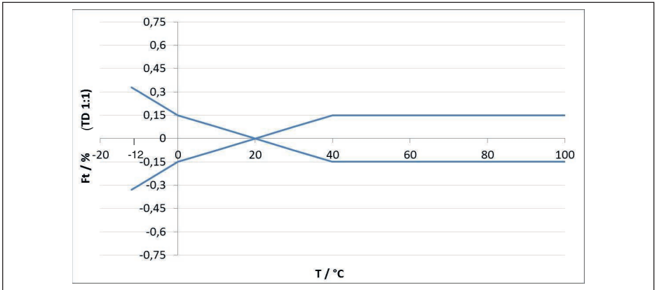
Figura 38: Errore di temperatura base F_{TBasis} con TD 1 : 1
