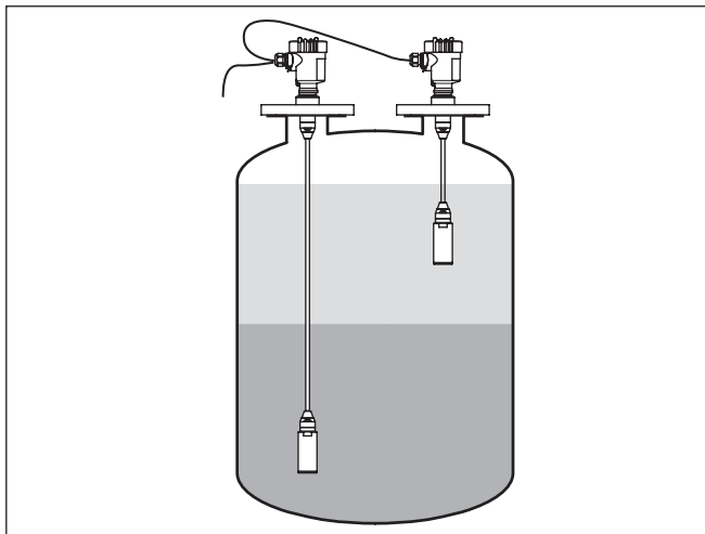
Figura 3: Misura elettronica di pressione differenziale tramite una combinazione primary/secondary
