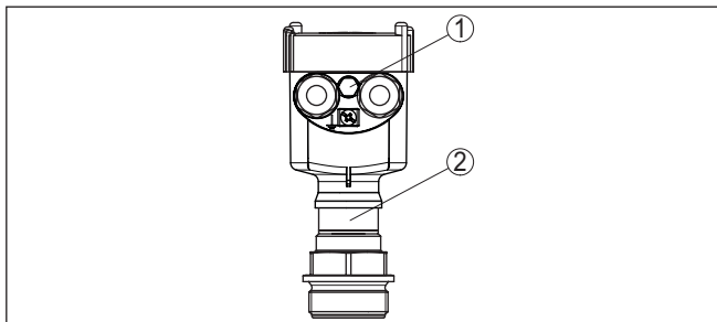
Fig. 6: Positie van het filterelement - gasdichte doorvoer
