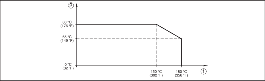
Fig. 29: Temperatuur-derating VEGABAR 83, uitvoering tot +180 °C (+356 °F)
