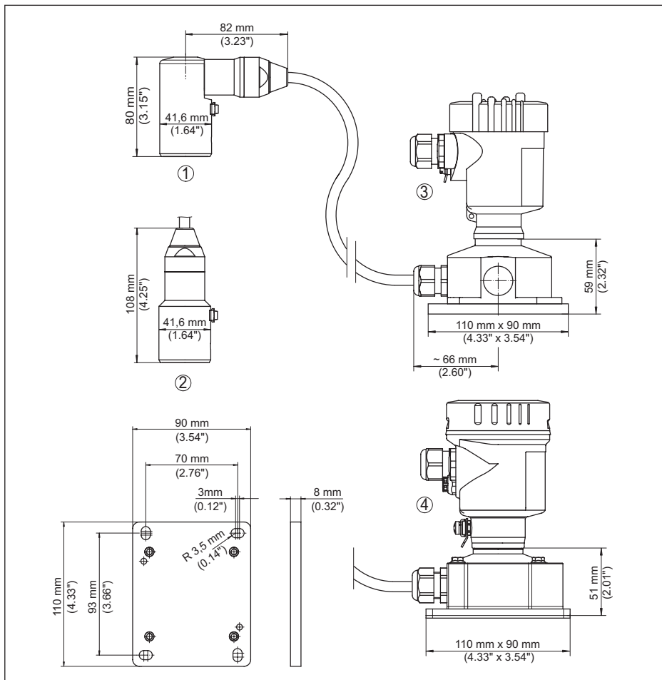
Fig. 34: VEGABAR 83, IP68-uitvoering met externe behuizing
