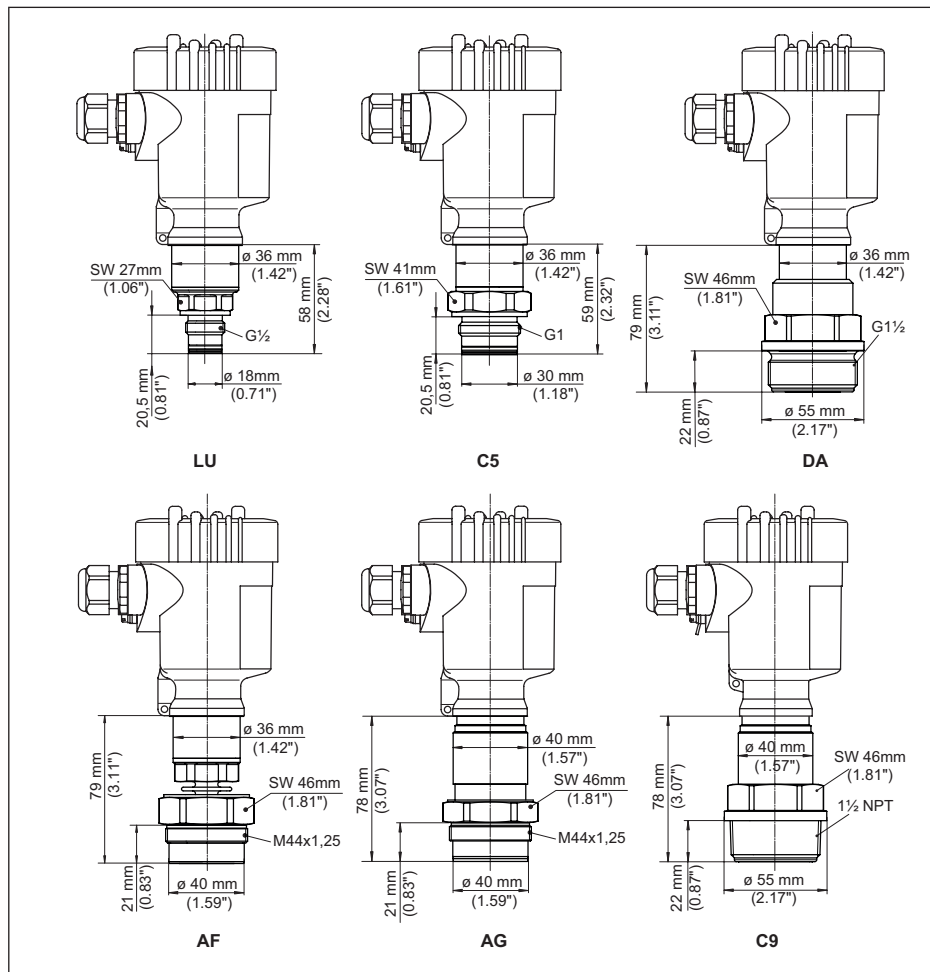
Fig. 36: VEGABAR 83, schroefdraadaansluiting vlak
