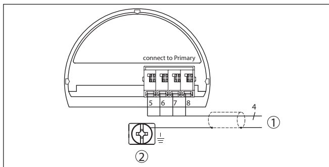
Fig. 19: Aansluitschema VEGABAR 83 secondary device
