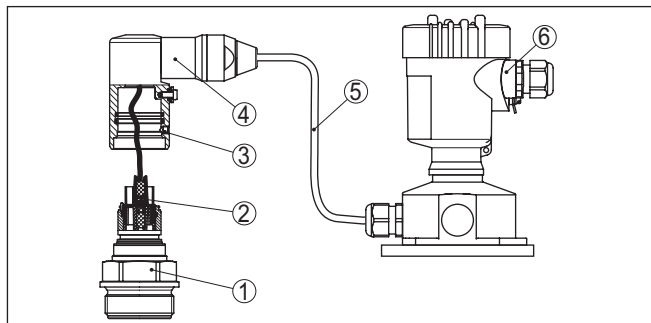
Fig. 22: VEGABAR 83 in IP 68-uitvoering 25 bar en kabeluitgang aan de zijkant, externe behuizing
