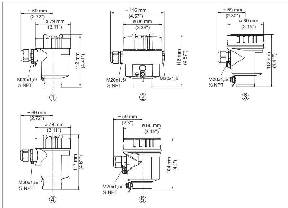
Fig. 33: Huisuitvoeringen in beschermingsklasse IP66/IP67 en IP66/IP68 (0,2 bar), (met ingebouwde display- en bedieningsmodule wordt het huis 9 mm/0.35 in resp. 18 mm hoger)
