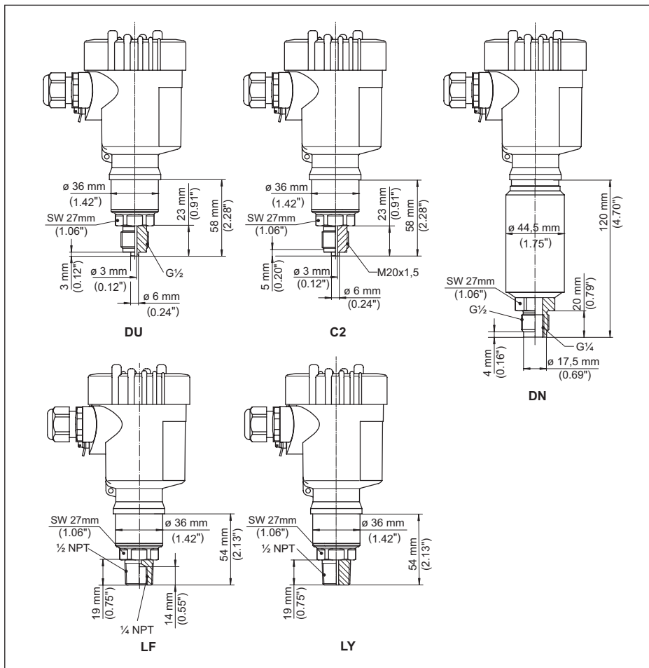
Fig. 35: VEGABAR 83, schroefdraadaansluiting niet vlak
