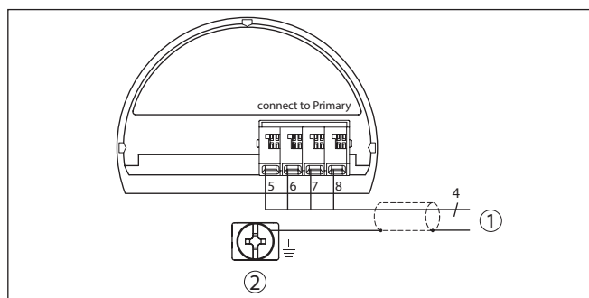
Fig. 15: Aansluitschema VEGABAR 83 secondary device
