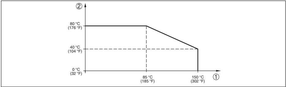
Fig. 27: Temperatuur-derating VEGABAR 83, uitvoering tot +150 °C (+302 °F)
