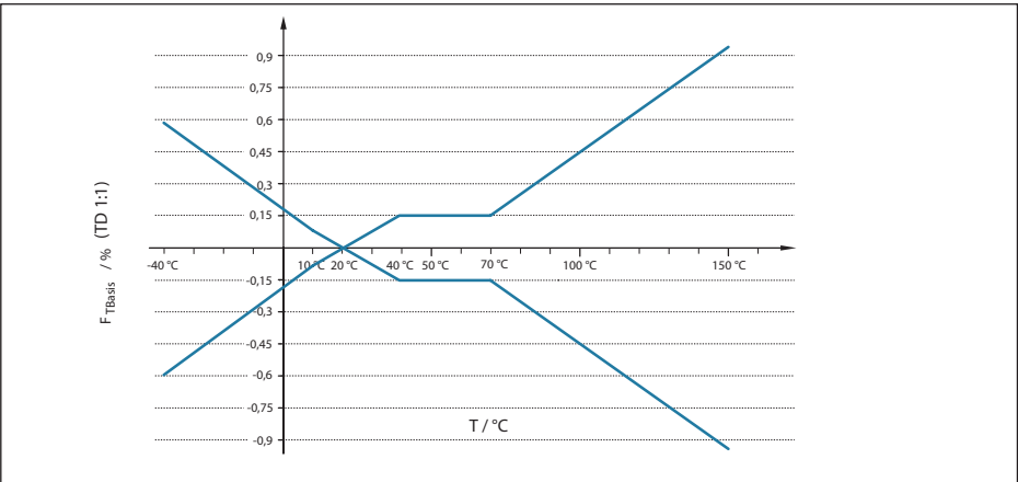
Fig. 24: Basistemperatuurfout F_{TBasis} bij TD 1 : 1
