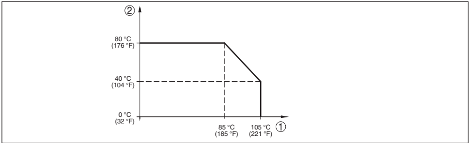
Fig. 26: Temperatuur-derating VEGABAR 83, uitvoering tot +105 °C (+221 °F)
