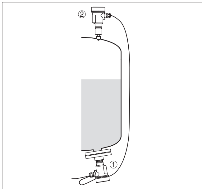
Fig. 8: Meetopstelling bij niveaumeting in tanks onder druk
