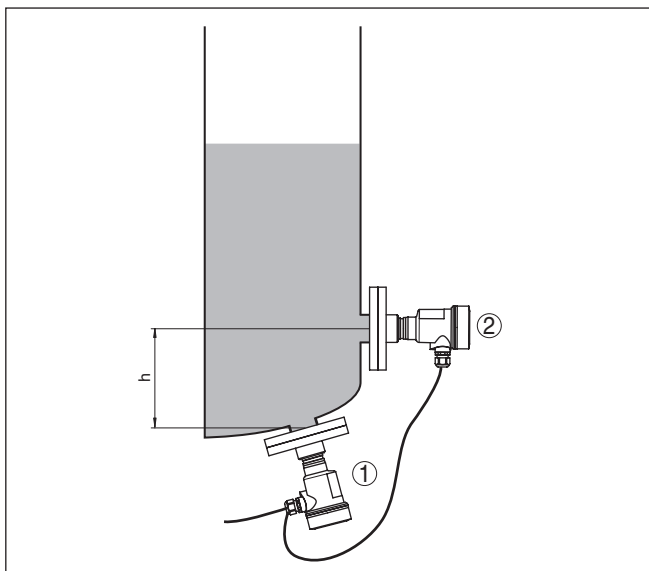
Fig. 12: Meetopstelling bij dichtheidsgecompenseerde niveaumeting, h = afstand tussen de beide meetpunten.
