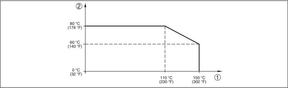
Fig. 28: Temperatuur-derating VEGABAR 83, uitvoering tot +150 °C (+302 °F)
