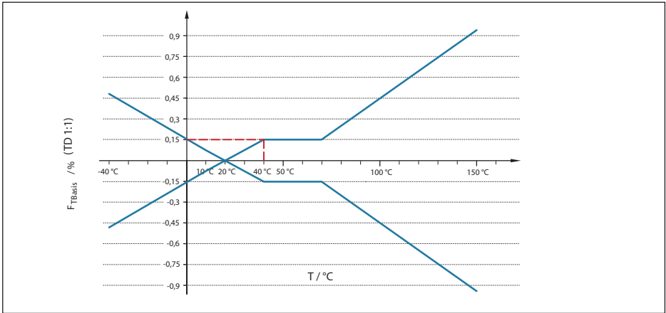
Fig. 31: Bepaling van de basistemperatuurfout voor het voorbeeld boven: F_{TBasis} = 0,15\%
