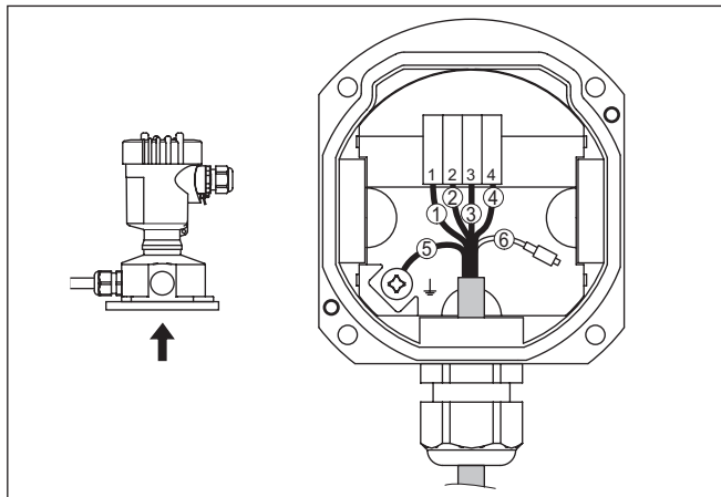
Fig. 18: Aansluiting van de procesmodule in de behuizingssokkel
