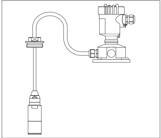
Abb. 15: VEGABAR 86 in IP68-Ausführung 25 bar, nicht-Ex und axialem Kabelabgang, externes Gehäuse
