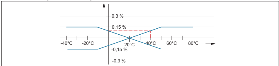
Abb. 25: F_a durch Thermische Änderung Stromausgang, in diesem Beispiel = \mathbf{0,1 \%}
