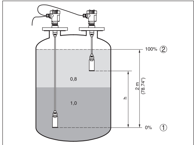
Abb. 20: Parametrierbeispiel Min.-/Max.-Abgleich Trennschichtmessung
