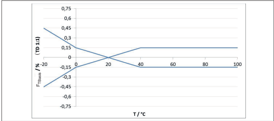
Abb. 23: Basis-Temperaturfehler F_{TBasis} bei TD 1 : 1
