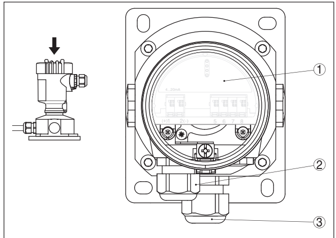
Abb. 16: Elektronik- und Anschlussraum
