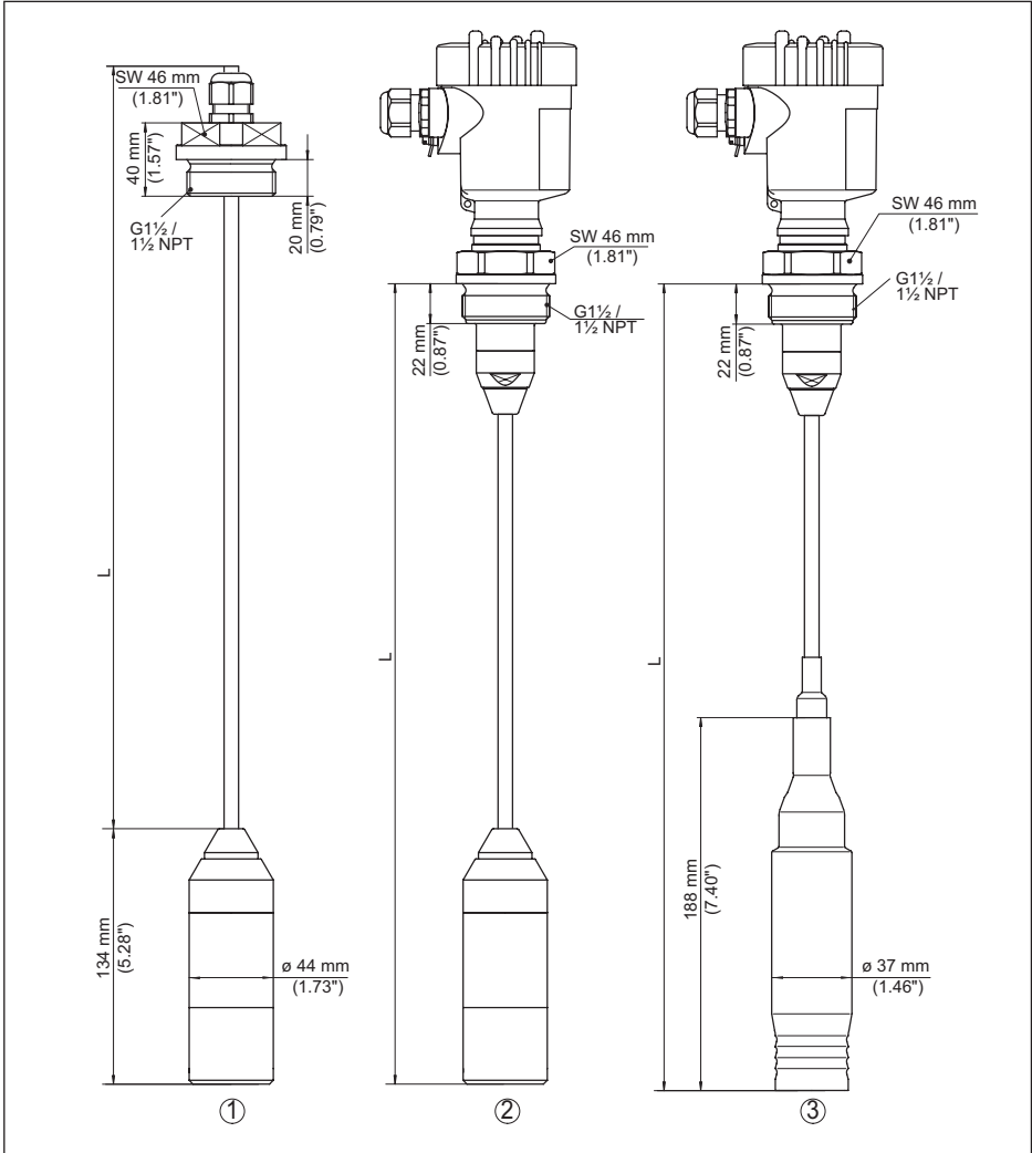
Abb. 30: VEGABAR 86, Kunststoffausführung
