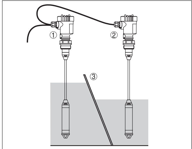
Abb. 8: Messanordnung bei der Pegeldifferenzmessung
