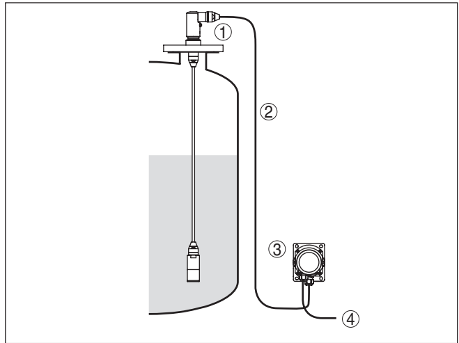
Abb. 12: Anordnung Messstelle, externes Gehäuse
