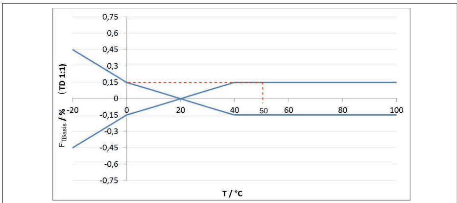
Abb. 24: Ermittlung des Basis-Temperaturfehlers für das Beispiel oben: F_{\text{TBasis}} = 0,15\%
