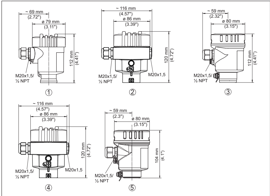
Abb. 26: Gehäuseausführungen in Schutzart IP66/IP67 und IP66/IP68 (0,2 bar), (mit eingebautem Anzeige- und Bedienmodul vergrößert sich die Gehäusehöhe um 9 mm/0.35 in bzw. 18 mm/0.71 in)
