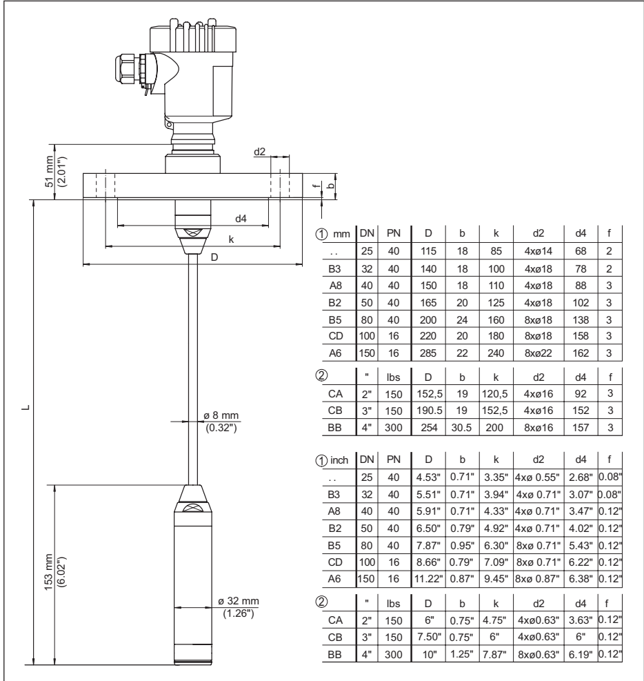
Abb. 31: VEGABAR 86, Flanschanschluss (Beispiel: Messwertnehmer 32 mm)
