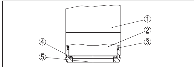
Abb. 2: Frontbündiger Einbau der keramischen Messzelle mit Doppeldichtung
