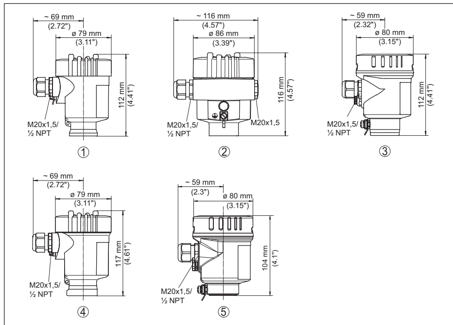
Figura 29: Differenti custodie con grado di protezione IP66/IP67 e IP66/IP68 (0,2 bar), (con tastierino di taratura con display incorporato l'altezza della custodia aumenta di 9 mm/0.35 in ovv. 18 mm/0.71 in)
