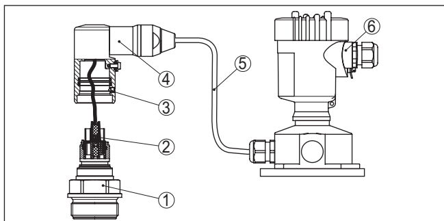
Figura 24: VEGABAR 86 in esecuzione IP68 25 bar e uscita del cavo laterale, custodia esterna
