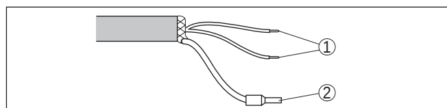
Figura 14: Assegnazione dei conduttori del cavo di connessione collegato fisso
