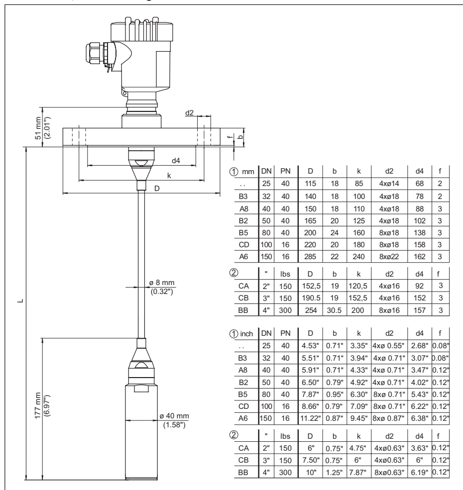
Figura 32: VEGABAR 87, attacco a flangia
