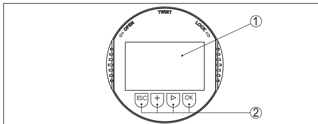
Figura 19: Elementi d'indicazione e di servizio
