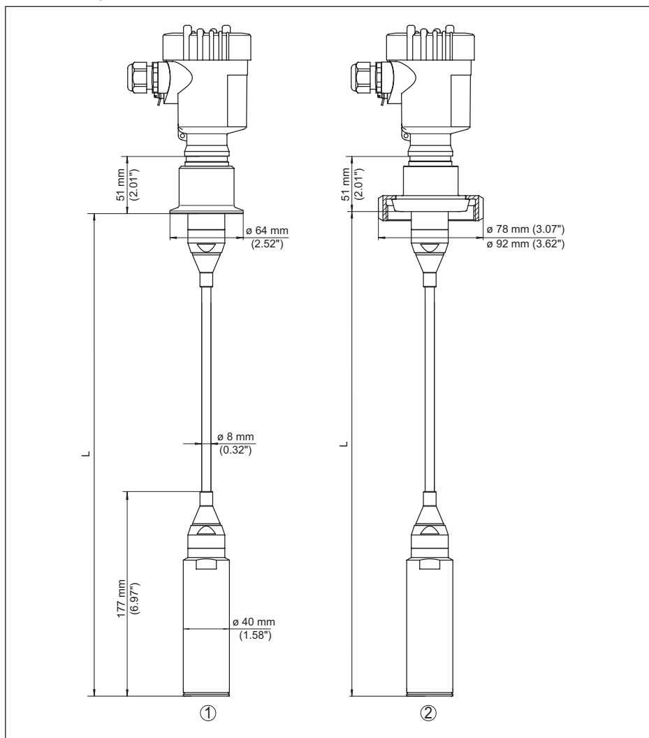
Figura 33: VEGABAR 87, attacchi igienici
