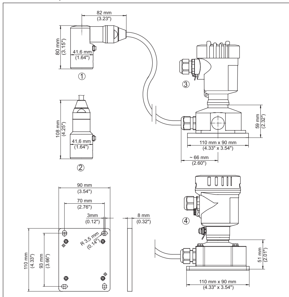
Figura 30: VEGABAR 87, esecuzione IP68 con custodia esterna
