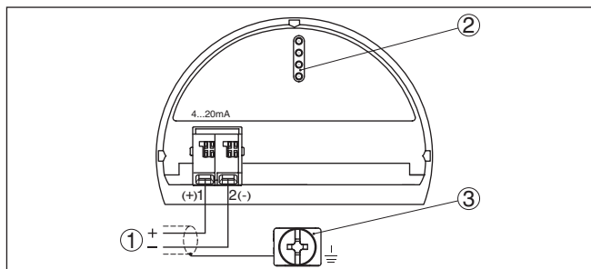
Figura 13: Vano dell'elettronica e di connessione - custodia a camera
