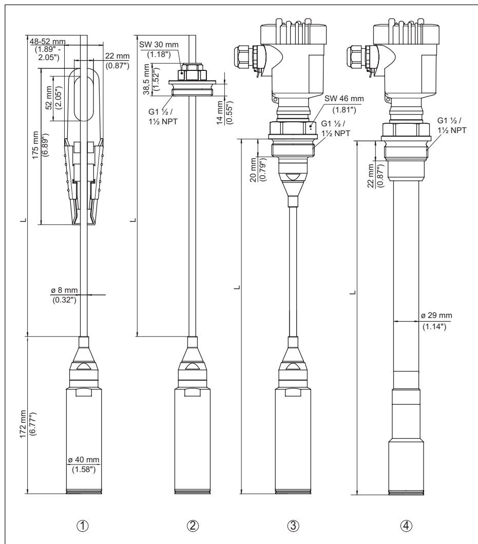
Figura 33: VEGABAR 87 - Attacchi standard
