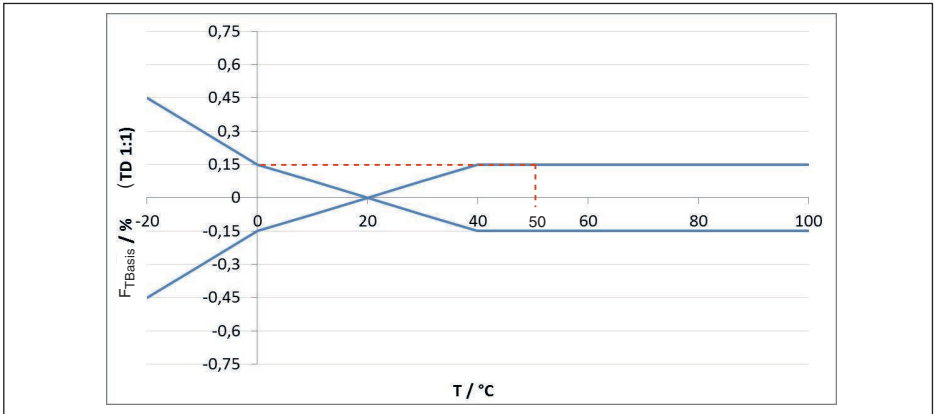
Figura 30: Calcolo dell'errore di temperatura base per il suddetto esempio: F_{TBasis} = 0,15 \%
