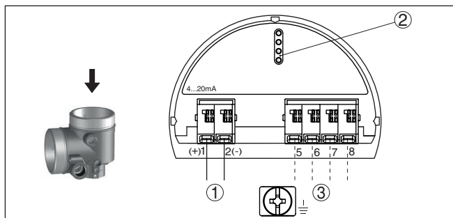
Figura 14: Vano dell'elettronica - custodia a due camere Ex-d-ia
