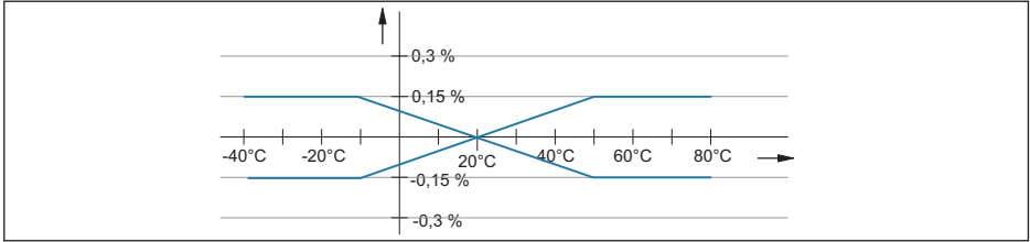
Figura 29: Variazione termica uscita in corrente
