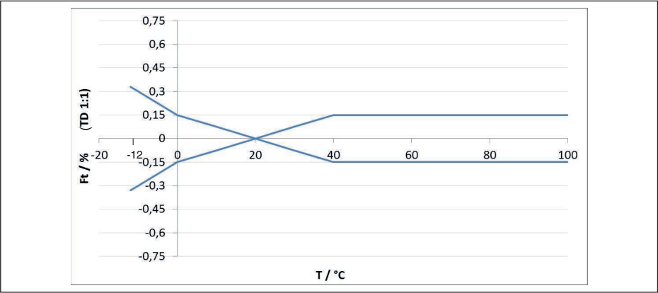
Figura 28: Errore di temperatura base F_{TBasis} con TD 1 : 1
