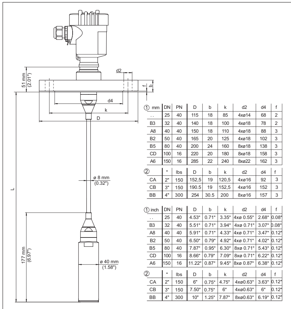
Figura 34: VEGABAR 87, attacco a flangia
