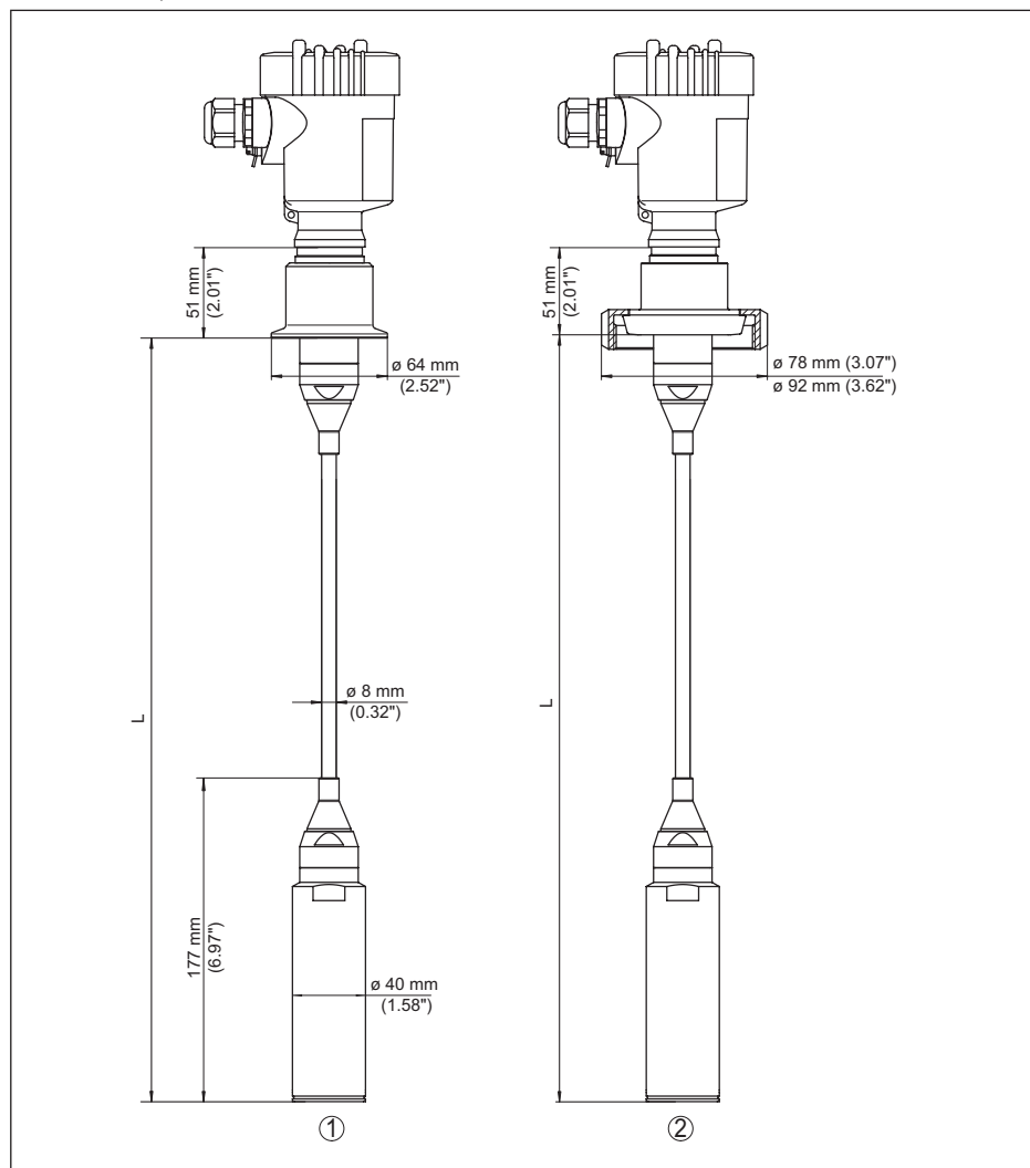
Figura 35: VEGABAR 87, attacchi igienici
