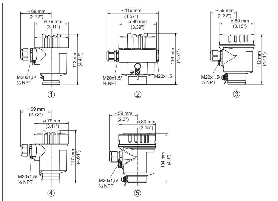
Figura 31: Differenti custodie con grado di protezione IP66/IP67 e IP66/IP68 (0,2 bar), (con tastierino di taratura con display incorporato l'altezza della custodia aumenta di 9 mm/0.35 in ovv. 18 mm/0.71 in)
