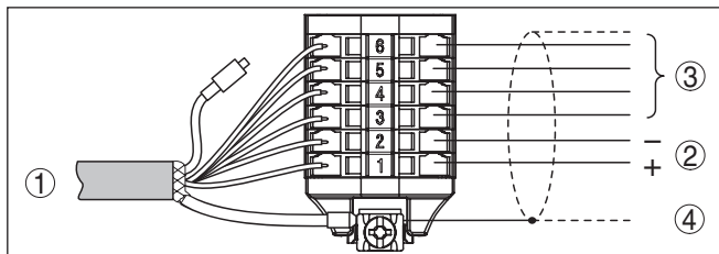
Rys. 10: Schemat przyłączy VEGABOX 03 dla VEGAWELL 52, 4 ... 20 mA/HART Pt 100
