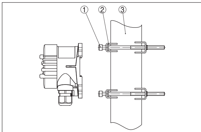
Rys. 6: VEGABOX 03 do montażu na rurze
