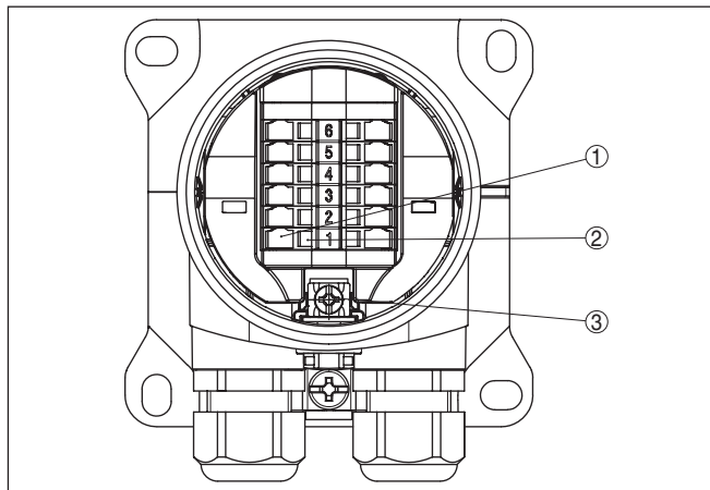
Rys. 8: Komora przyłączy VEGABOX 03
