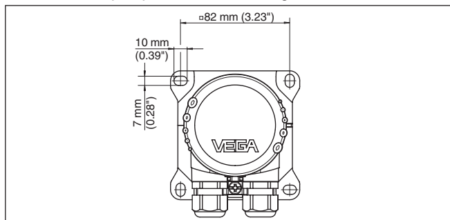
Rys. 3: Rozmieszczenie otworów przy montażu ściennym VEGABOX 03
