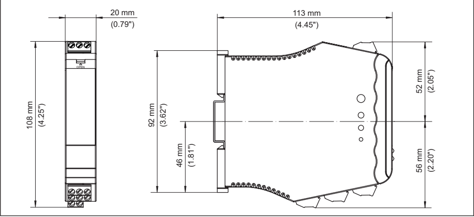
插图. 20: VEGATOR 111 的尺寸
