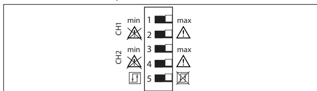
Fig. 2: Commutateur DIL VEGATOR 112
