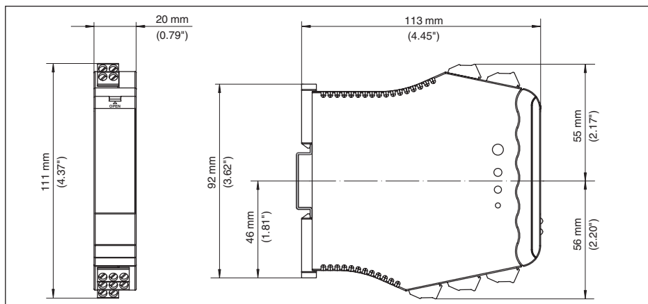
Fig. 4: Encombrement VEGATOR 112
