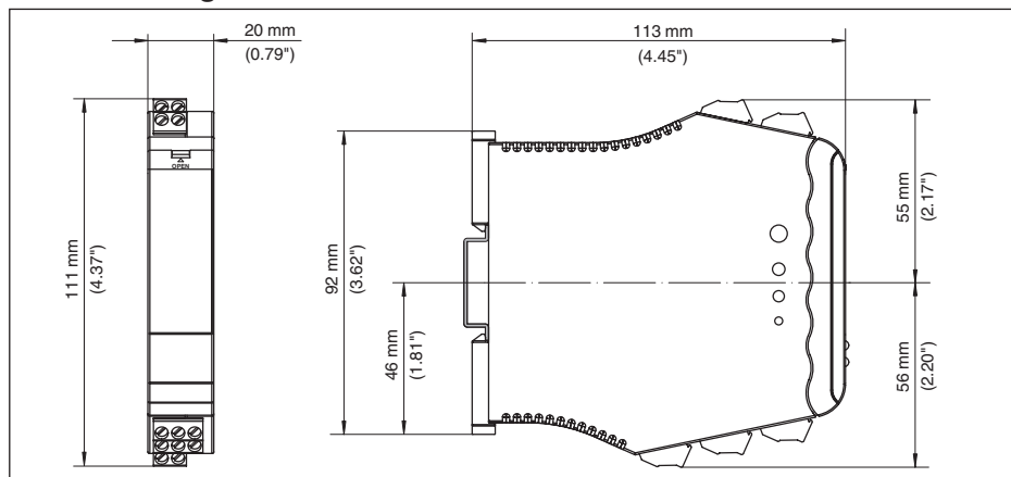
Fig. 3: Afmetingen VEGATOR 122
