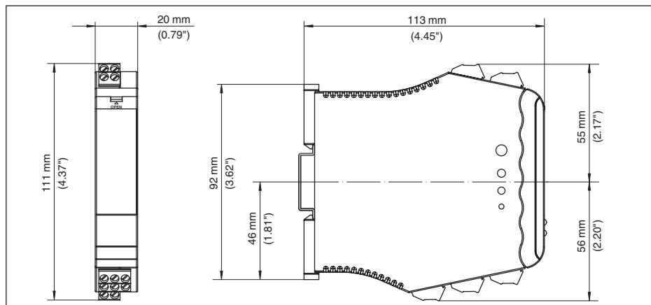
Fig. 54: Medidas VEGATOR 122
