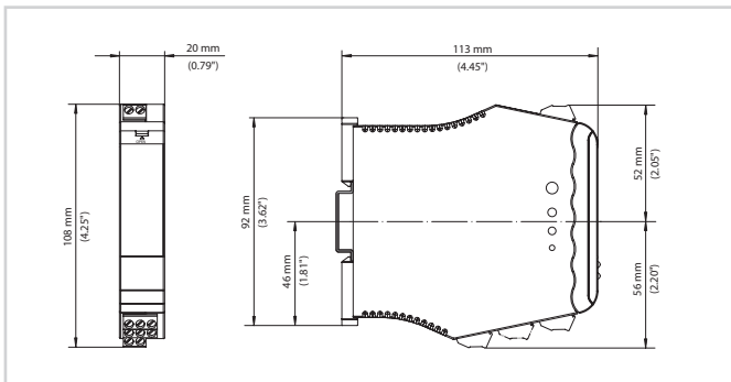
VEGATOR 111 的尺寸
