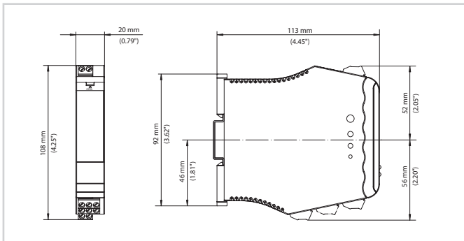
Encombrement VEGATOR 111
