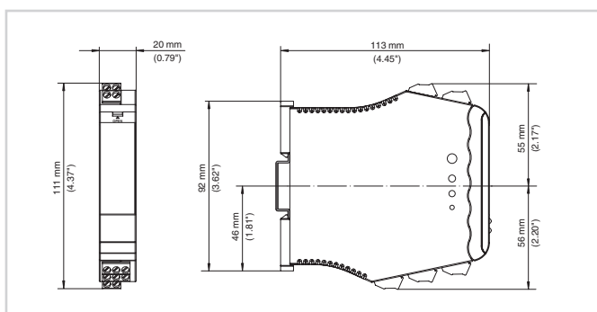
Medidas VEGATOR 112
