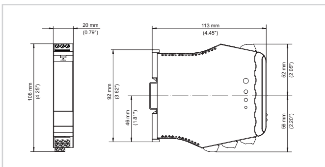
Medidas VEGATOR 121
