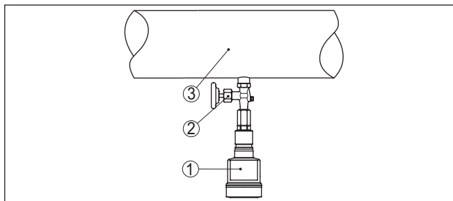
Abb. 11: Messanordnung bei der Prozessdruckmessung von Flüssigkeiten in Rohrleitungen
