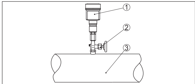
Abb. 9: Messanordnung bei Prozessdruckmessung von Gasen in Rohrleitungen
