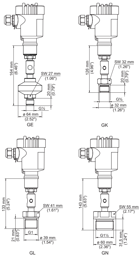
Abb. 42: VEGABAR 81, Gewindeanschluss
