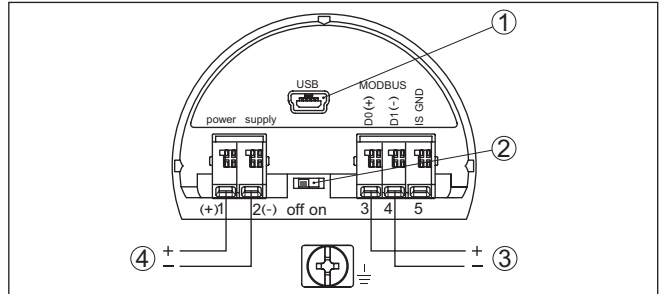
Abb. 21: Anschlussraum
