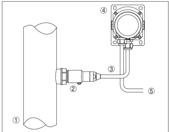
Abb. 13: Anordnung Prozessbaugruppe, externes Gehäuse
