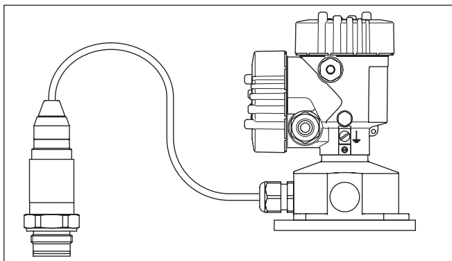
Abb. 18: VEGABAR 81 in IP68-Ausführung 25 bar mit axialem Kabelabgang, externes Gehäuse
