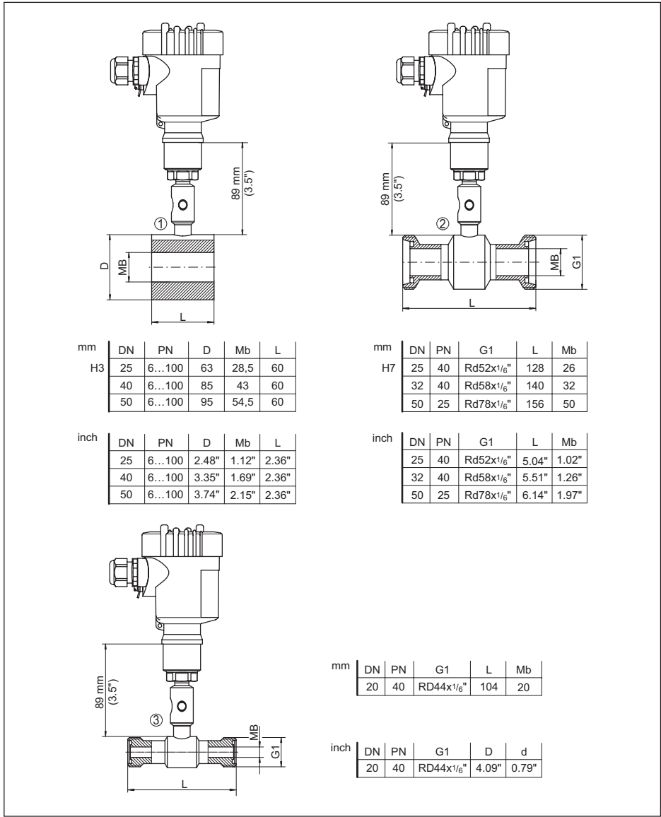
Abb. 43: VEGABAR 81, Rohrdruckmittler
