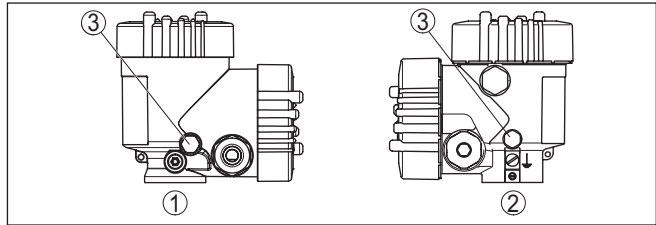
Abb. 8: Position des Filterelementes
