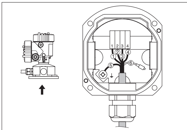
Abb. 20: Anschluss des Sensors im Gehäusesockel
