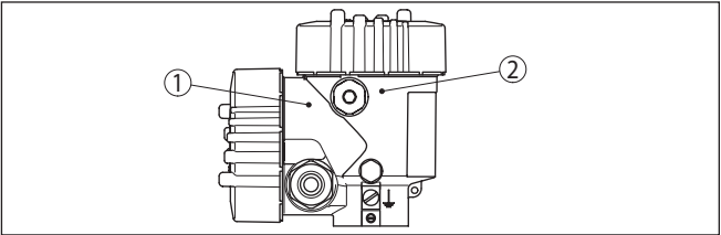
Abb. 15: Position von Anschlussraum (Modbuselektronik) und Elektronikraum (Sensorelektronik)
