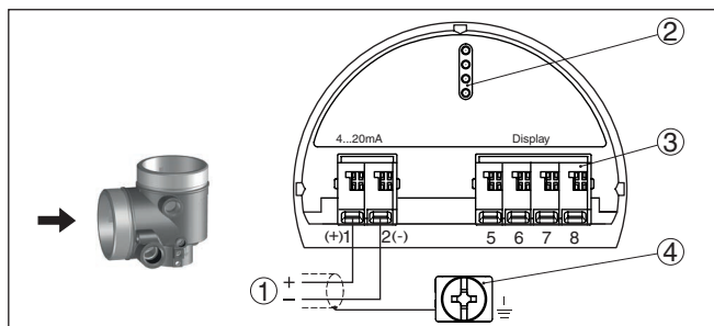
Fig. 5: Aansluitruimte - tweekamerbehuizing
