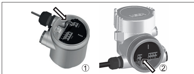
Fig. 3: Aansluitstappen 5 en 6
