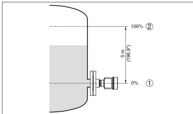
Fig. 9: Parametreervoorbeeld min.-/max.-inregeling niveaumeting
