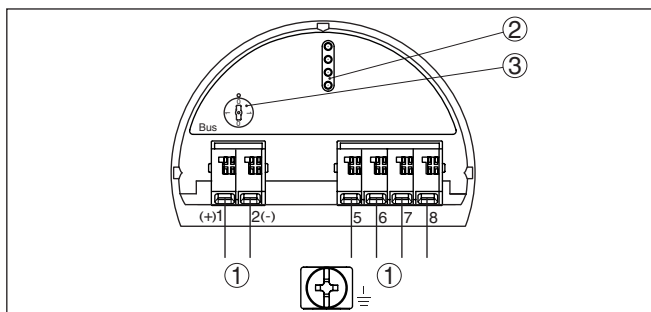
Figura 5: Vano dell'elettronica - custodia a due camere
