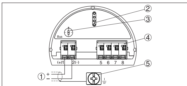
Fig. 4: Elektronica- en aansluitruimte - eenkamerbehuizing
