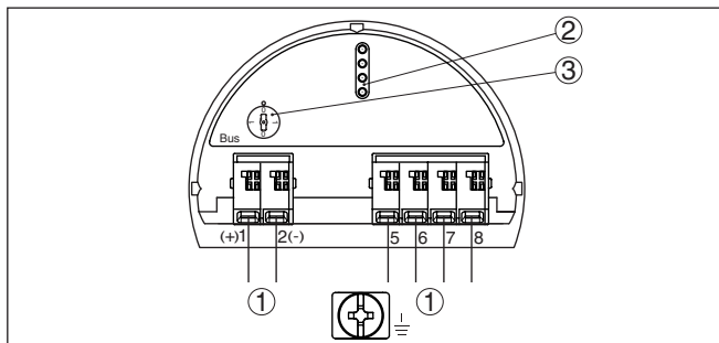
Fig. 5: Elektronicaruimte - tweekamerbehuizing
