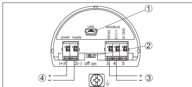
Figura 5: Vano di connessione
