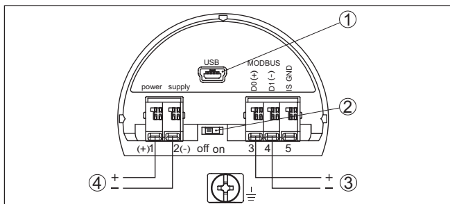
Fig. 5: Aansluitruimte
