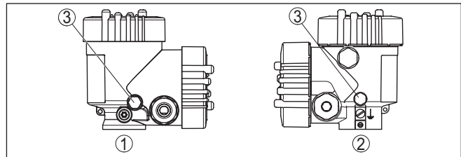
Abb. 2: Position des Filterelementes
