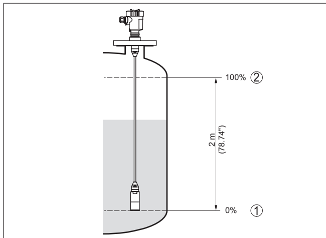
Figura 6: Esempio di parametrizzazione taratura di min./max. per misura di livello
