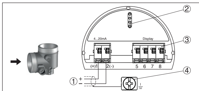
Abb. 5: Anschlussraum - Zweikammergehäuse
