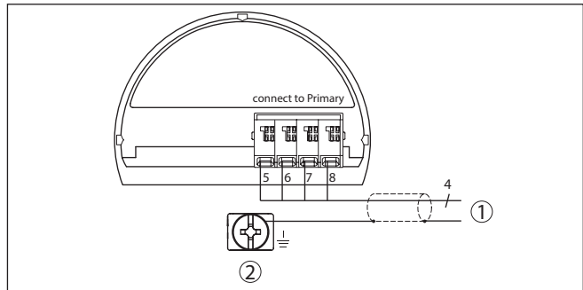
Fig. 3: Esquema de conexiones VEGABAR 82 dispositivo secundario
