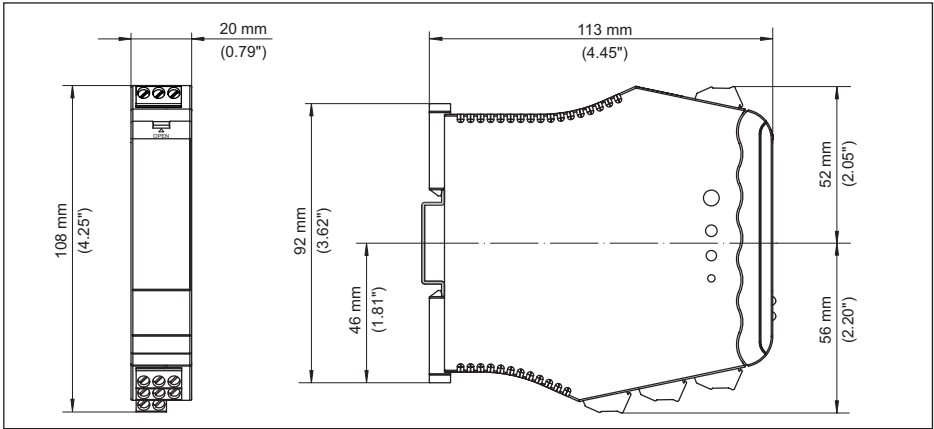
Figura 9: Dimensioni VEGATOR 141
