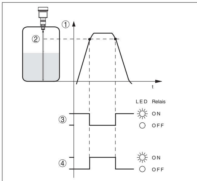
Figura 8: Diagramma funzionale controllo a un punto
