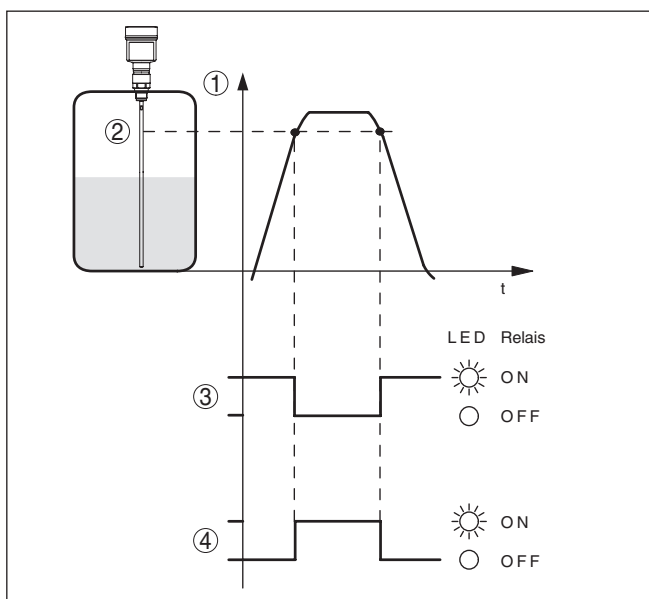
Fig. 8: Functiediagram eenpuntsregeling
