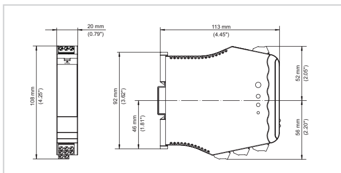
VEGATOR 142 的尺寸
