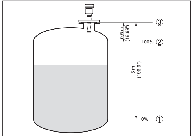
Abb. 8: Parametrierbeispiel Min.-/Max.-Abgleich
